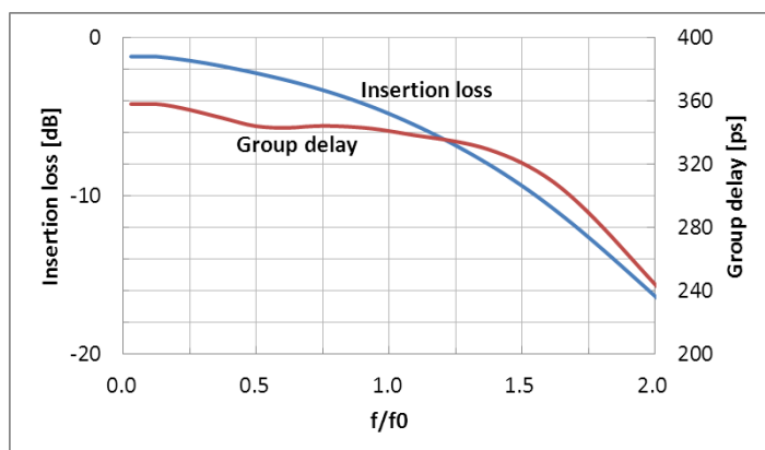
伝送特性
