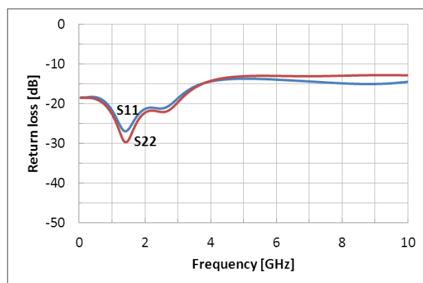
反射特性
