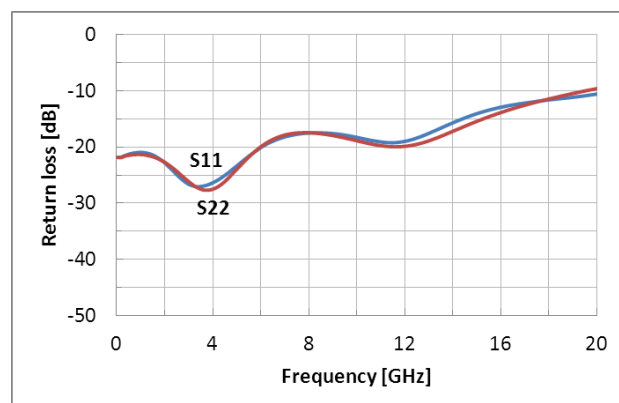
反射特性
