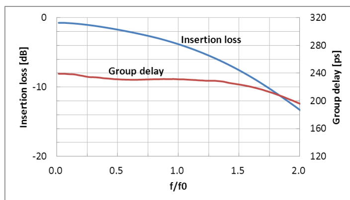
伝送特性
