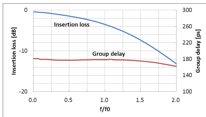
伝送特性
