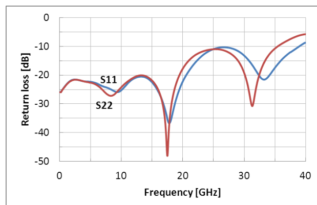
反射特性
