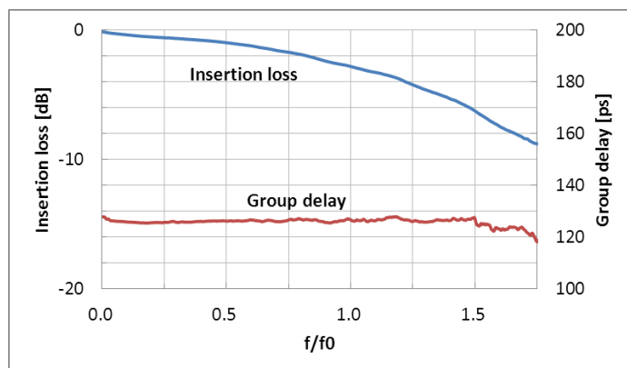
伝送特性
