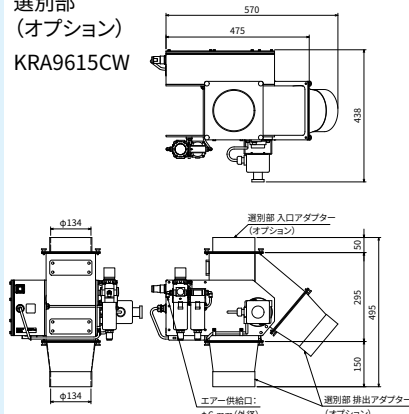
選別部 (オプション) KRA9620CW
