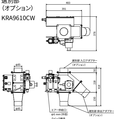
選別部 (オプション) KRA9615CW
