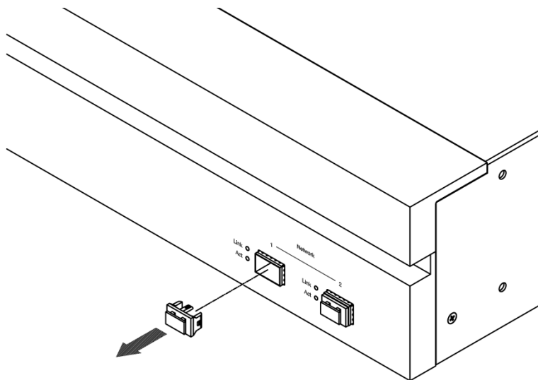
図 2.5.2.1-1 SFP ケージプラグの取り外し
