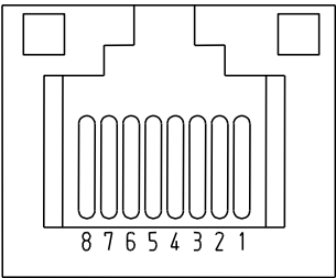
* 嵌合面から見た図
