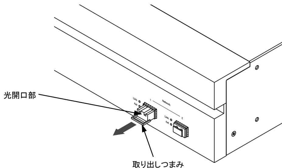
図 2.5.2.2-1 SFP モジュールの取り外し
