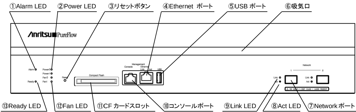
図 1.3-1 装置正面図と各部の名称
