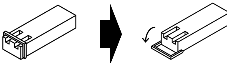
図 2.5.2.2-2 SFP モジュール取り出しつまみの操作
