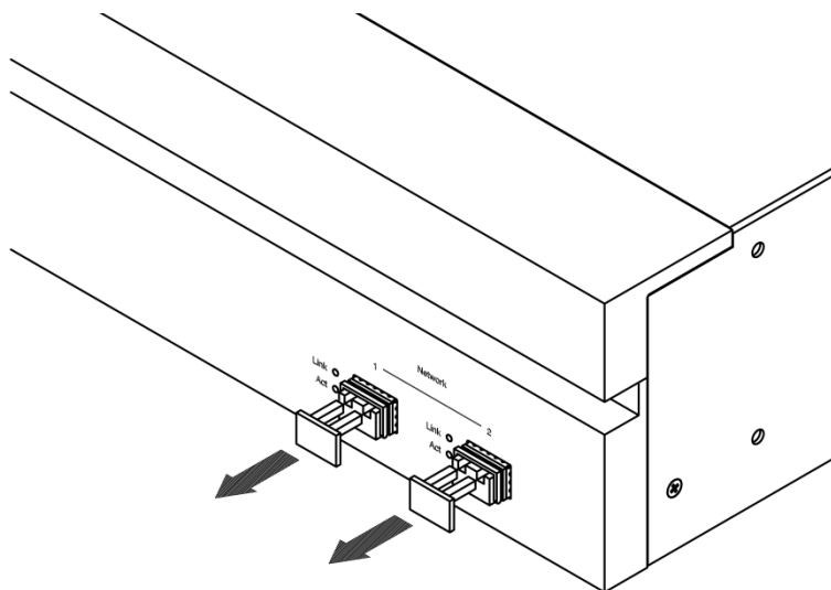
図 2.5.3.1-1 防塵プラグの取り外し
