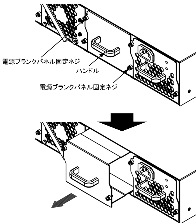
図 4.3.1-1 電源ブラנקパネルの取り外し
