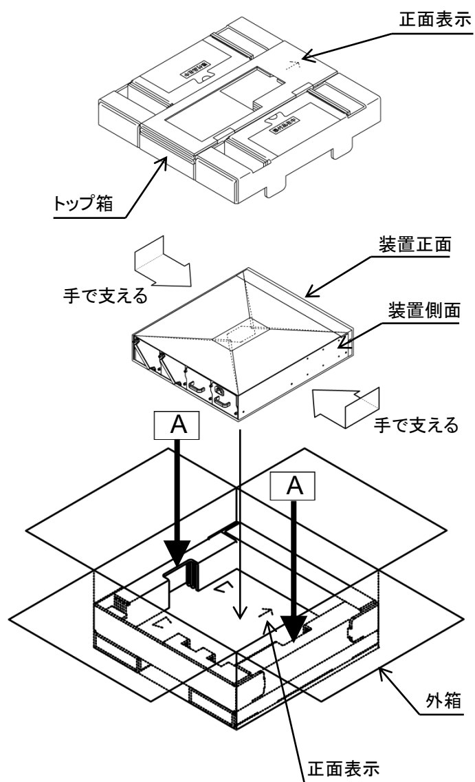
図 2.10.1-1 梱包方法
