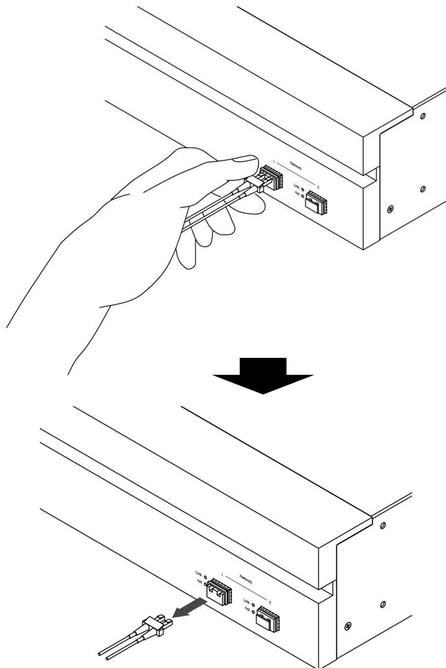
図 2.5.3.2-1 光ファイバケーブルの取り外し
