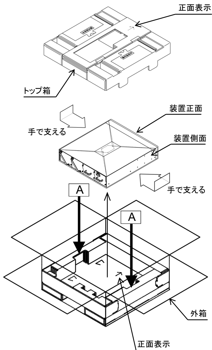
図 2.1.1-1 開梱方法
