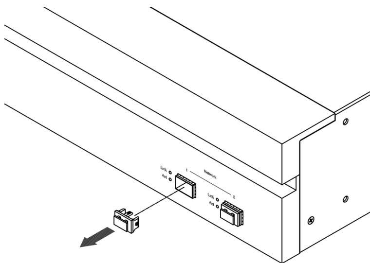
図 2.5.2.1-1 SFP ケージプラグの取り外し
