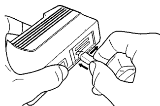
図 2.5.1.2-2 フェルールクリーナの使用例(2)
