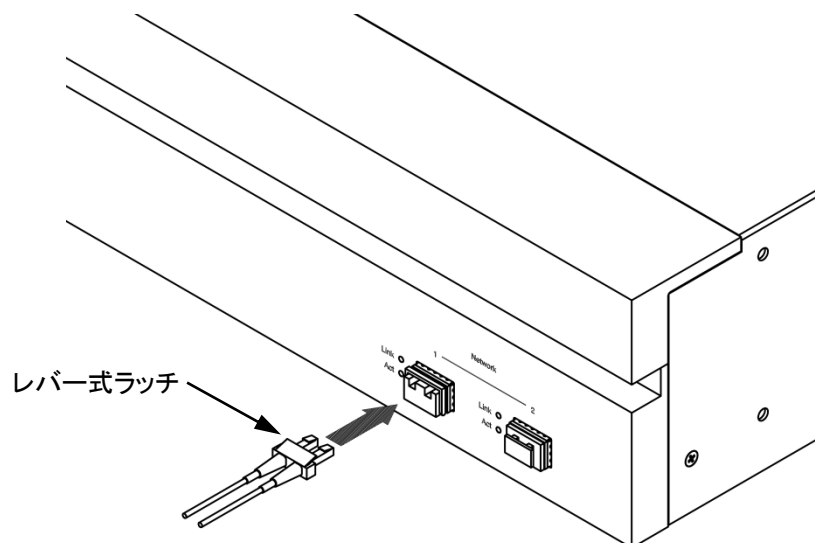
図 2.5.3.1-3 光ファイバケーブルの差し込み
