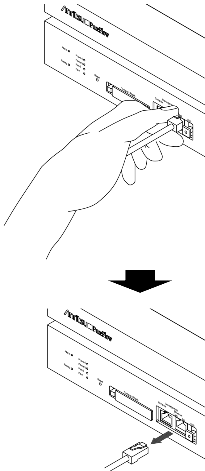
図 2.6.2-1 UTP ケーブルの取り外し
