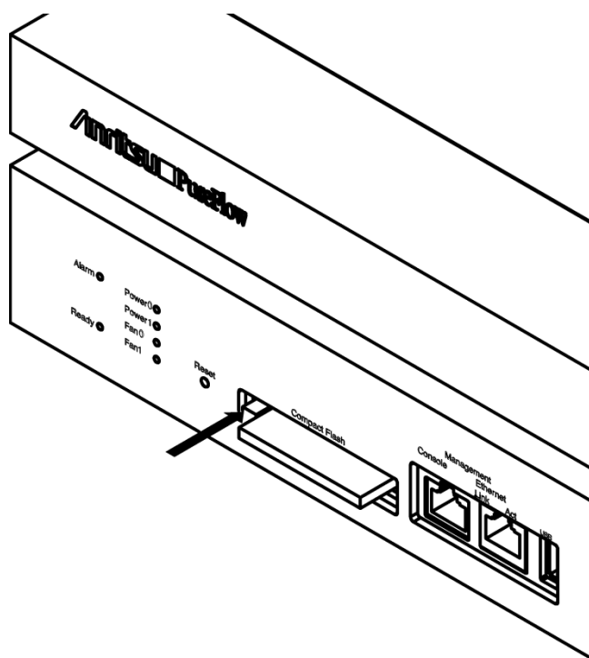
図 2.7-3 CF カードの取り出し
