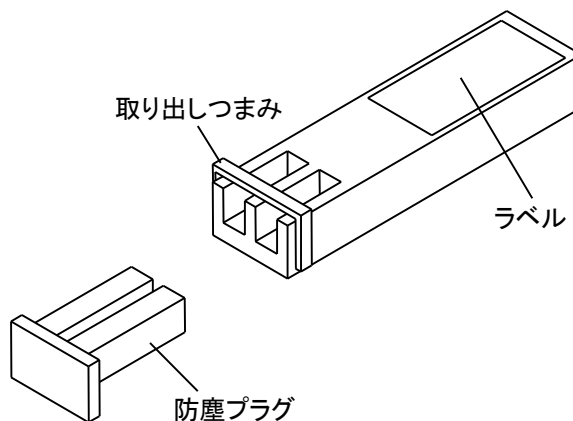
図 2.5-1 SFP モジュール外観 (LC コネクタの場合)
