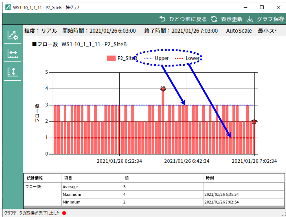
図 4.10.2-4 フロー数, 棒グラフでの上限値・下限値の描写
