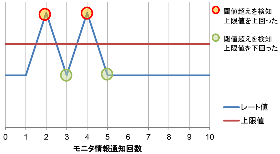
図 4.10.1-1 連続検知回数 1 回の場合の閾値超過検知タイミング
