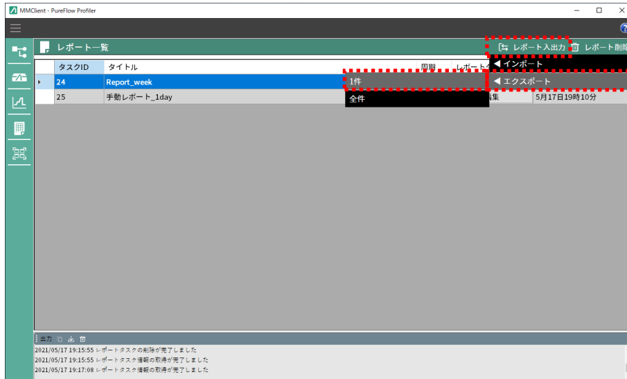
図 5.5.1-3 エクスポート－1 件の選択
