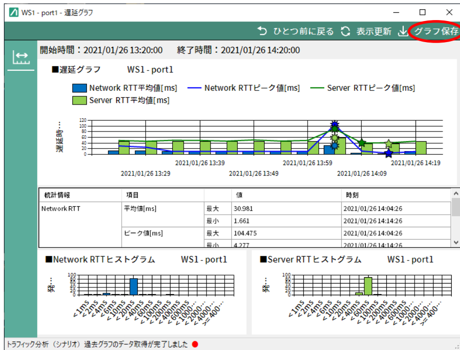
図 4.5.5-3 グラフ保存(トラフィック分析グラフ:遅延)
