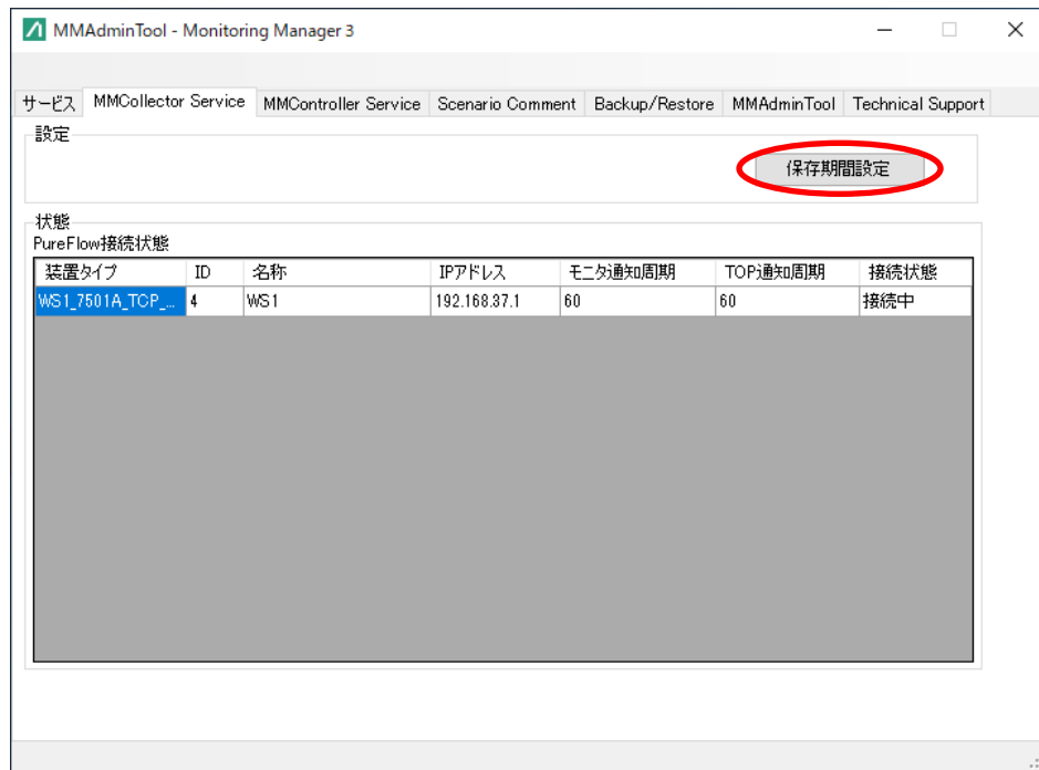
図 7.4.1-1 MMCollector Service 管理
