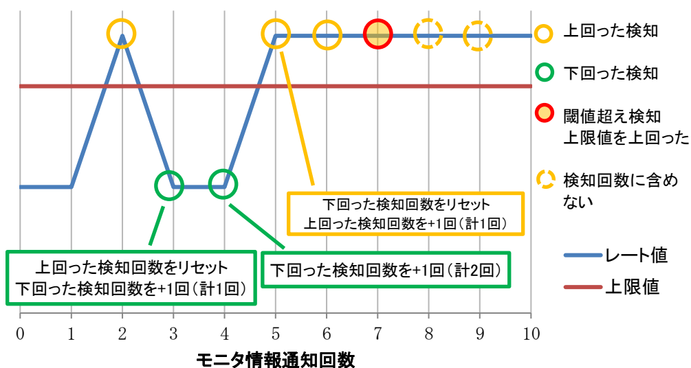
図 4.10.1-2 閾値超え検知タイミング(上限値を上回った)
