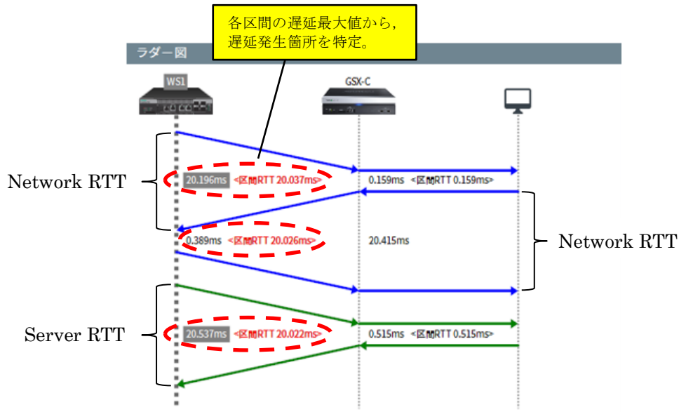
図 4.7.14-2 ラダー図
