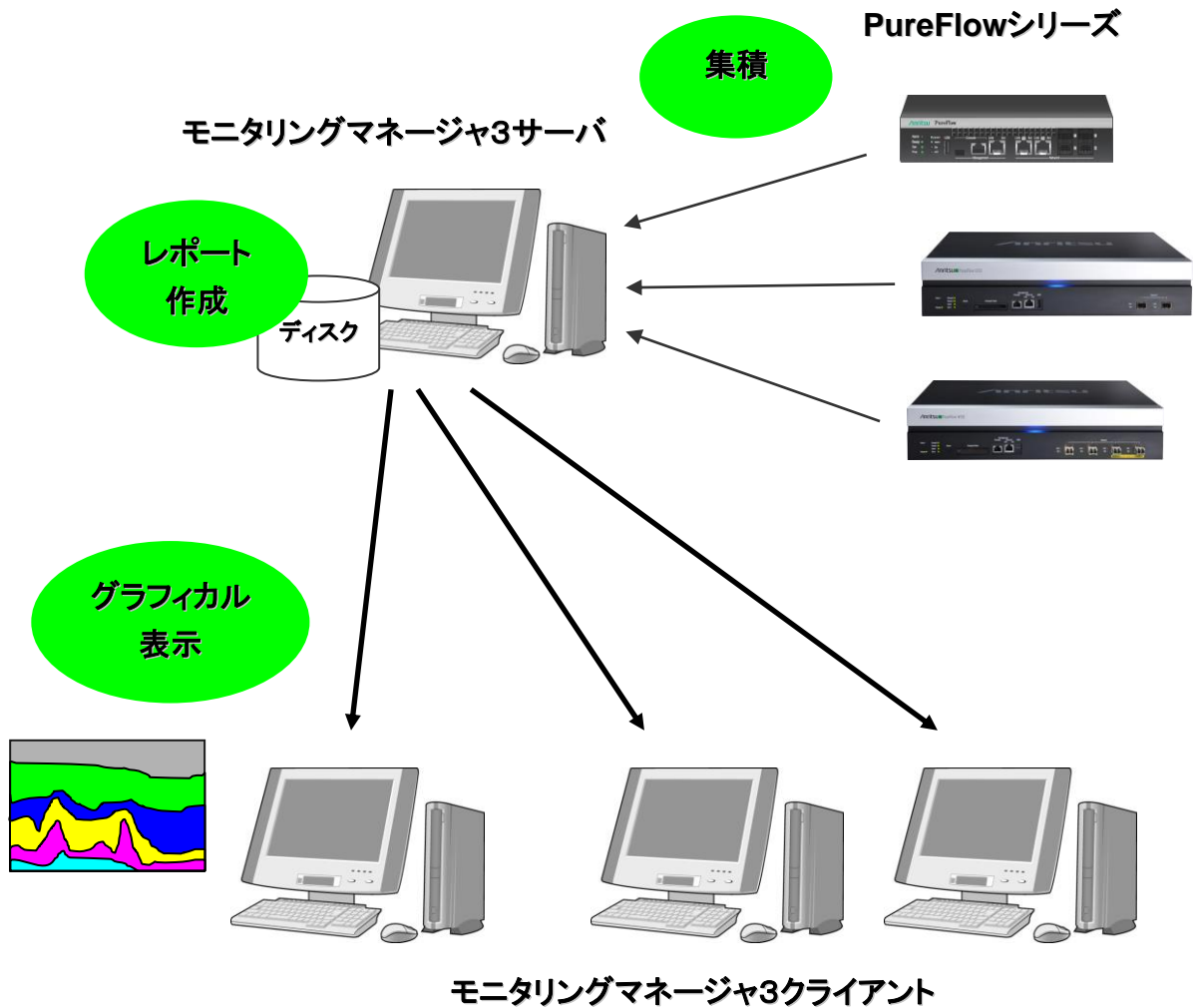
図 1.1-1 システム構成図
