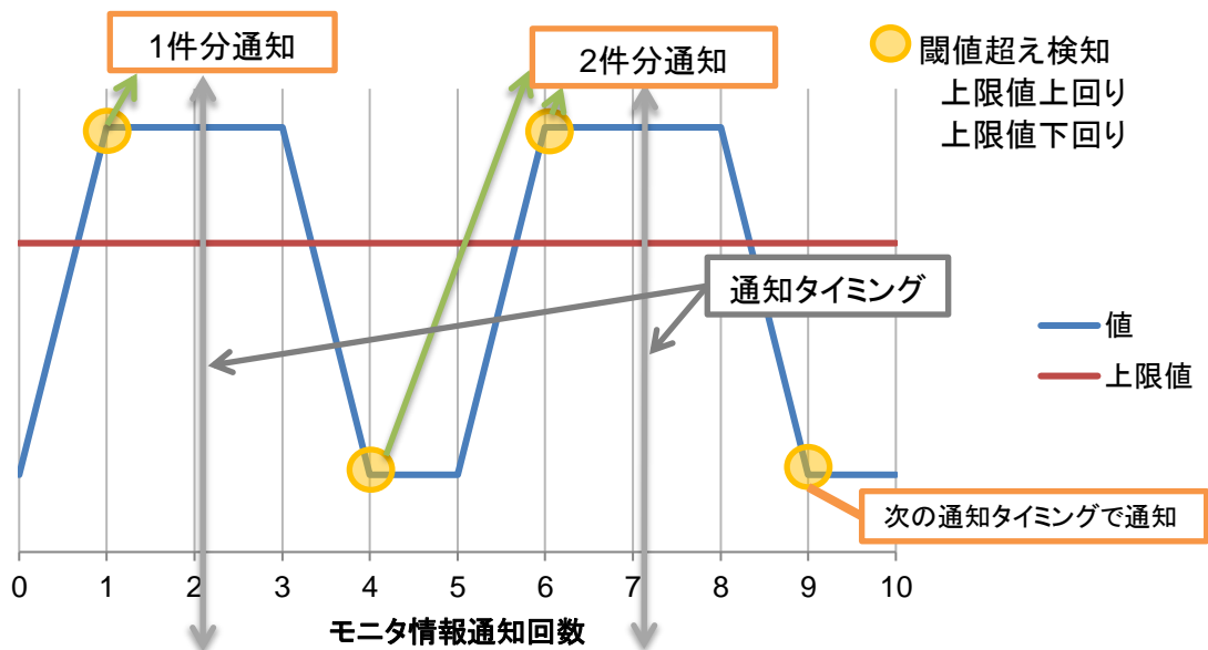
図 4.10.1-5 モニタ情報通知周期 60 秒、閾値検知回数 1 回、閾値超え通知周期 5 分の場合
