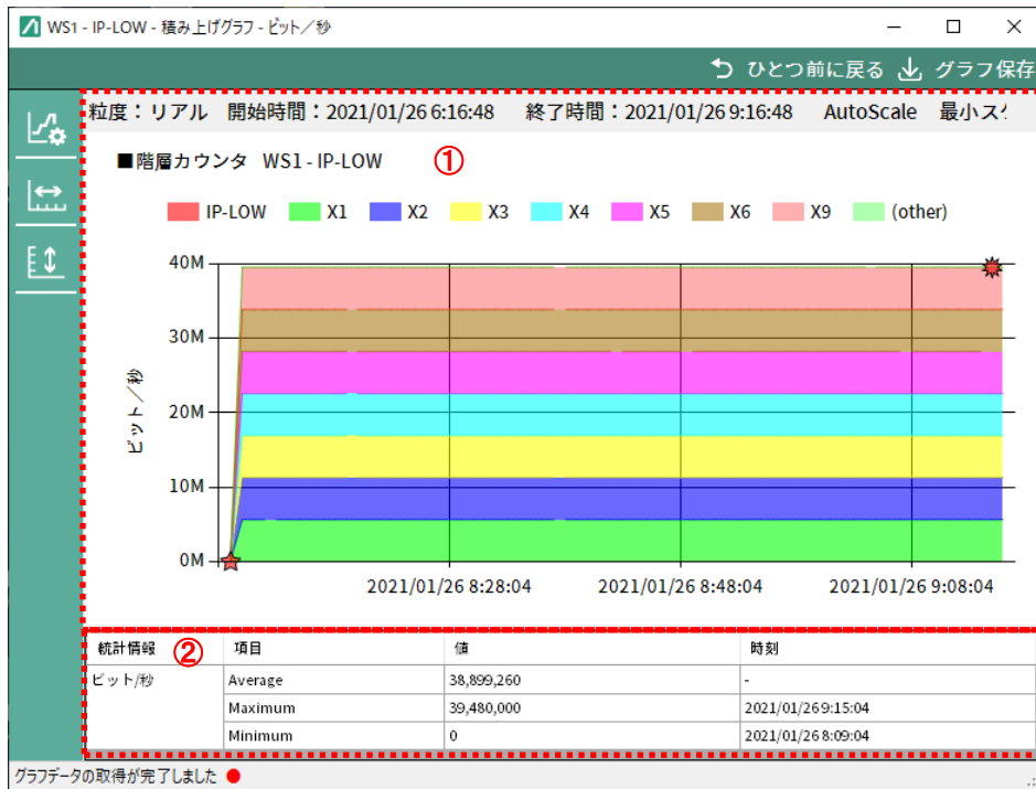
図 4.7.1-1 階層カウンタ 積み上げグラフ
