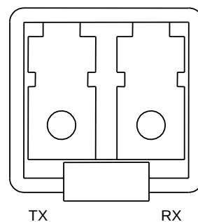
図 A.8-1 1000BASE-LX モジュール正面図
