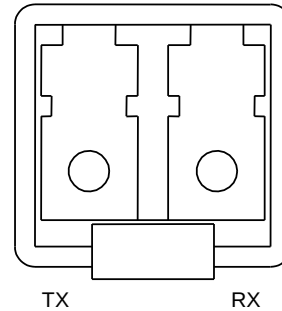
図 A.7-1 1000BASE-SX モジュール正面図
