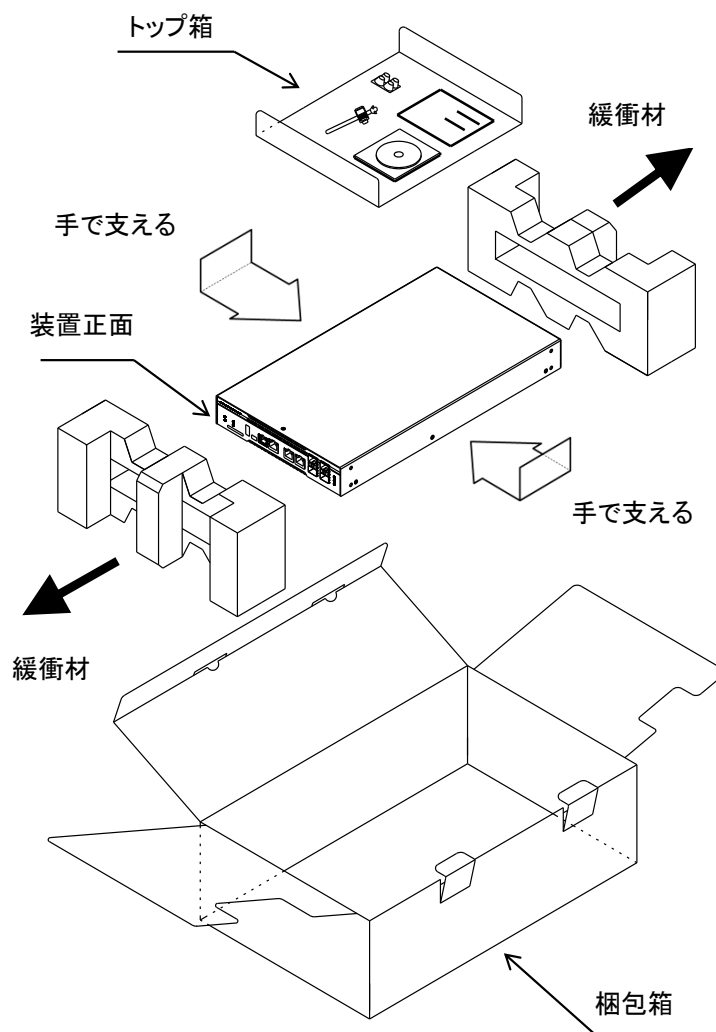
図 2.1.1-1 開梱方法
