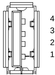
図 A.5-1 USB コネクタ正面図
