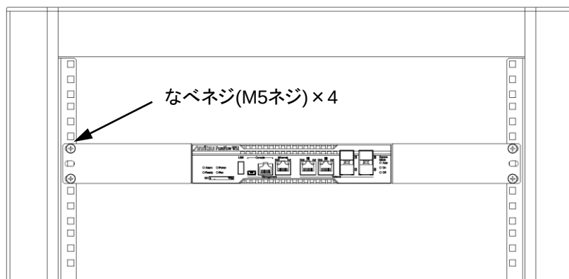
図 2.4.2.1-4 19 インチラックへの装置搭載 (EIA, IEC 規格)
