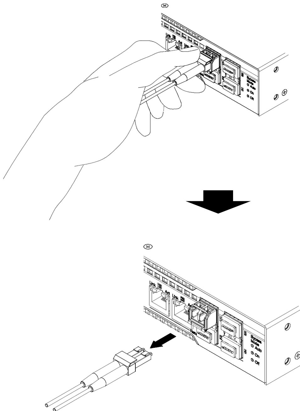
図 2.7.2-1 光ファイバケーブルの取り外し
