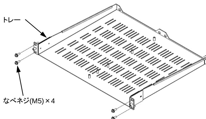
図 2.4.2.2-1 トレーの取り付け
