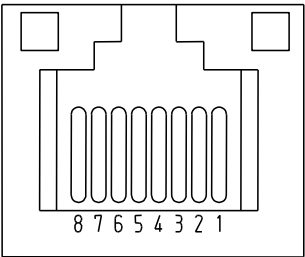
図 A.4-1 ピン配置
