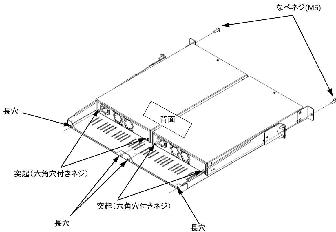
図 2.4.2.2-3 トレーへの装置搭載
