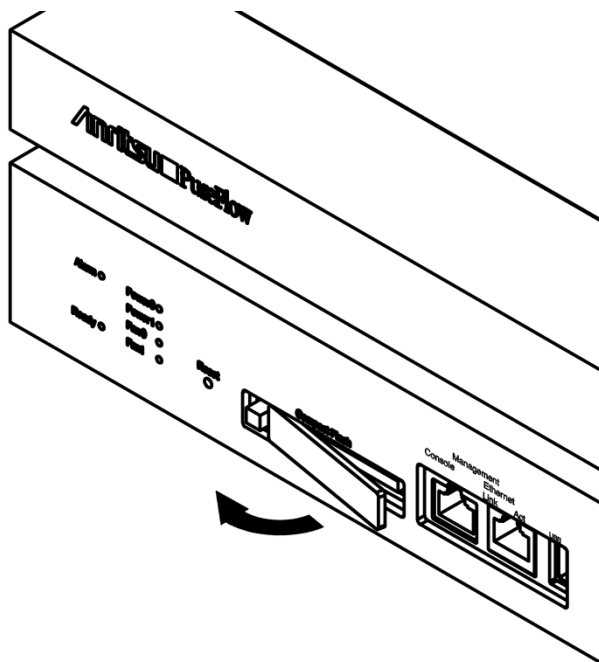
図 2.9-1 CF キャップの取り外し
