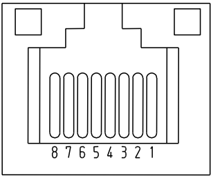
図 A.2-1 ピン配置
