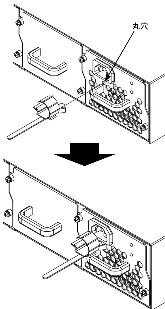
図 3.1-3 AC 電源コードクランプの取り付け
