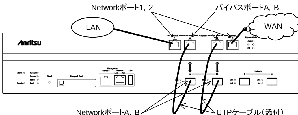
図 2.5.2-3 装置の正面図 (NF7605A)
