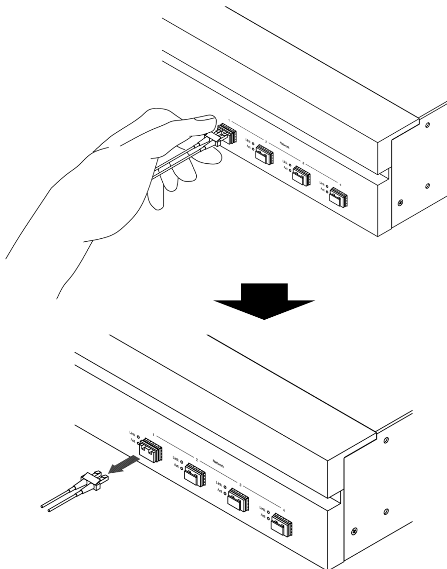
図 2.7.2-1 光ファイバケーブルの取り外し
