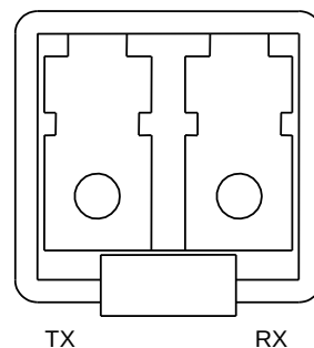
図 A.7-1 1000BASE-LX モジュール正面図
