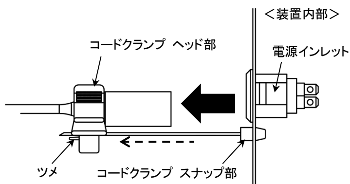
図 3.4-2 AC 電源コードクランプの取り外し
