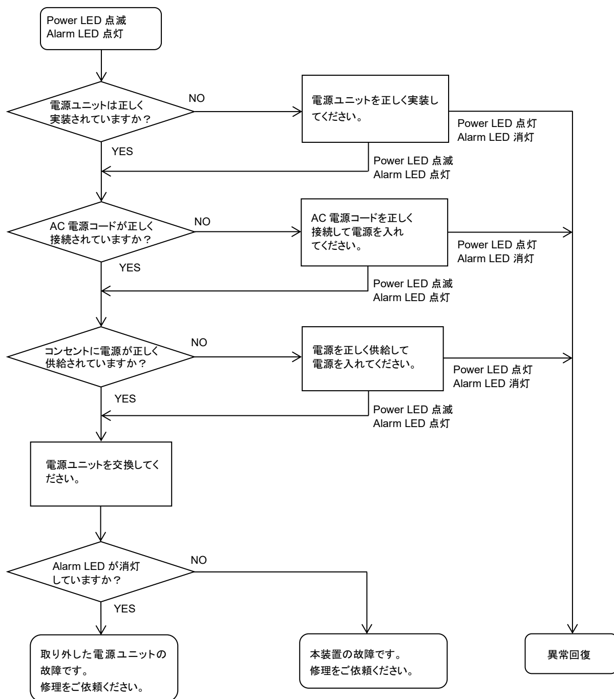
図 5.2.1-1 Power LED 点滅時異常探求フロー
