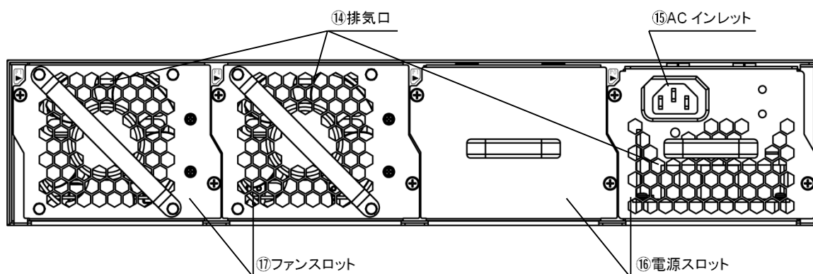
図 1.3-2 装置背面図と各部の名称
