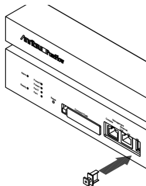
図 2.10-4 USBキャップの取り付け
