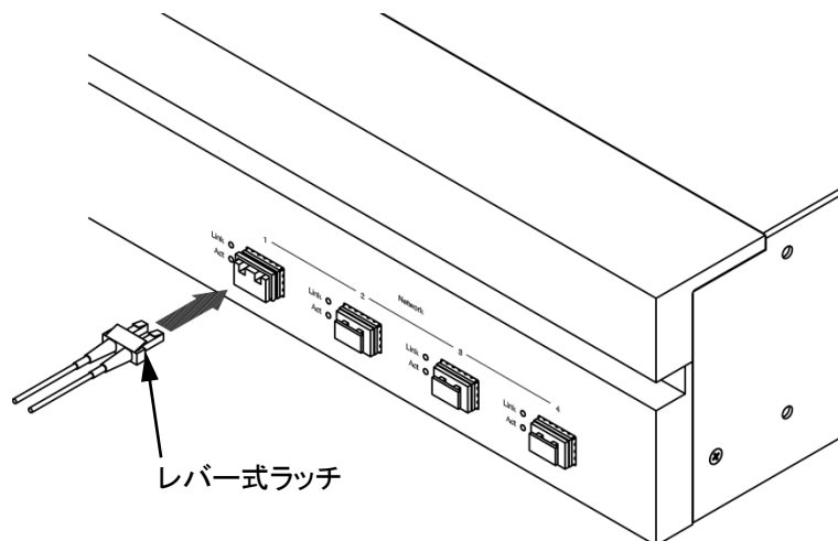
図 2.7.1-3 光ファイバケーブルの差し込み
