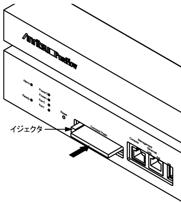
図 2.9-2 CF カードの挿入
