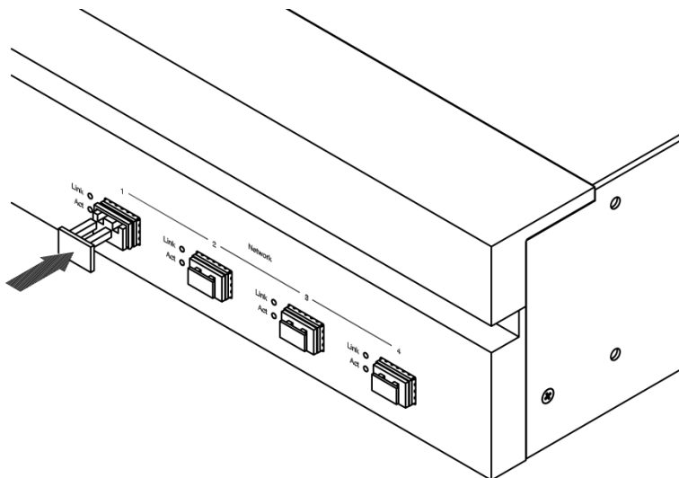
図 2.7.2-2 防塵プラグの取り付け
