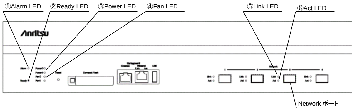
図 5.1-1 LED の名称
