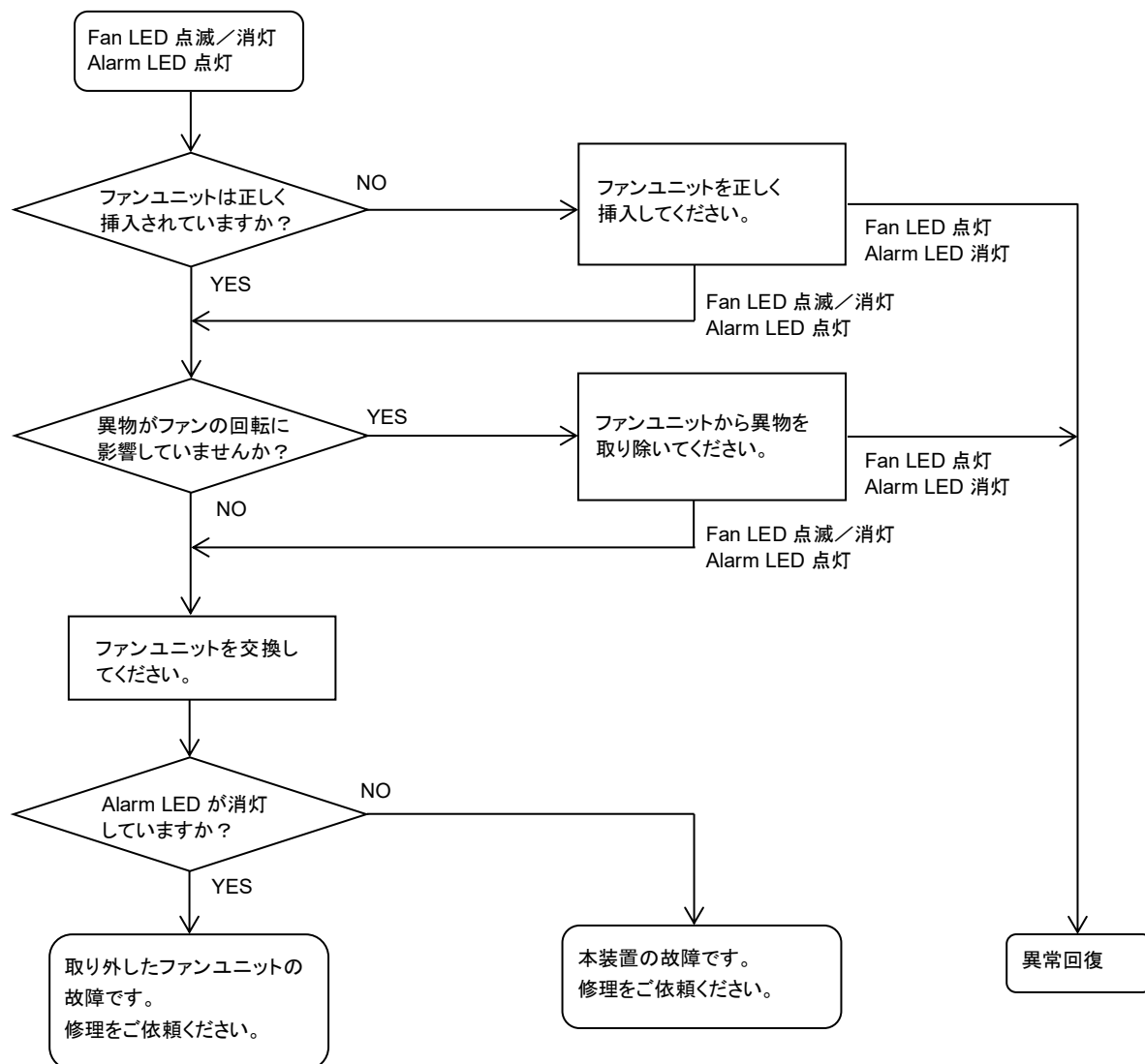
図 5.2.2-1 Fan LED 点滅時異常探求フロー
