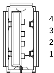
図 A.3-1 USB コネクタ正面図
