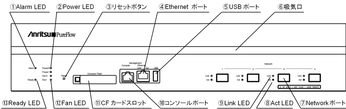
図 1.3-1 装置正面図と各部の名称
