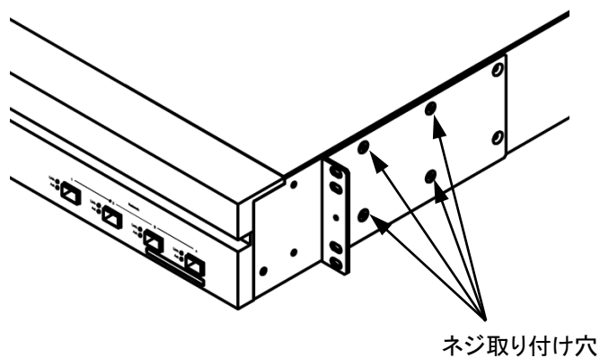
図 2.4.2-4 取り付け穴の位置(前方位置)
