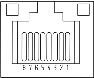
図 A.2-1 ピン配置
