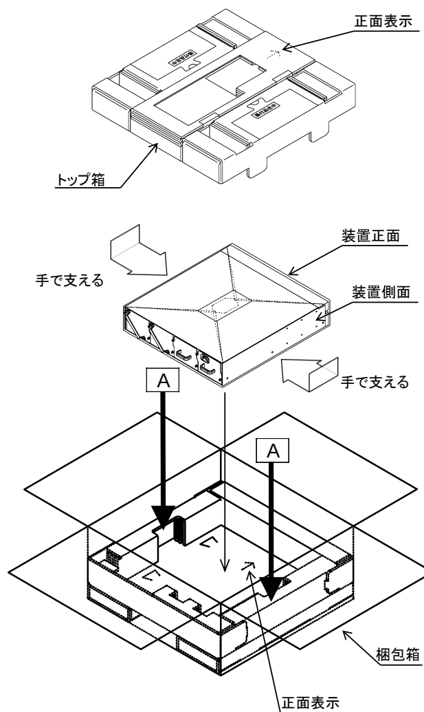
図 2.12.1-1 梱包方法
