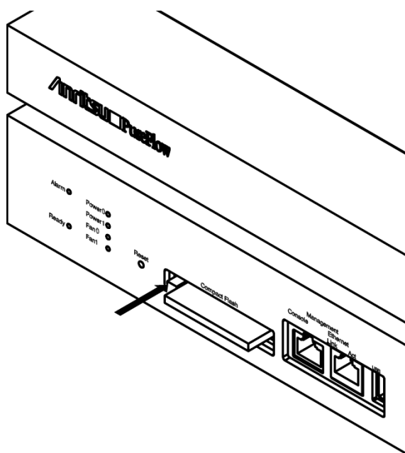
図 2.9-3 CF カードの取り出し
