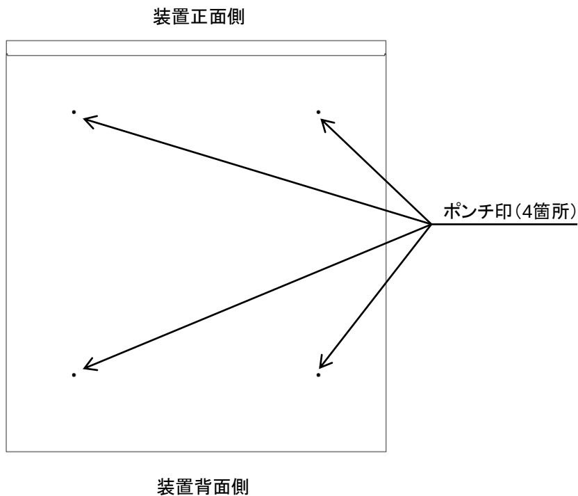
図 2.4.1-1 ゴム足用ポンチ印
