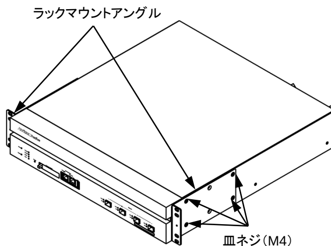
図 2.4.2-1 ラックマウントアングルの取り付け
