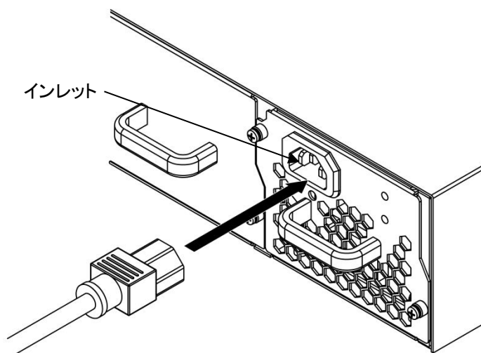
図 3.1-1 AC 電源コードの接続(インレット)
