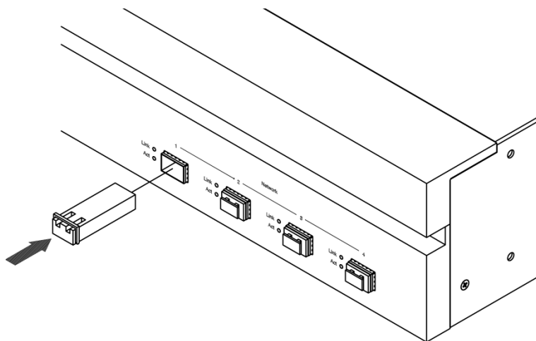
図 2.6.2.1-2 SFP モジュール挿入
