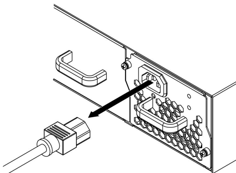
図 3.4-3 AC 電源の切断(インレット)
