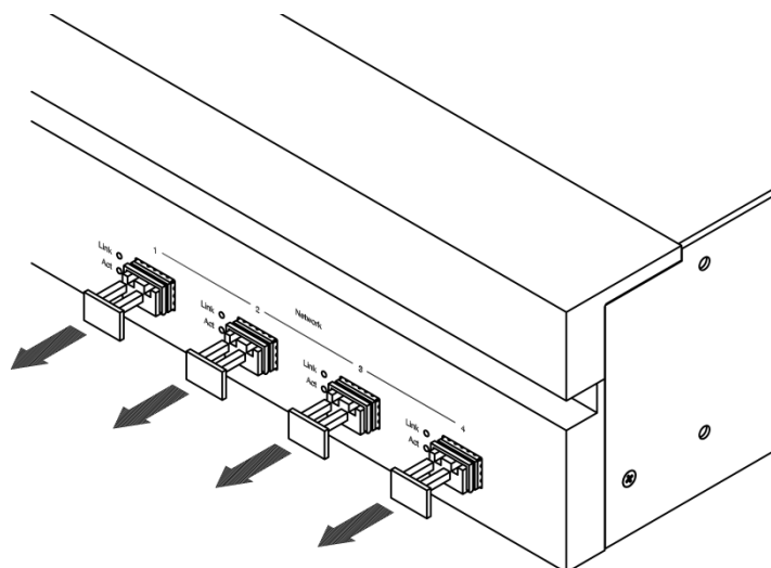
図 2.7.1-1 防塵プラグの取り外し
