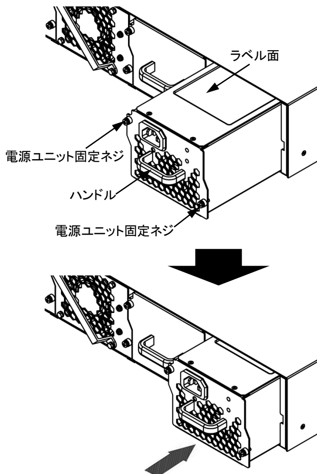
図 4.2.2-1 電源ユニットの取り付け
