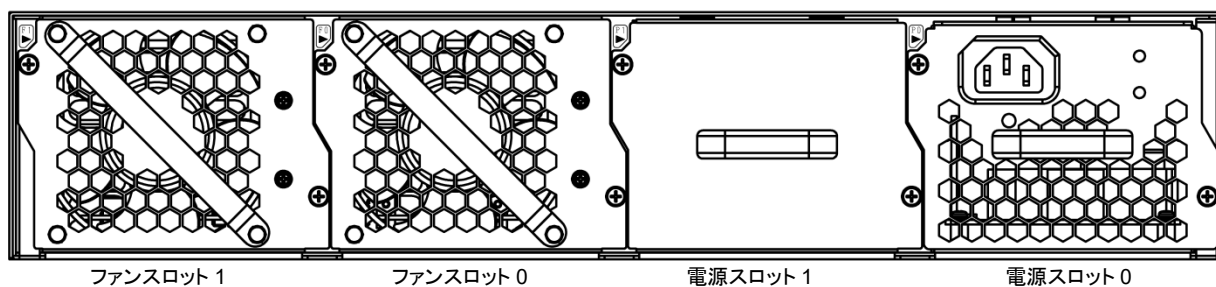
図 1.1-4 装置の背面図
