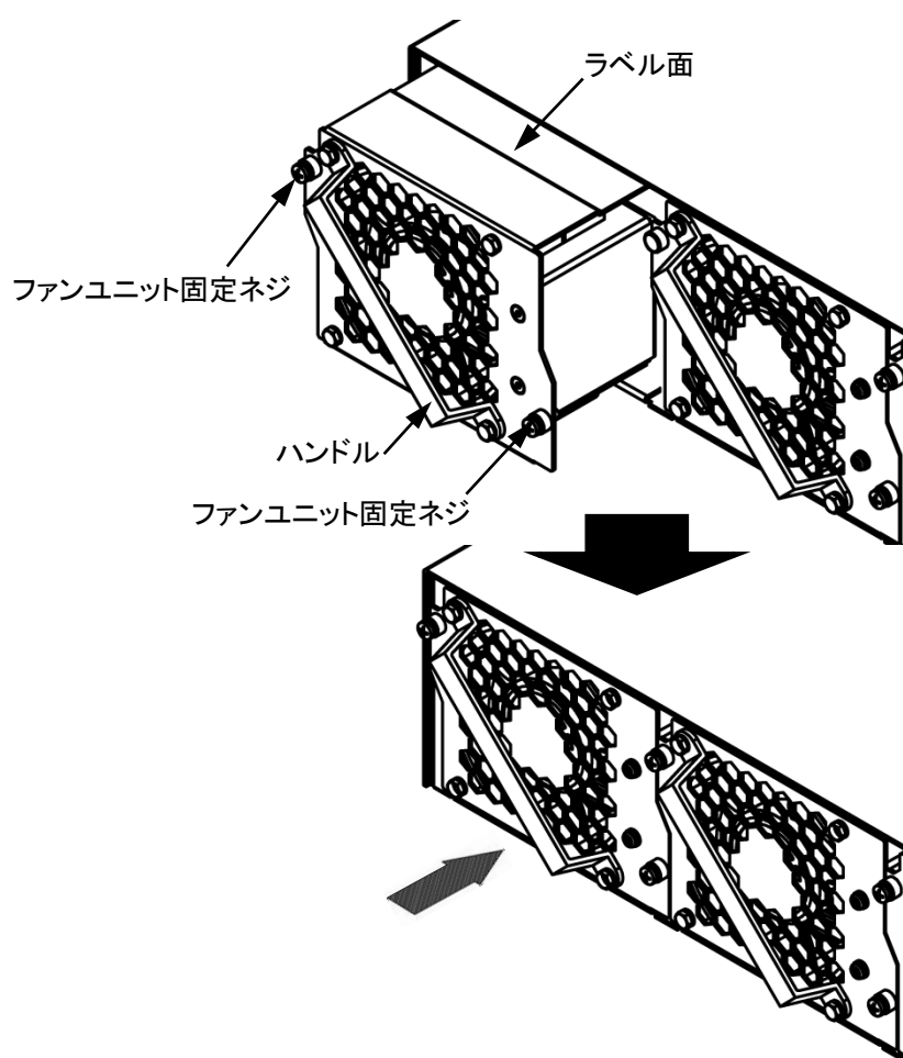
図 4.1.2-1 ファンユニットの取り付け
