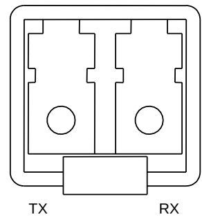
図 A.4-1 10GBASE-SR モジュール正面図
