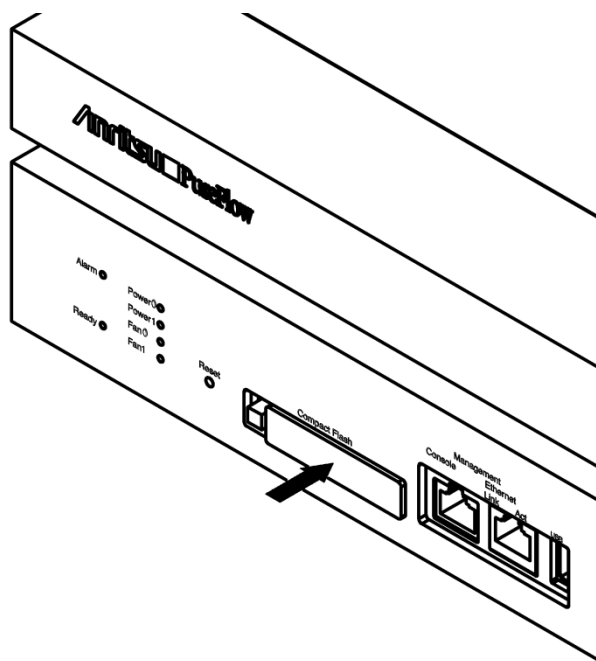
図 2.9-4 CF キャップの取り付け
