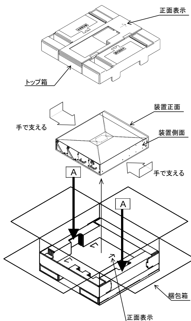
図 2.1.1-1 開梱方法
