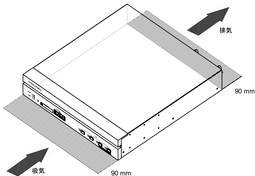
図 2.3-1 空きスペース
