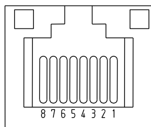
図 A.8-1 ピン配置
