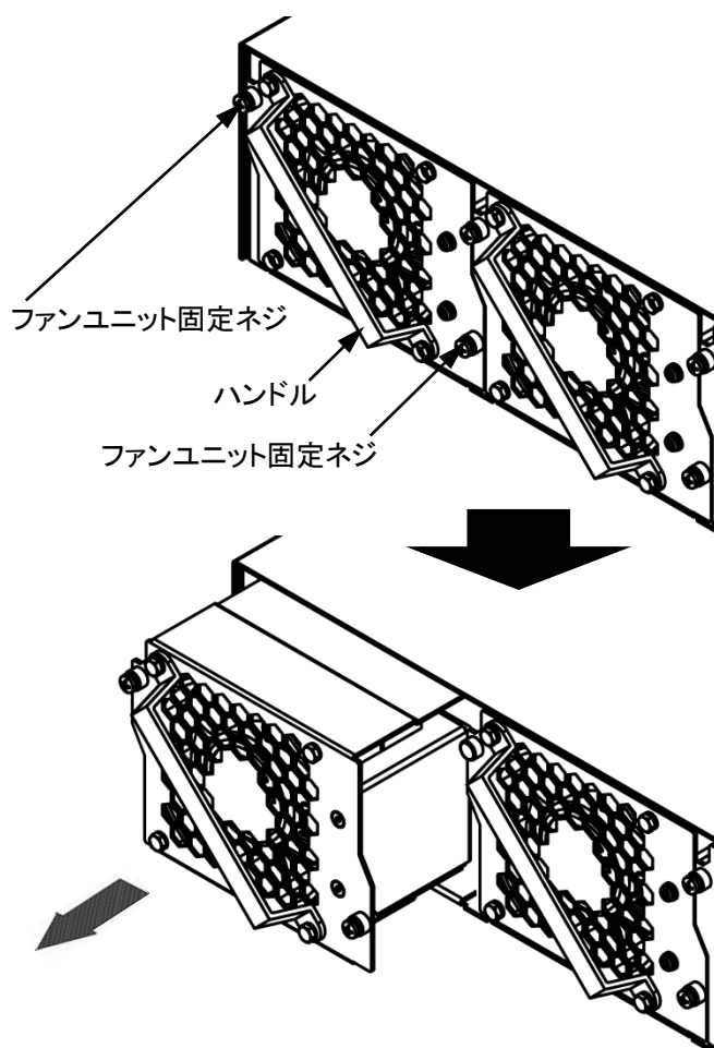
図 4.1.1-1 ファンユニットの取り外し
