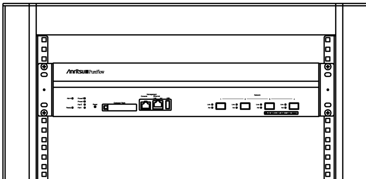
図 2.4.2-5 ラックへの装置搭載
