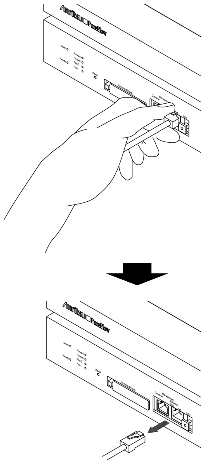
図 2.8.2-1 UTP ケーブルの取り外し
