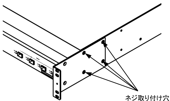
図 2.4.2-3 取り付け穴の位置(後方位置)
