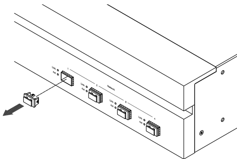
図 2.6.2.1-1 SFP ケージプラグの取り外し
