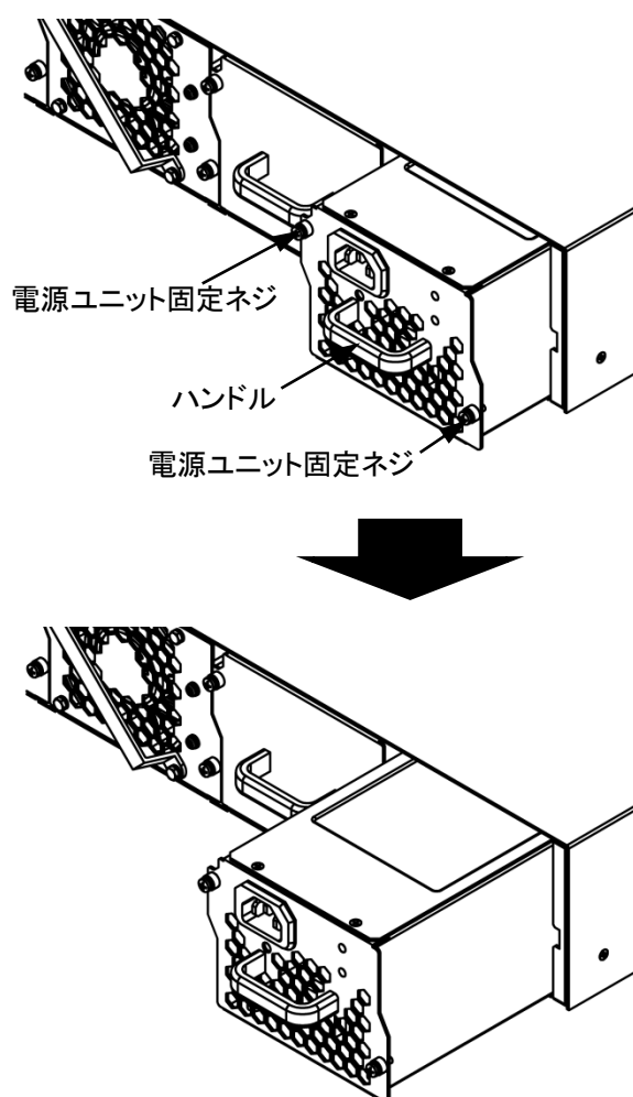
図 4.2.1-1 電源ユニットの取り外し
