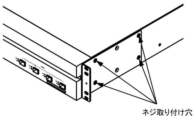
図 2.4.2-2 取り付け穴の位置(標準位置)
