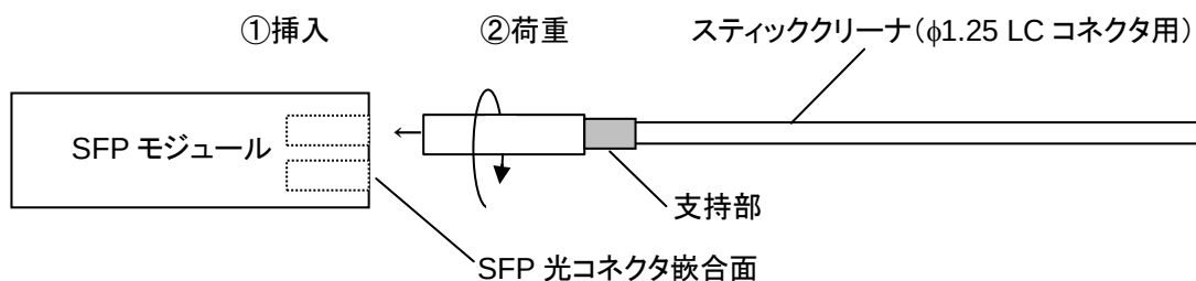
図 2.6.1.1-1 スティッククリーナの使用例
