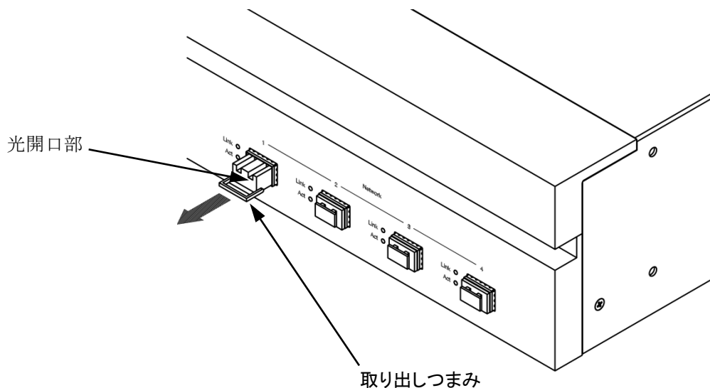
図 2.6.2.2-1 SFP モジュール取り外し
