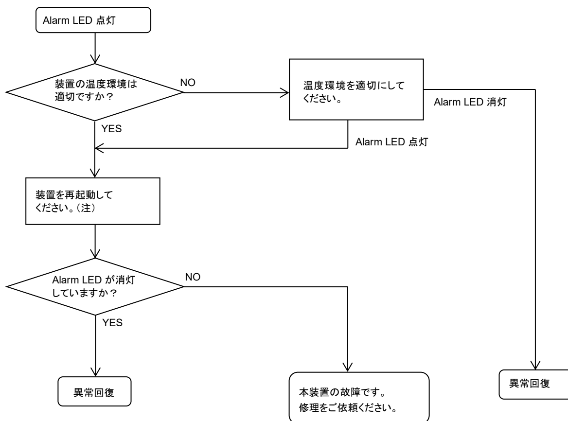
図 5.2.3-1 そのほかの異常探求フロー
