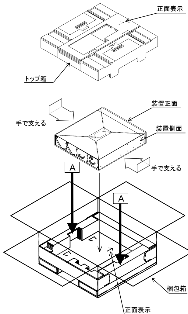
図 2.12.1-1 梱包方法
