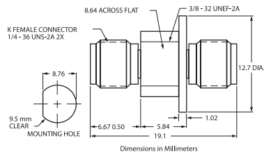
K232B outline
