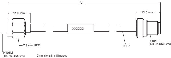
K120MF outline
