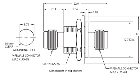
V232 outline
