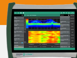
各種無線設備のフィールド検証用 多機能スペクトラムアナライザ MS2080A
