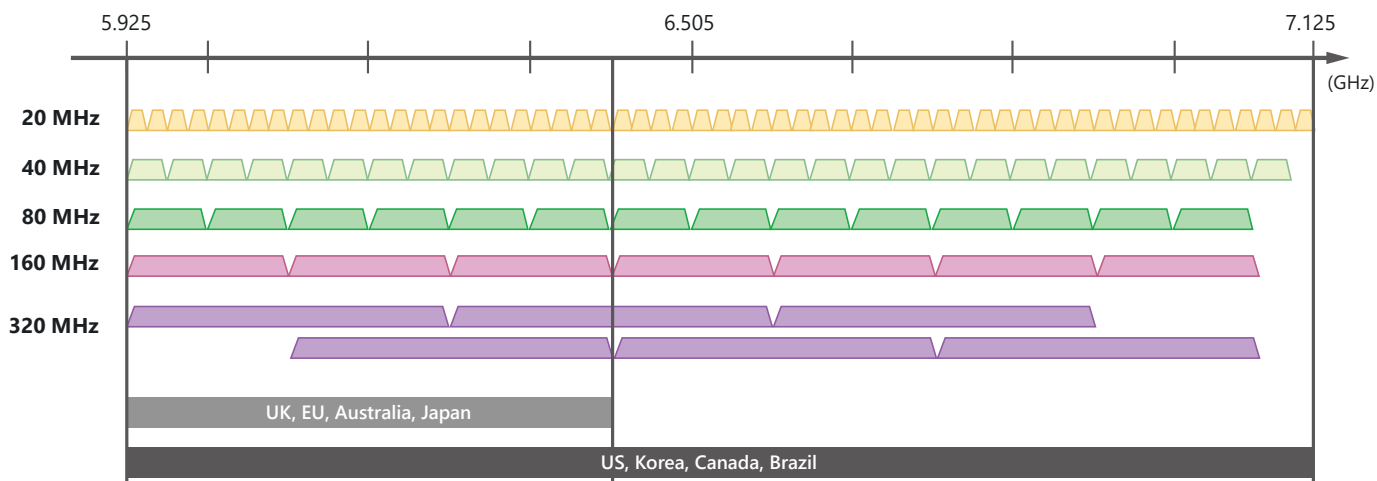
図2 無線LANで使用する周波数帯
