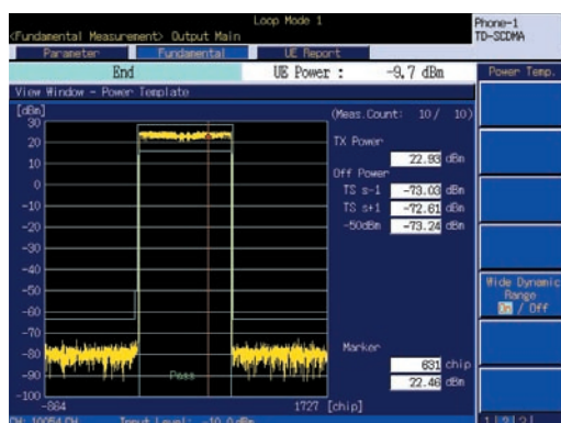
テンプレート判定
