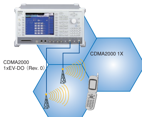
MT8820Bとの接続例：MT8820B 1台 (パラレルフォン測定対応) の場合
