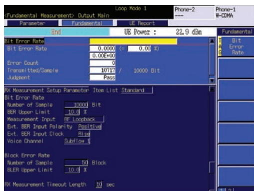
ビット誤り率測定
