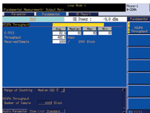
スループット・モニタ
