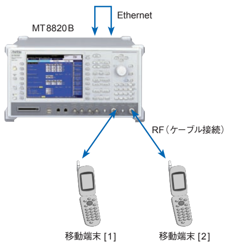
MT8820Bとの接続例：MT8820B 1台 (パラレルフォン測定対応) の場合
