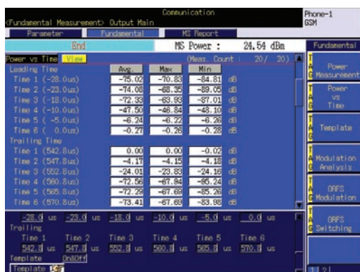
電力対時間 (GSM)
