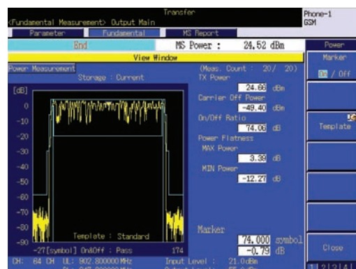
バースト波形表示 (8PSK)
