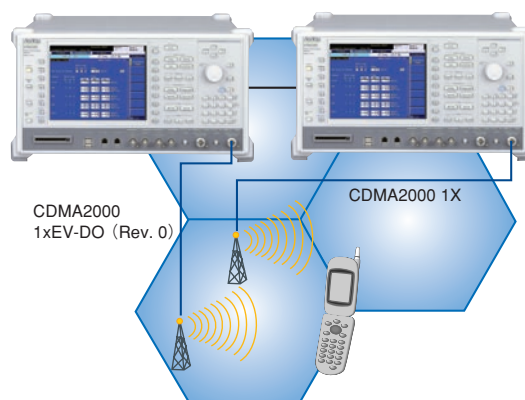
MT8820Bとの接続例：MT8820B 2台の場合
