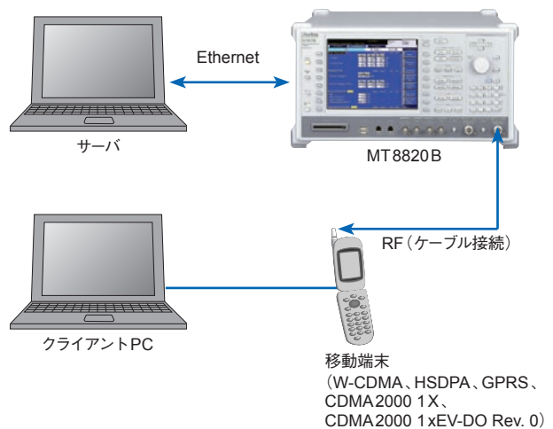
MT8820Bとの接続例
