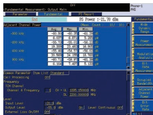
隣接チャネル漏洩電力
