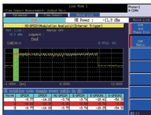
コード・ドメイン・パワー測定
