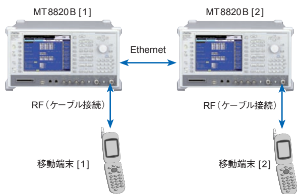
MT8820Bとの接続例：MT8820B 2台の場合
