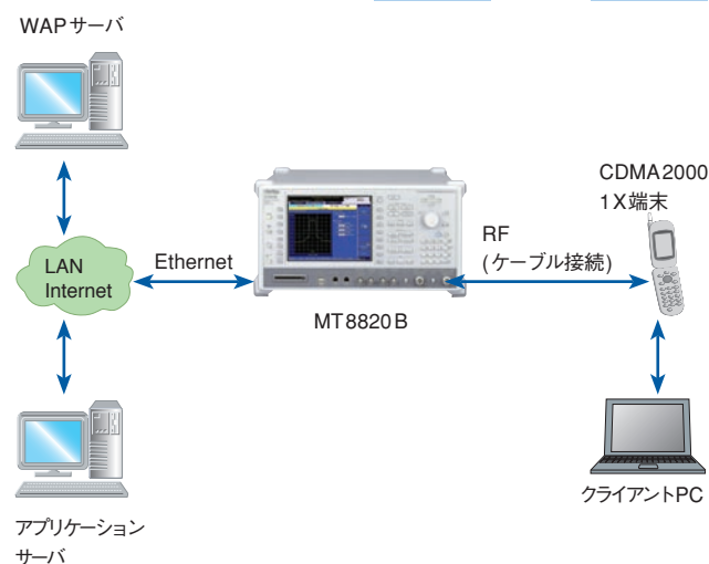
IPデータ通信モード接続例
