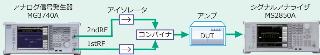
アンプの相互変調特性測定構成例
