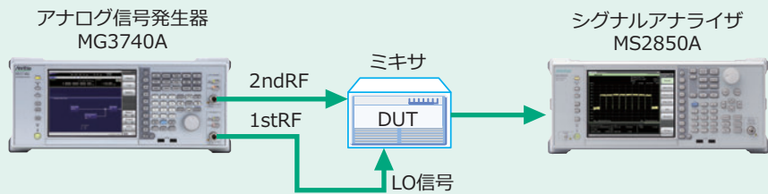
ミキサの歪み特性測定構成例
