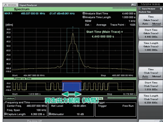
キャプチャした波形を任意の範囲(時間)で切り出して連続再生出力
