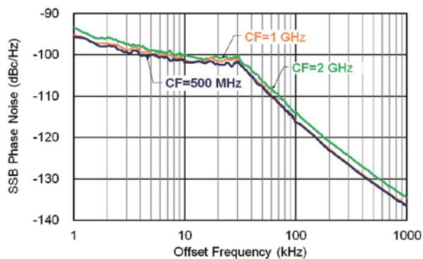
SSB位相雑音の一例 (スペクトラムアナライザ、シグナルアナライザ 共通)
