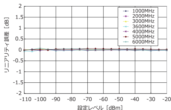
リニアリティの一例 (基準レベル -15 dBm)
