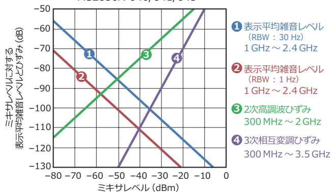
ひずみ特性 (スペクトラムアナライザ) MS2830A-040/041/043
