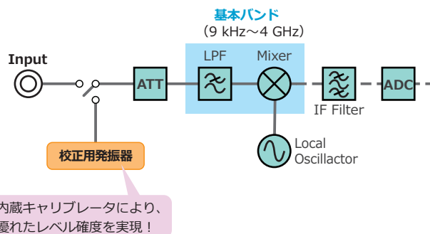
MS2830A ブロック図
