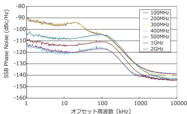
SSB位相雑音の一例
