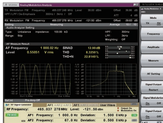
FM変調信号出力 (下側) とAF信号測定 (上側) の測定例
