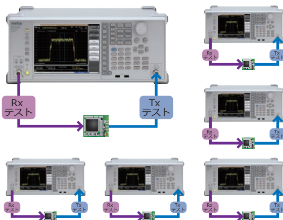
ゴールデンユニットの信号を製造検査やキャリブレーションに使用
