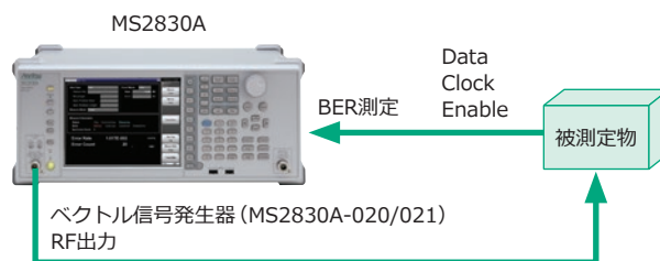
BER測定セットアップ例 (MS2830A-020/021搭載時)
