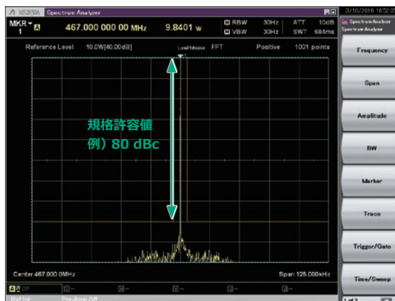
スプリアス発射 (帯域外領域) 測定の一例
