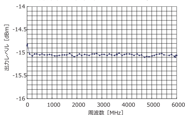
周波数特性の一例 (基準レベル -15 dBm)
