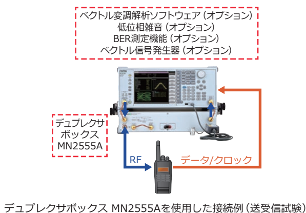
デュプレクサボックス MN2555Aを使用した接続例 (送受信試験)
