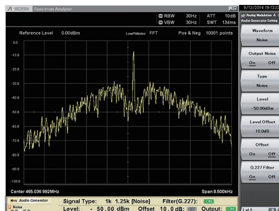
G.227擬似音声出力 (下側) とスペクトラムアナライザ (上側) の測定例
