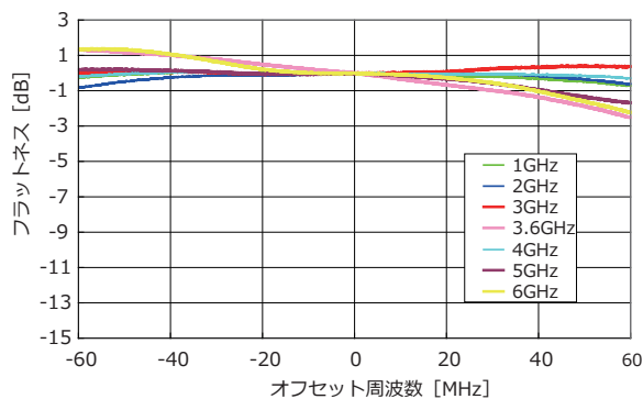
ベクトル変調帯域幅の一例
