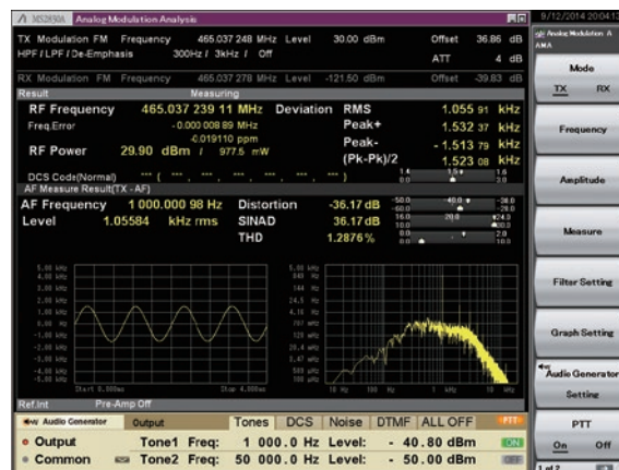
AF信号出力 (下側) とFM変調信号測定 (上側) の測定例
