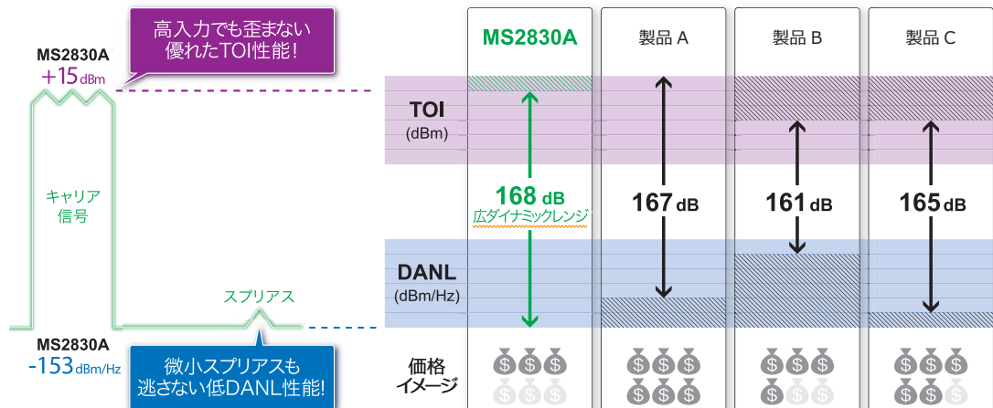
ひずみ特性 (スペクトラムアナライザ) MS2830A-040/041/043
