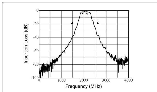
周波数特性
