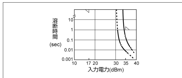
入力電力と溶断時間特性の例
