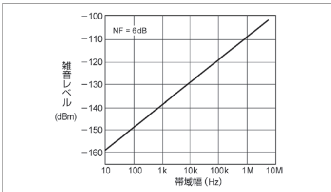
入力換算雑音レベルとIF帯域幅
