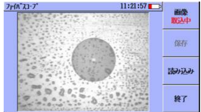
汚れの付着した光ファイバのフェルルール端面例
