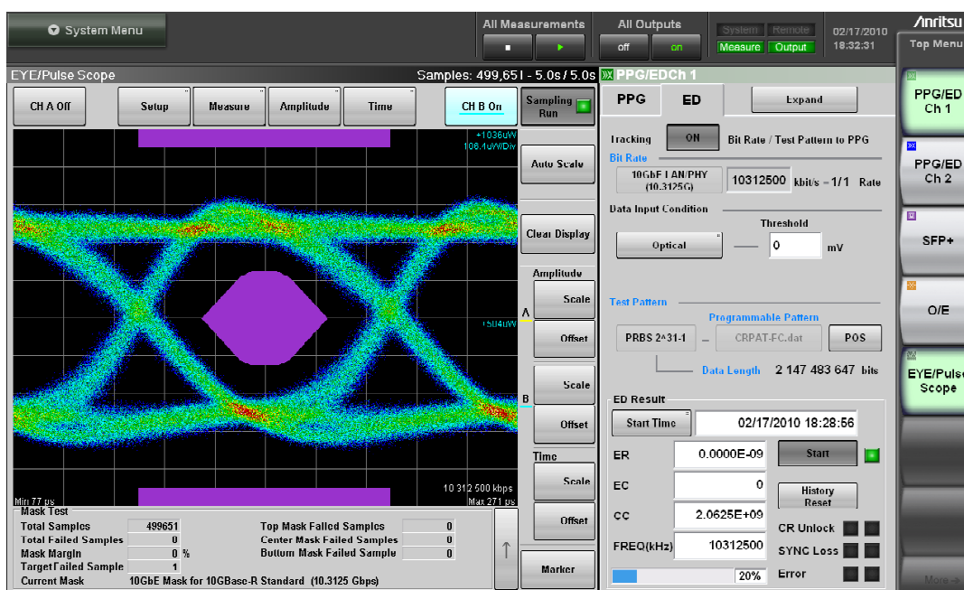
BERとアイパターンの同時測定画面
