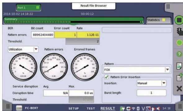
メータ表示、カラー合否判定表示により、問題点をすばやく認識
