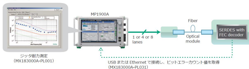
電気FEC信号伝送評価
