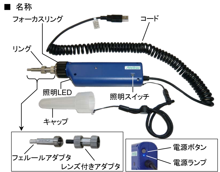
図 2 各部の名称
