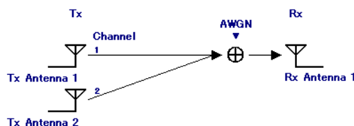
図3.1.2.2-5 2x1 MISO
