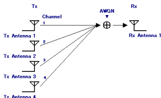
図3.1.2.2-13 4x1 MISO
