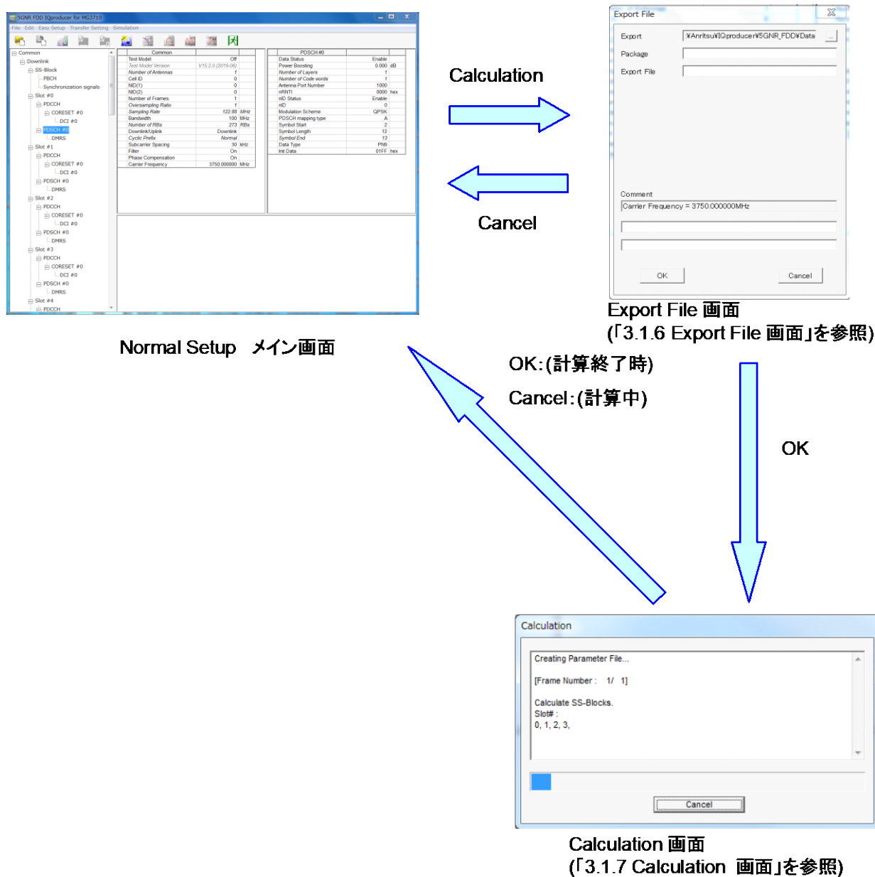
図3.1.1.3-1 画面遷移
