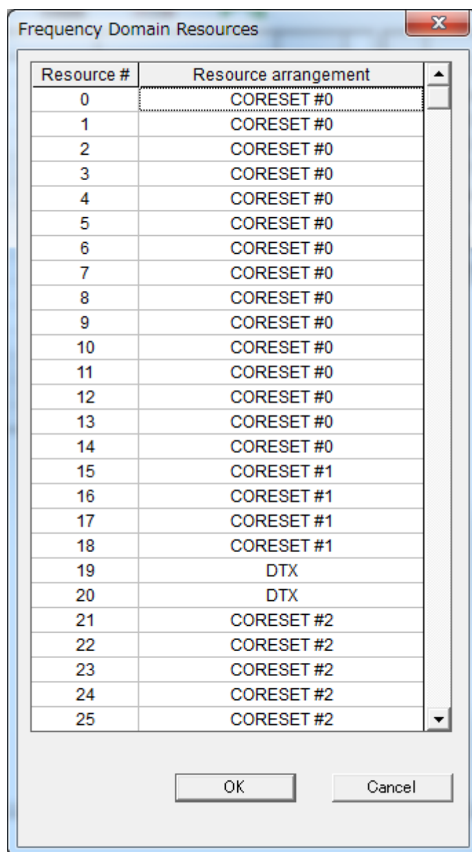
図3.1.4.5-1 Frequency Domain Resourcesダイアログボックス
