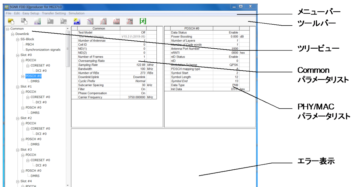
図3.1.1-1 Normal Setup メイン画面
