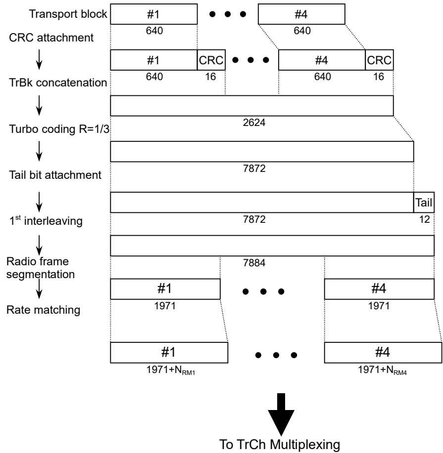
図3.1.2-3 UL ISDN のチャネルコーディング
