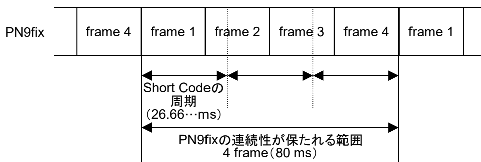
図3.8.1-3 PN9fix データとショートコード
