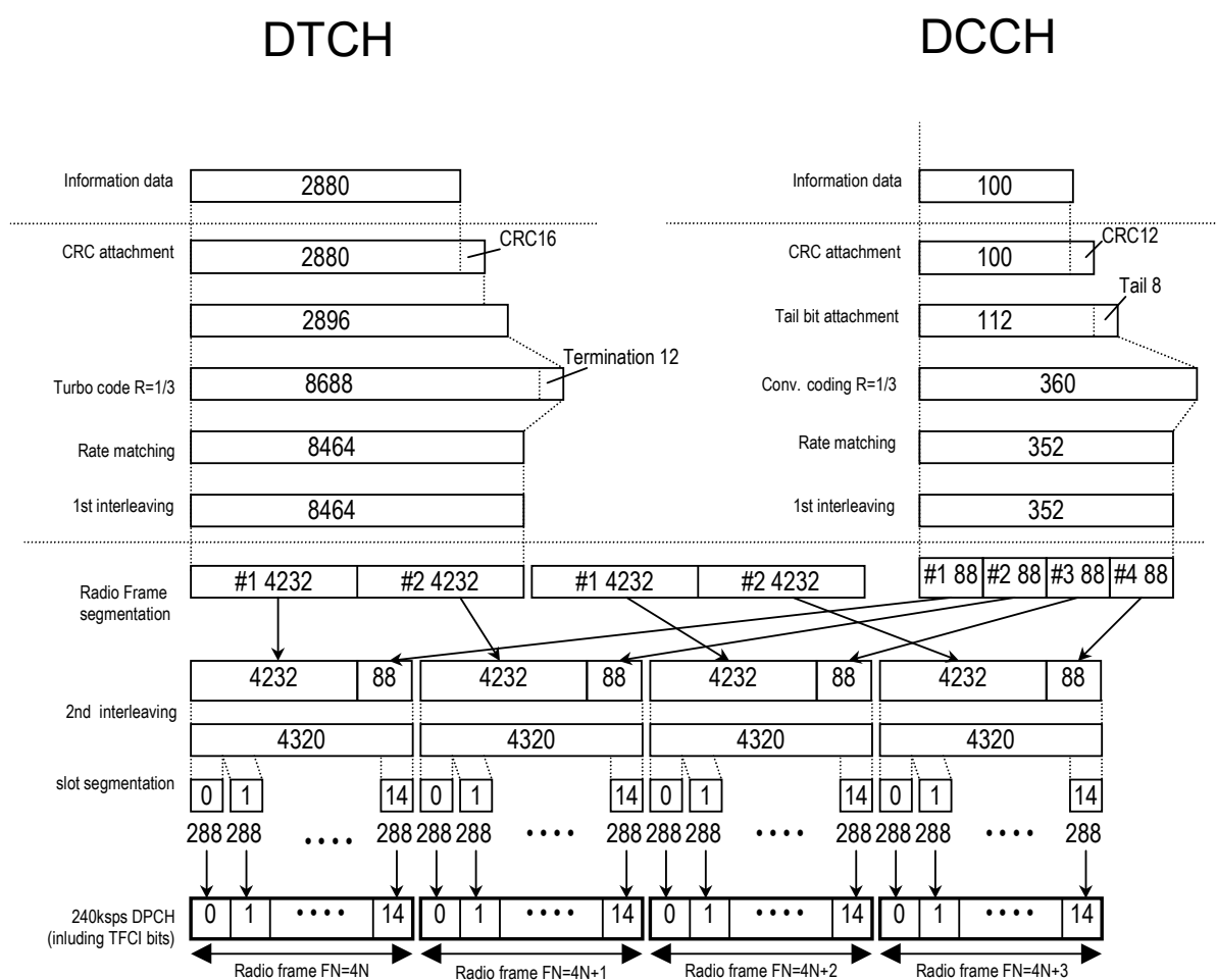
図3.1.4-3 DL reference measurement channel (144 kbps) のチャンネルコーディング
