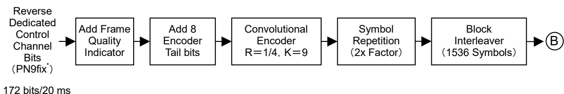
図3.8.5-2 波形パターン RVS_RC3_DCCH 信号生成のブロックダイアグラム (1/2)
