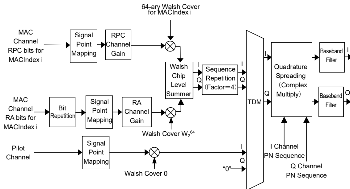
図3.9.3-1 1xEV-DO フォワードアイドルスロットのブロック図
