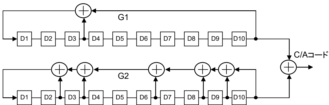
図3.18.1-3 C/A コード生成法
