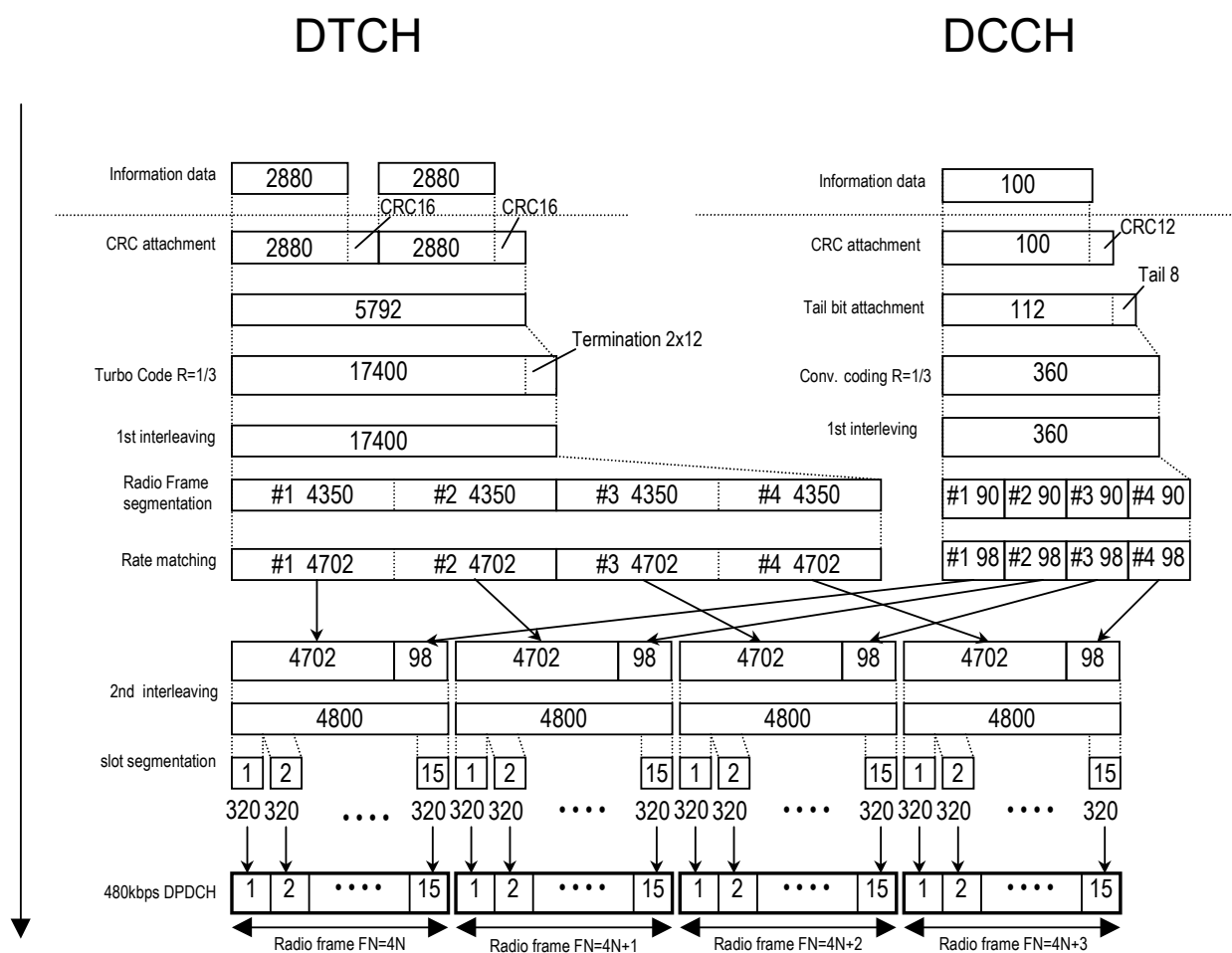
図3.1.1-4 UL reference measurement channel (144 kbps) のチャネルコーディング
