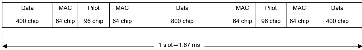
図3.9.1-3 1xEV-DO フォワード (アイドルスロットを除く) のスロットのフォーマット
