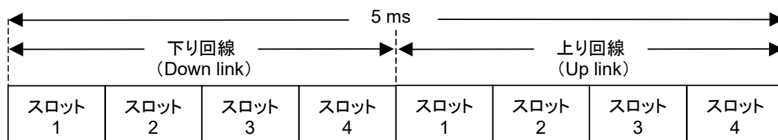
図3.6.1-1 PHS のフレーム構造
