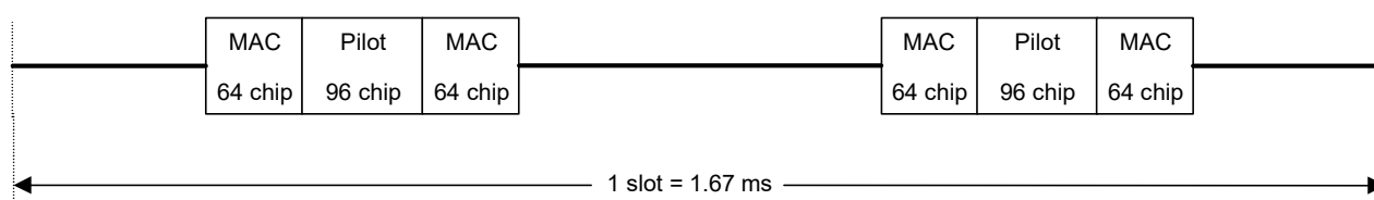
図3.9.3-2 1xEV-DO フォワードアイドルスロットのフォーマット
