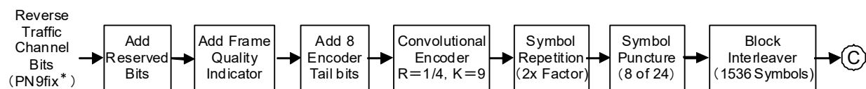
図3.8.6-2 波形パターン RVS_RC4_FCH の信号生成ブロックダイアグラム (1/2)
