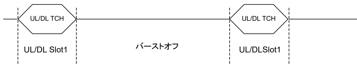
図3.6.1-2 PHS のフレーム構造
