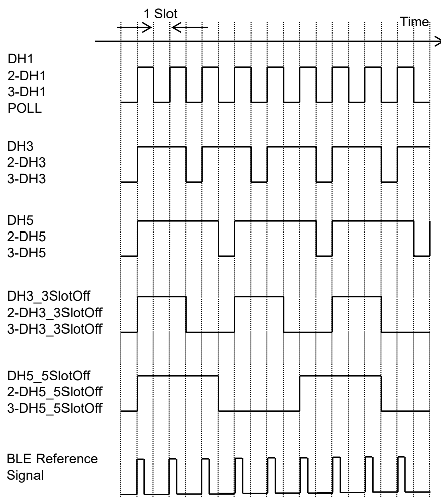
図3.12-1 波形パターンのタイミングチャート
