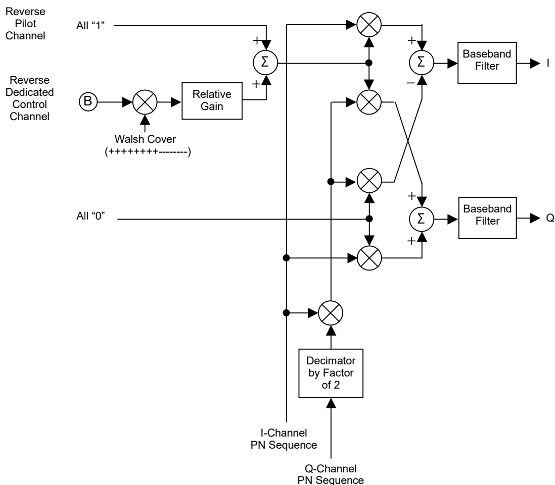
図3.8.5-2 波形パターン RVS_RC3_DCCH 信号生成のブロックダイアグラム (1/2)
