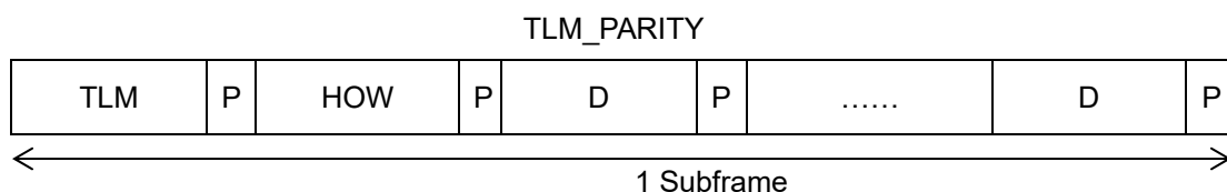
図3.13.1-2 PN9、PARITY 波形のフォーマット
