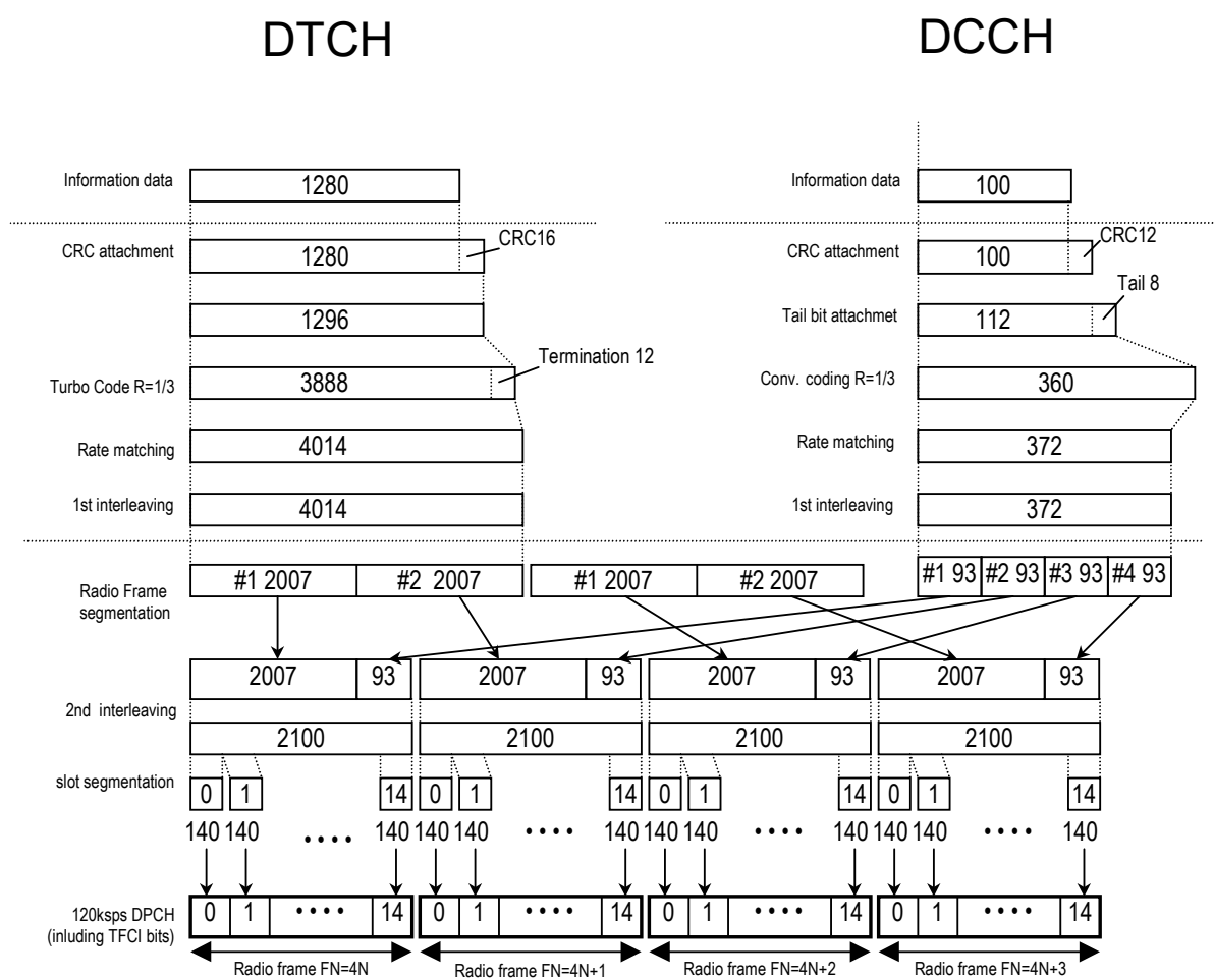
図3.1.4-2 DL reference measurement channel (64 kbps) のチャネルコーディング
