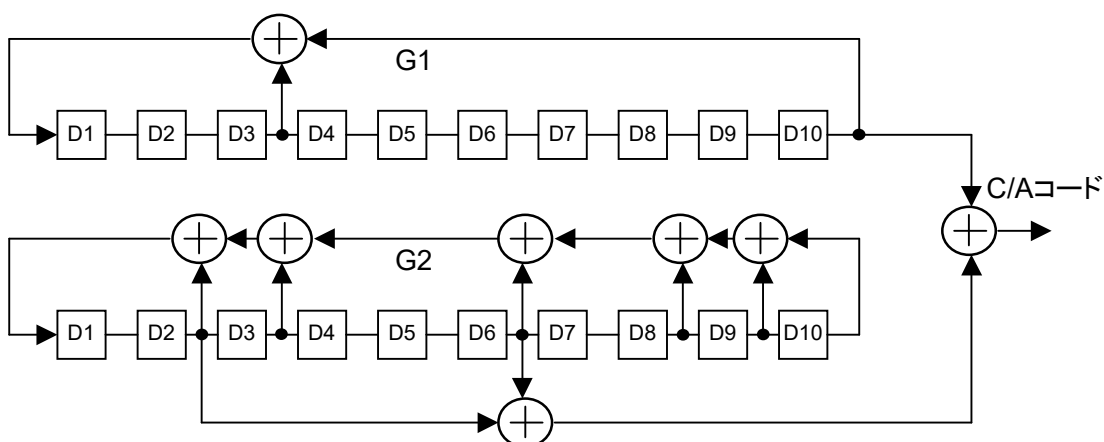
図3.13.1-4 C/A コード生成法
