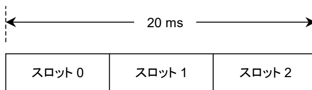
図3.4.1-1 フルレートのフレーム構造
