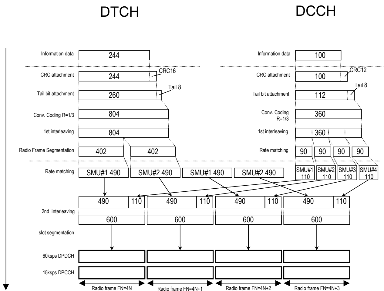
図3.1.1-2 UL reference measurement channel (12.2 kbps) のチャネルコーディング
