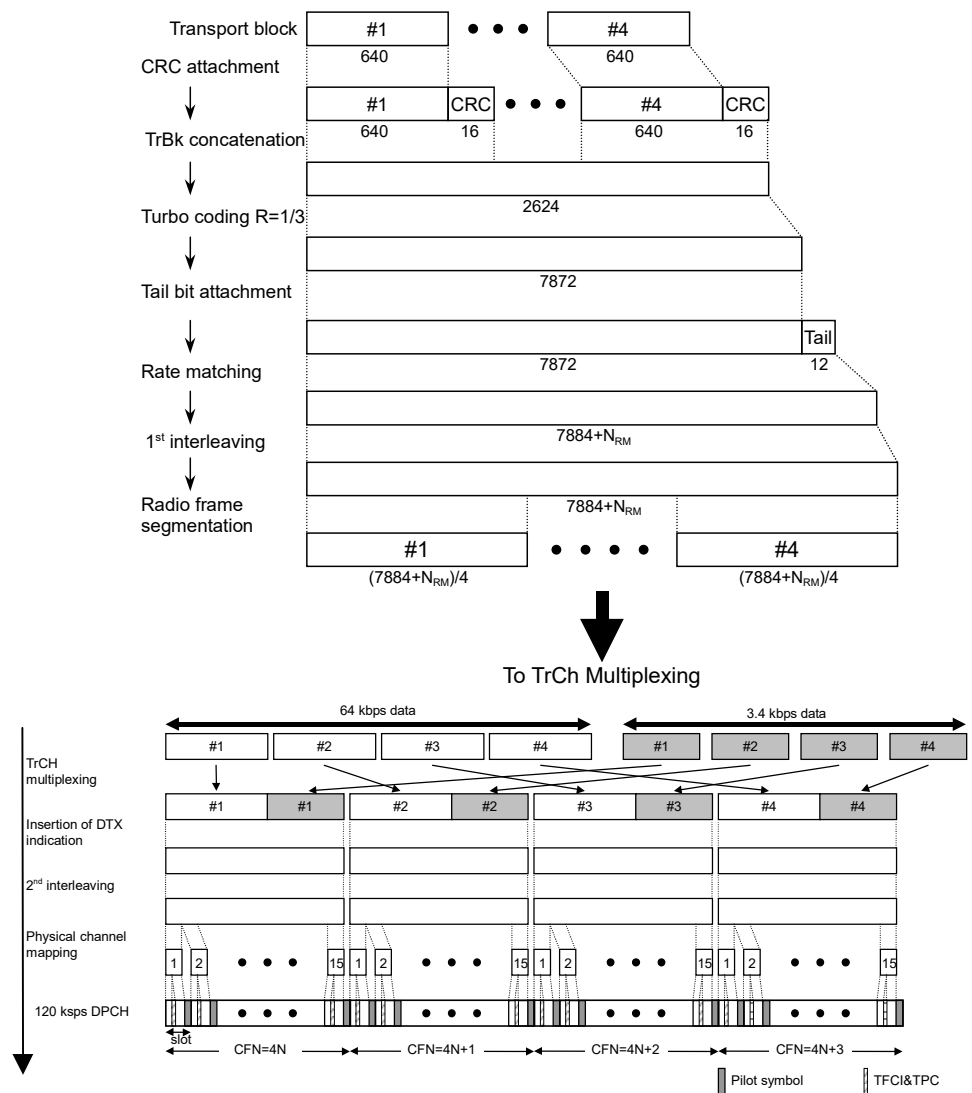
図3.1.5-3 DL ISDN のチャンネルコーディングと多重
