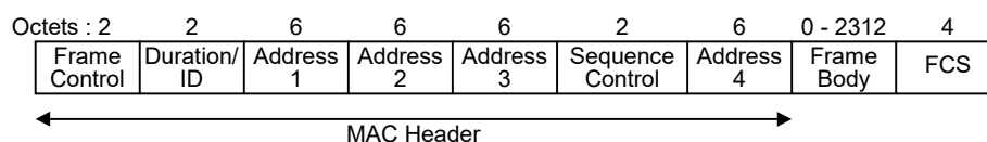
図3.10.1-2 IEEE802.11a MAC フレームフォーマット
