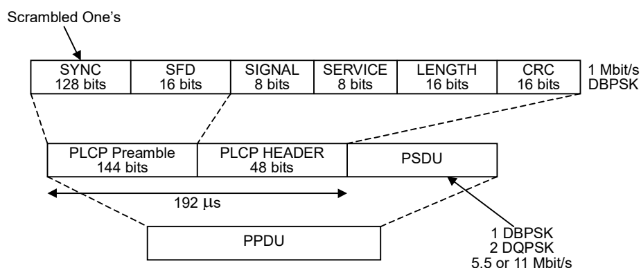
図3.10.2-1 IEEE802.11b Long PLCP PPDU フレームフォーマット
