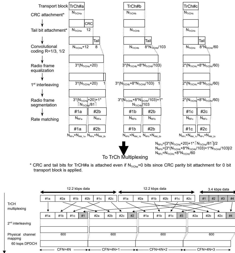
図3.1.2-2 UL AMR TFCSx のチャネルコーディングと多重 (2/2)
