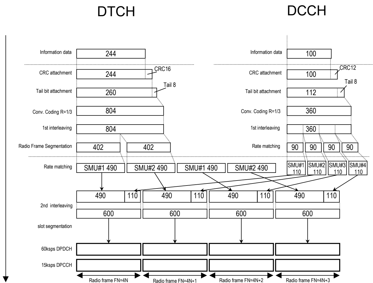
図3.1.1-1 UL reference measurement channel (12.2 kbps) のチャネルコーディング
