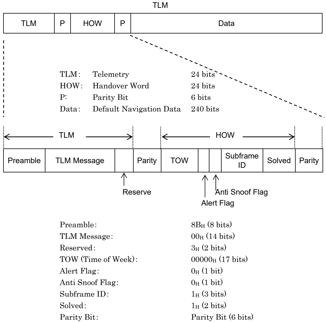
図3.18.1-1 DefaultNavData 波形のフォーマット
