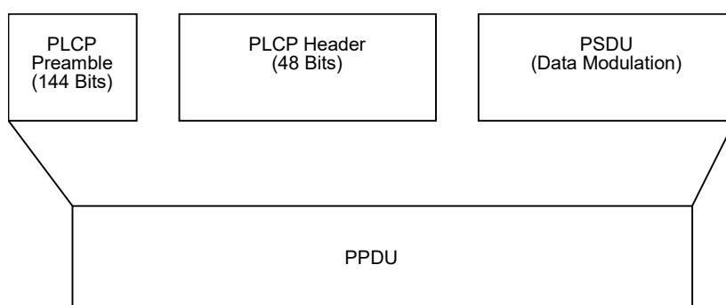
図3.10.3-1 IEEE802.11g Long preamble PPDU フレームフォーマット
