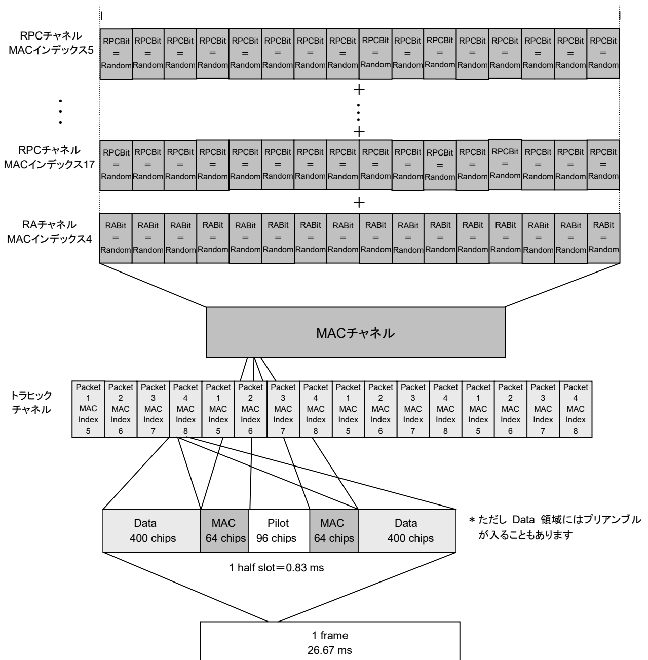
図3.9.1-5 各チャネルの多重
