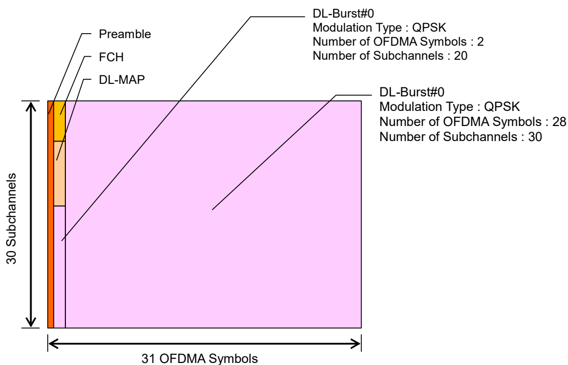
図3.14.1-1 WiMAX_DL_10MHz_QPSK のフレーム構成
