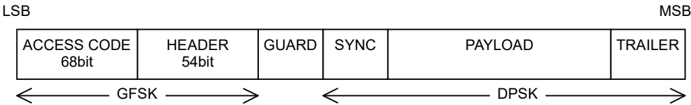
図3.12.2-1 Enhanced Data Rate 波形のパケット構造
