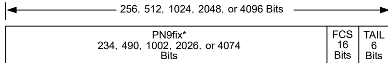
図3.9.2-1 1xEV-DO リバースのパケットのフォーマット
