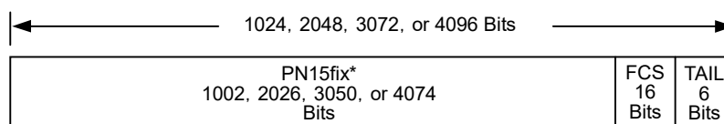
図3.9.1-1 1xEV-DO フォワードのパケットのフォーマット
