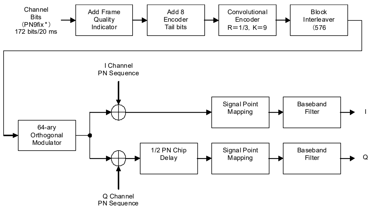
図3.8.1-2 波形パターン RVS_RC1_FCH の信号生成ブロックダイアグラム
