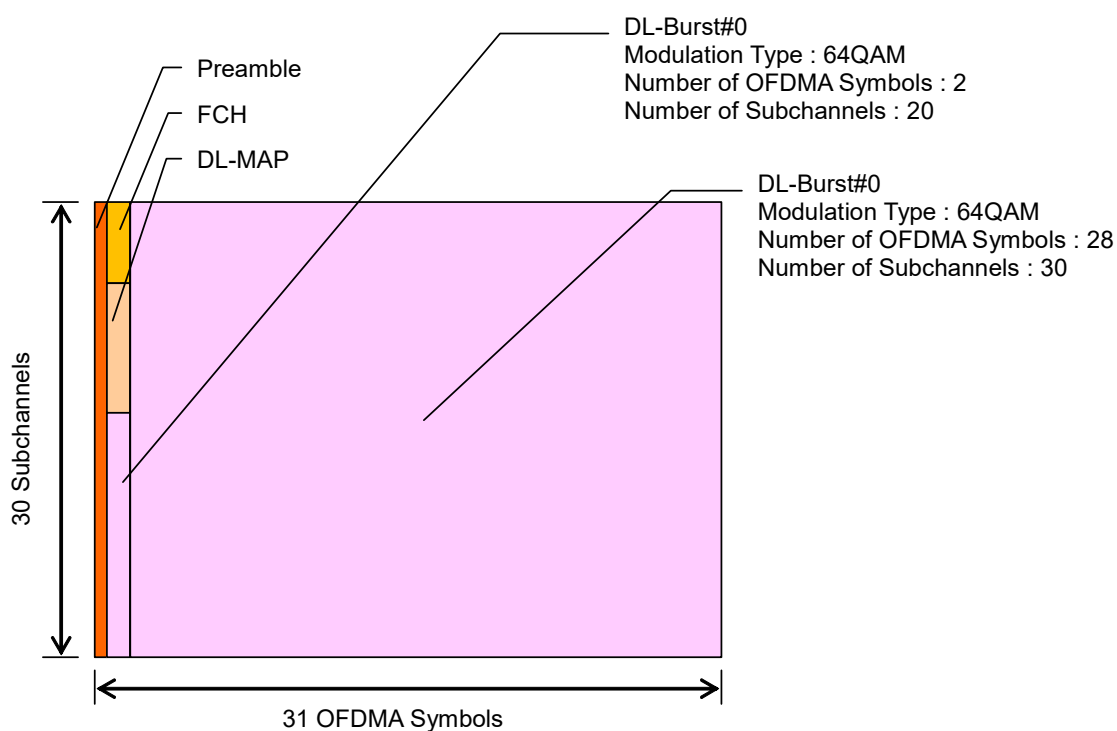
図3.14.1-2 WiMAX_DL_10MHz_64QAM のフレーム構成
