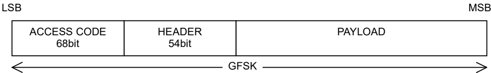
図3.12.1-1 Basic Rate 波形の packets 構成
