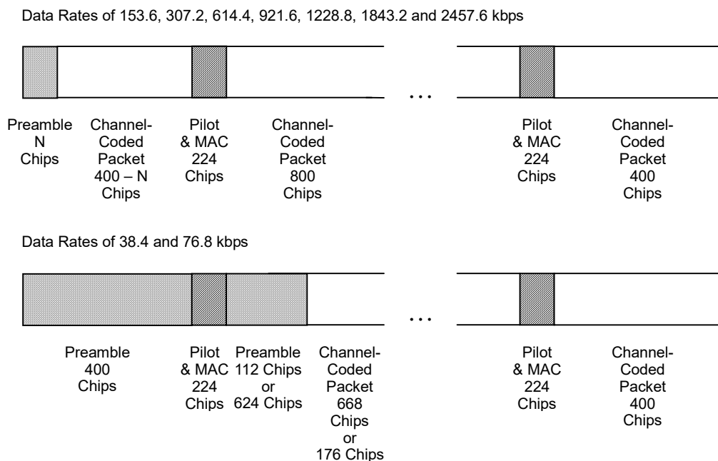
図3.9.1-4 タイミングダイヤグラム
