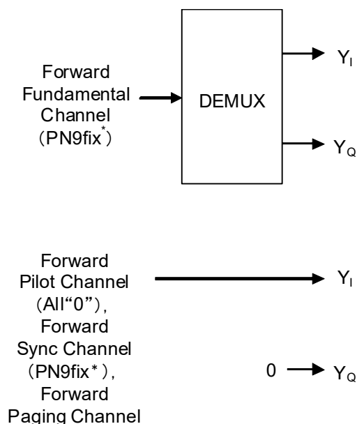
図3.8.8-1 波形パターン FWD_RC3-5 9channel のブロックダイアグラム (1/2)
