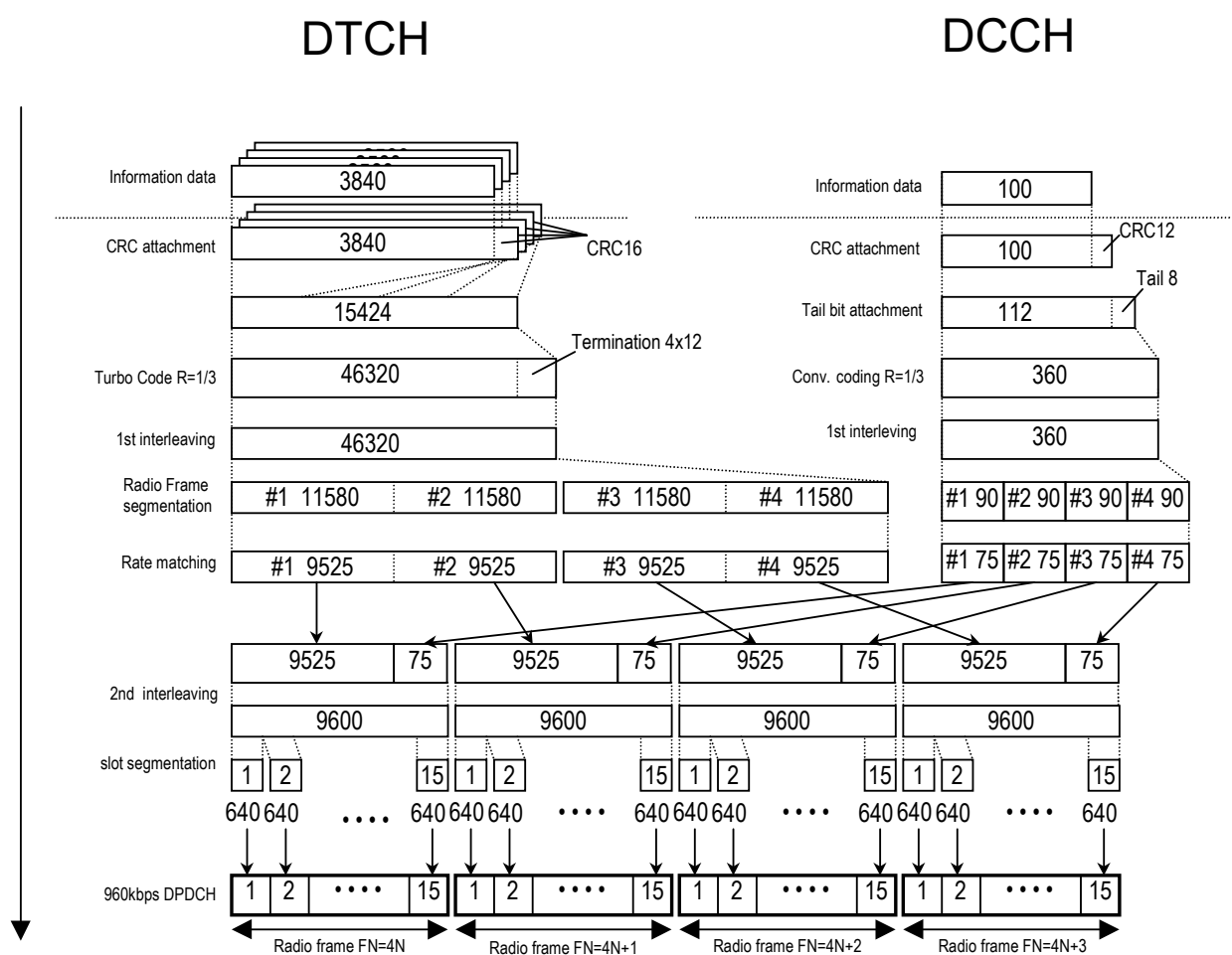
図3.1.1-5 UL reference measurement channel (384 kbps) のチャネルコーディング
