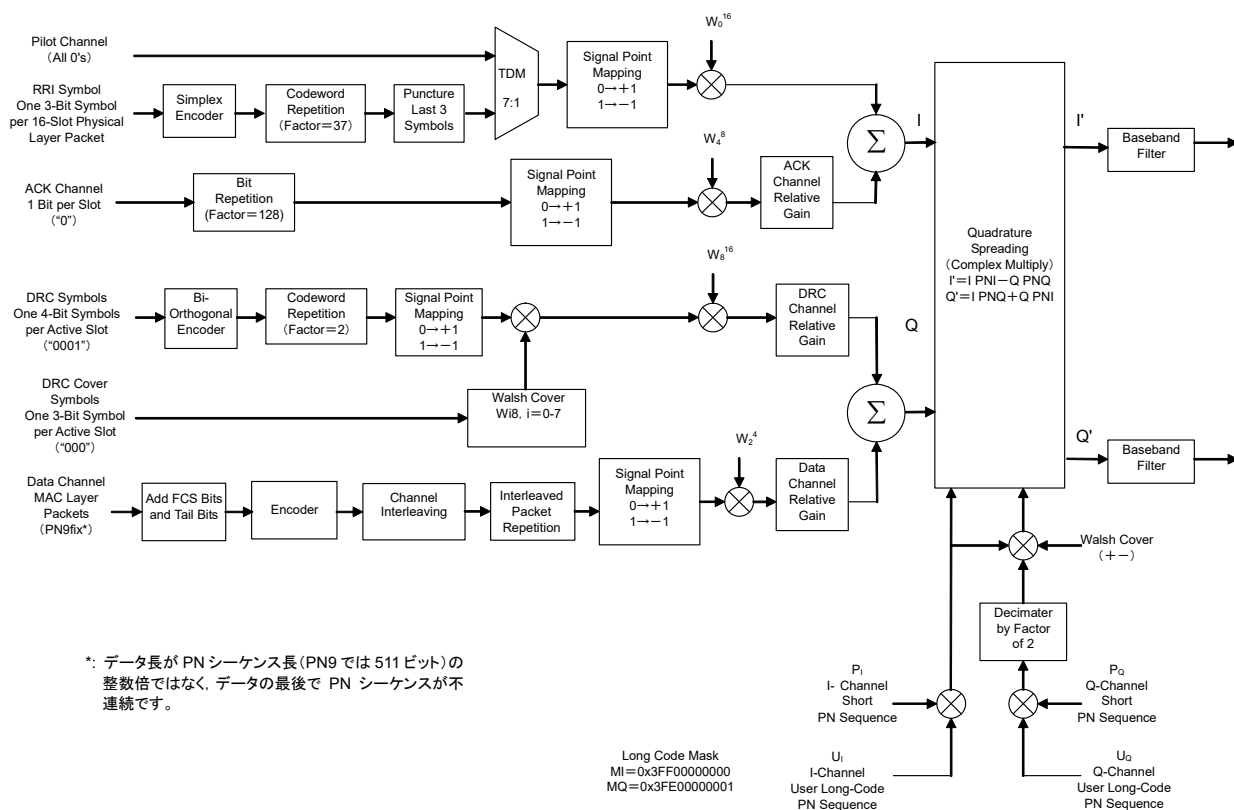
図3.9.2-2 1xEV-DO リバースブロックダイアグラム
