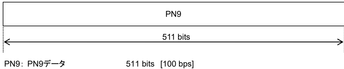
図3.17.1-2 GLONASS_PN9 波形のフォーマット
