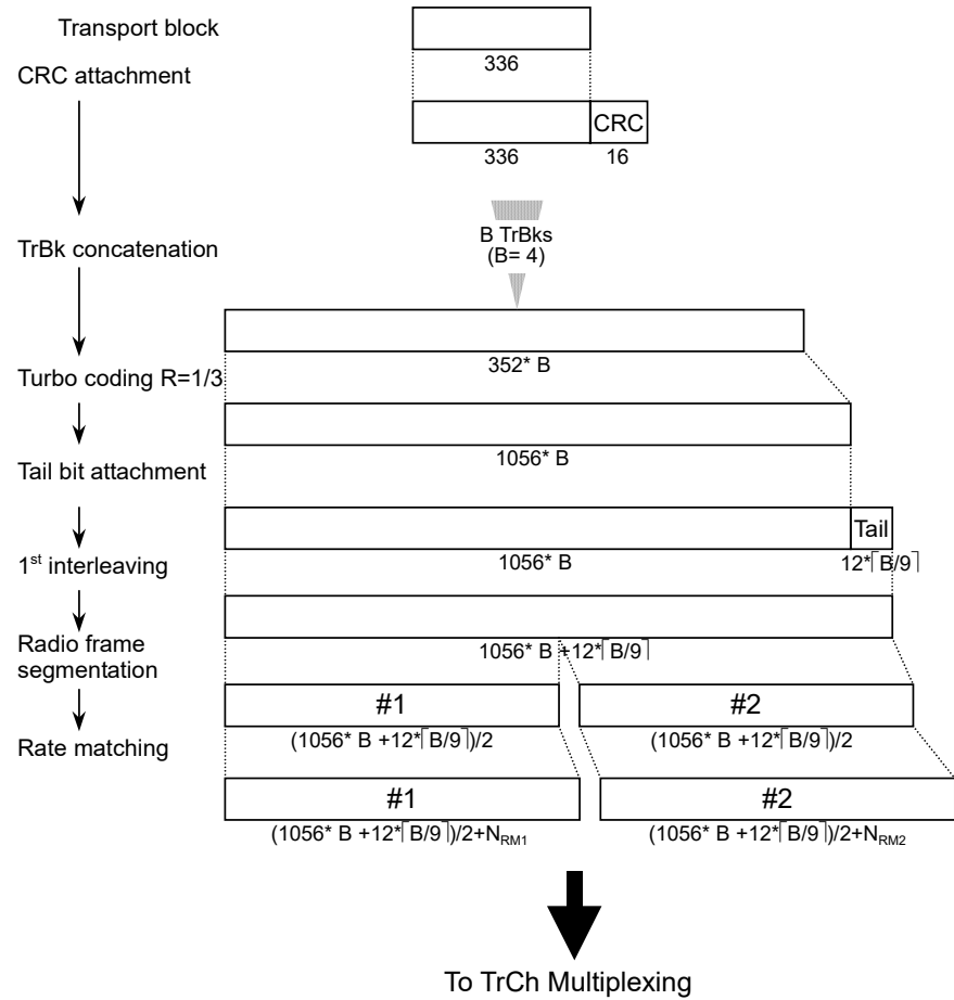
図3.1.2-5 UL 64 kbps Packet のチャネルコーディング
