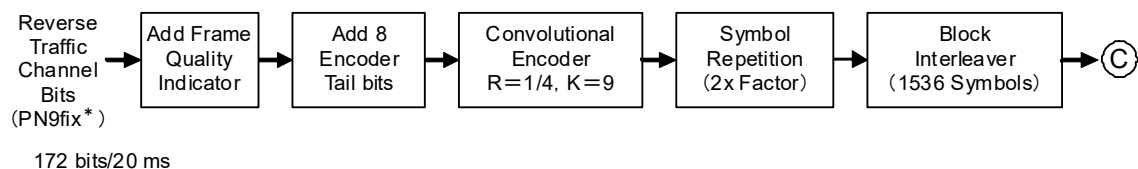
図3.8.4-2 波形パターン RVS_RC3_FCH_SCH の信号生成ブロックダイアグラム (1/2)
