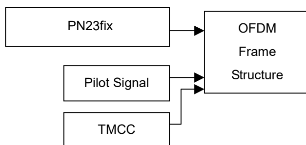
図3.11.1-2 ISDB-T の波形パターンの生成
