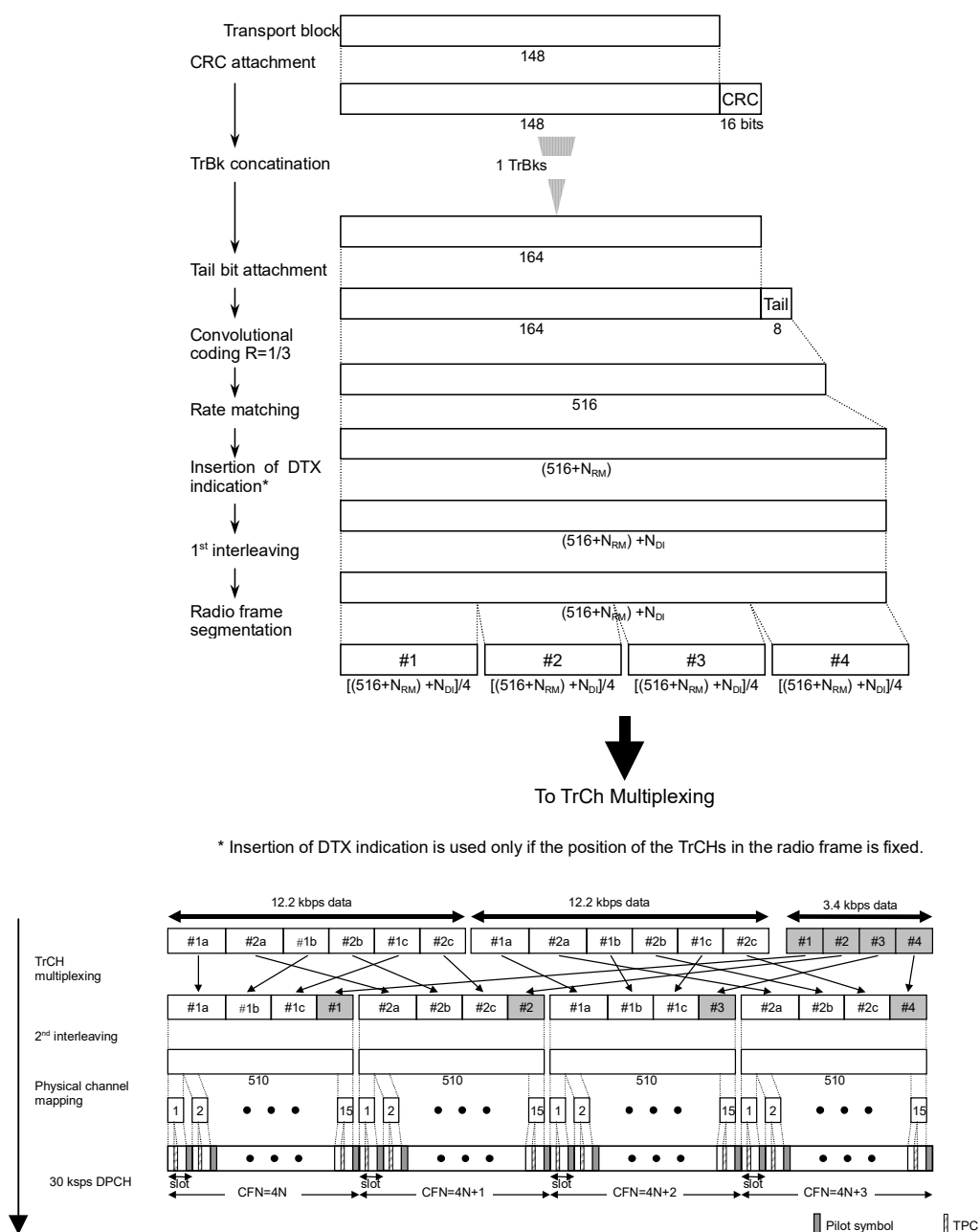
図3.1.5-2 DL AMR TFCSx のチャネルコーディングと多重 (2/2)
