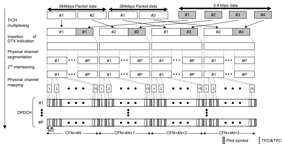
図3.1.5-5 DL 384 kbps Packet の多重
