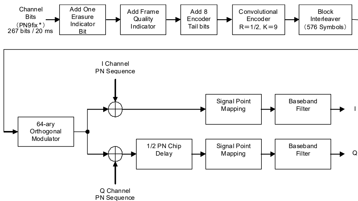
図3.8.2-2 波形パターン RVS_RC2_FCH のブロックダイヤグラム
