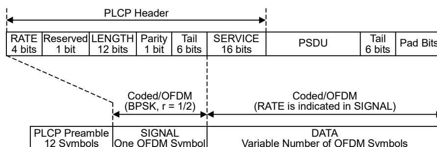
図3.10.1-1 IEEE802.11a PPDU フレームフォーマット
