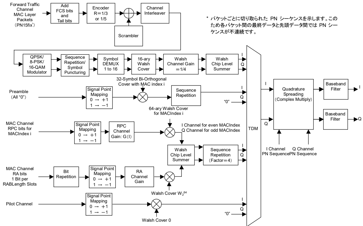
図3.9.1-2 1xEV-DO フォワードブロックダイアグラム
