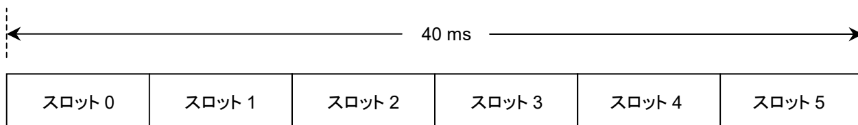
図3.4.1-2 ハーフレートのフレーム構造
