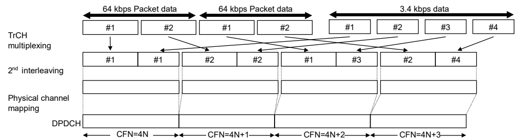
図3.1.2-4 UL ISDN の多重
