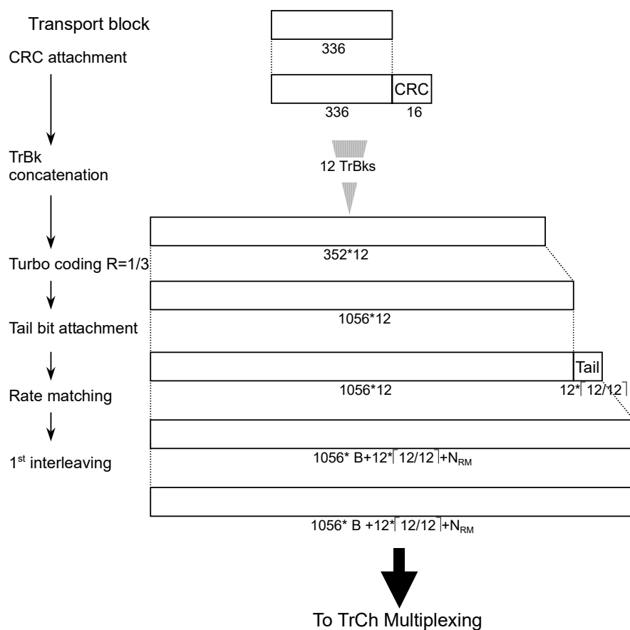
図3.1.5-4 DL 384 kbps Packet のチャネルコーディング
