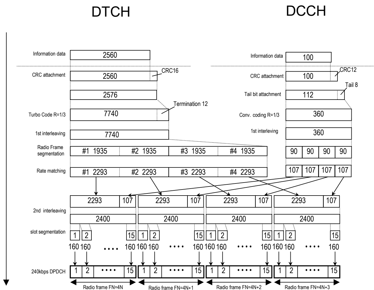
図3.1.1-3 UL reference measurement channel (64 kbps) のチャネルコーディング
