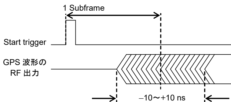
図3.13-1 SYNC_ADJ の出力タイミング
