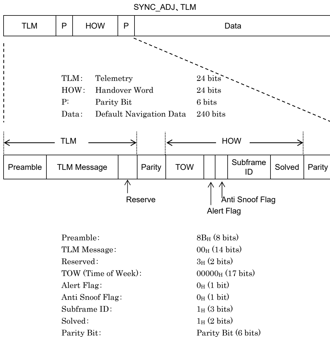
図3.13.1-1 SYNC_ADJ、TLM 波形のフォーマット
