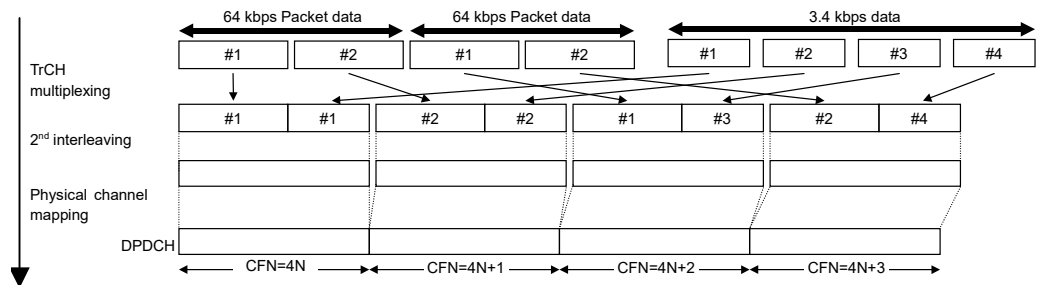
図3.1.2-6 UL 64 kbps Packet の多重
