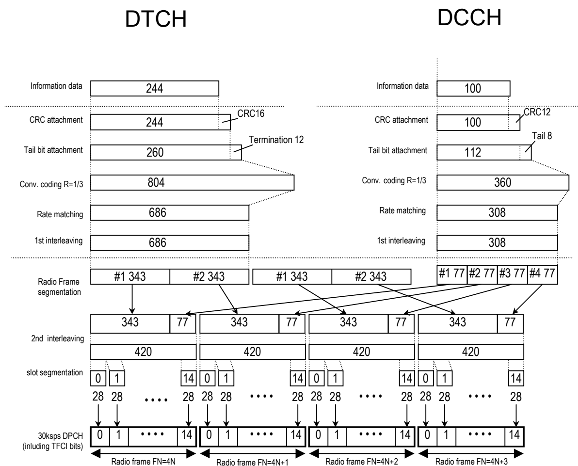
図3.1.4-1 DL reference measurement channel (12.2 kbps) のチャネルコーディング
