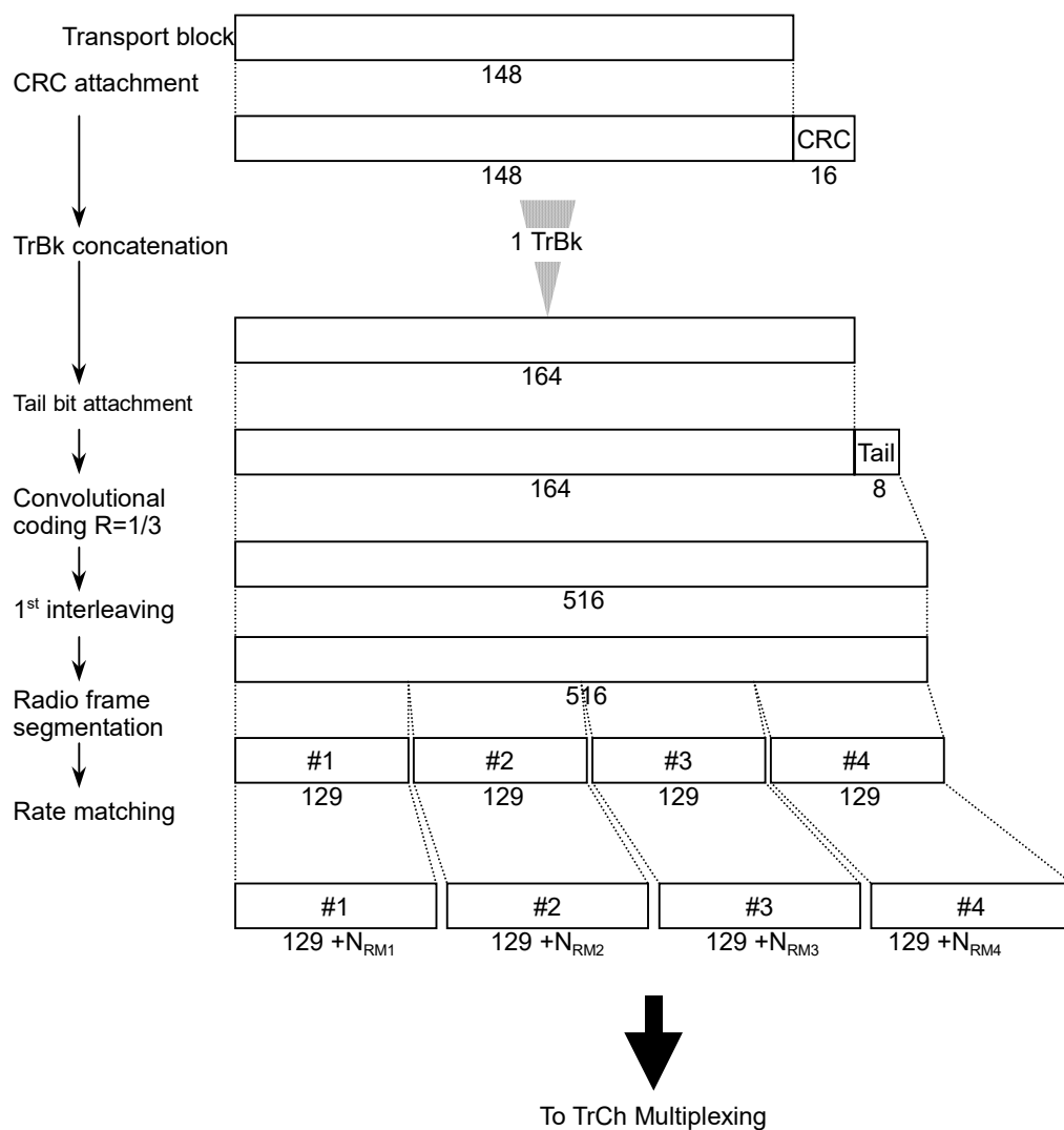
図3.1.2-1 UL AMR TFCSx のチャネルコーディングと多重 (1/2)
