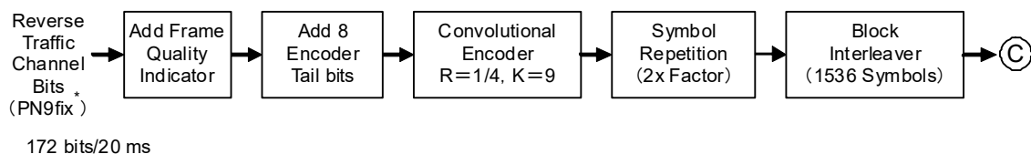
図3.8.3-2 波形パターン RVS_RC3_FCH の信号生成ブロックダイアグラム (1/2)
