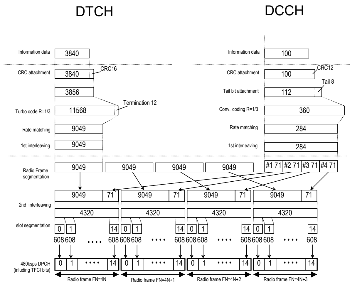
図3.1.4-4 DL reference measurement channel (384 kbps) のチャネルコーディング
