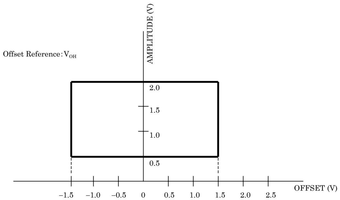
図4 DATA 出力振幅, オフセット設定範囲 (終端条件 50 \Omega / -2 \text{ V} )
