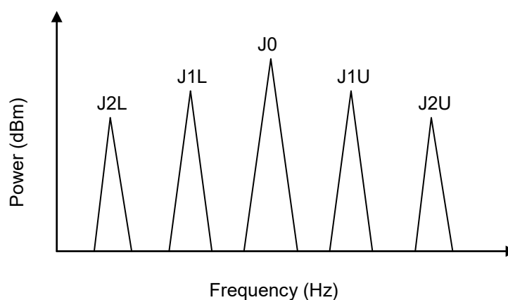
図5.1.2-1 スペクトラム波形
