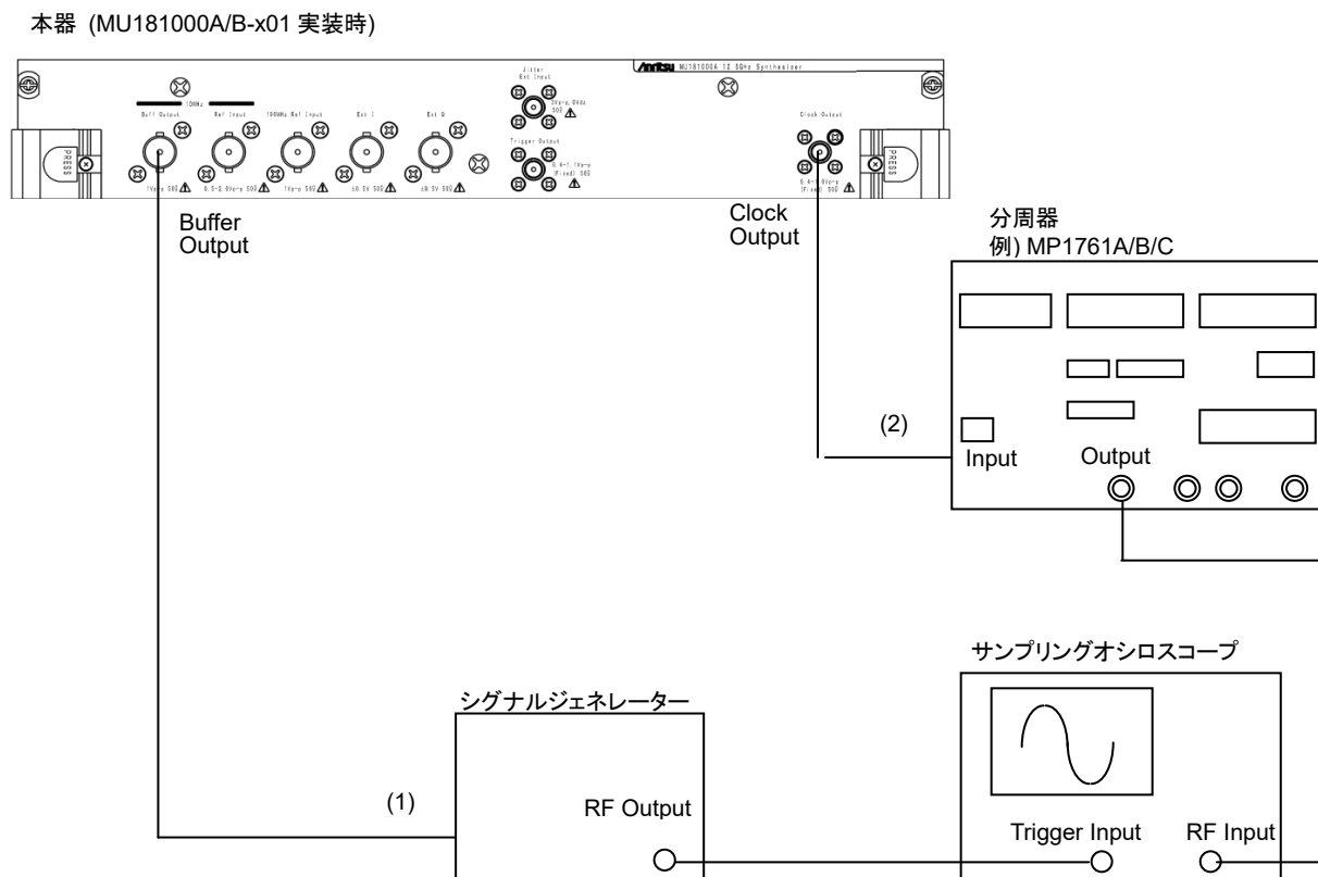
図6.3.5-1 三角波変調測定の接続図
