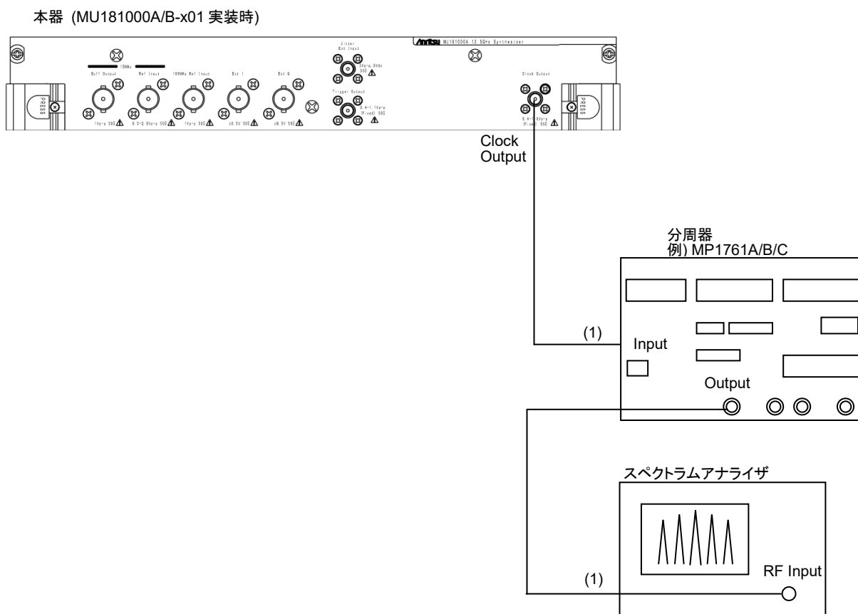
図6.3.3-2 0.4 Ulp-p 以上の正弦波ジッタ測定の接続
