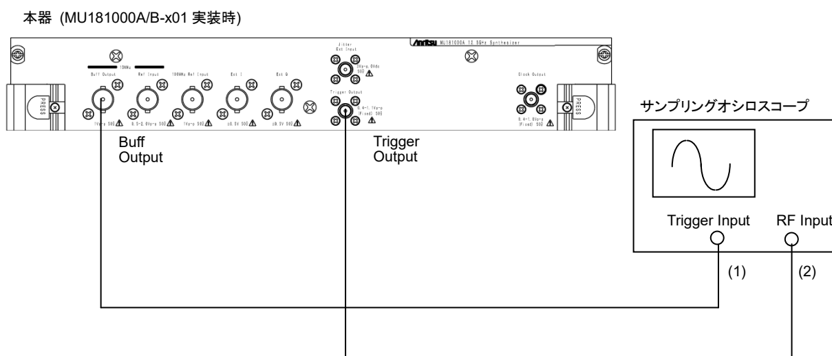
図6.3.6-1 トリガ出力波形測定のための接続図
