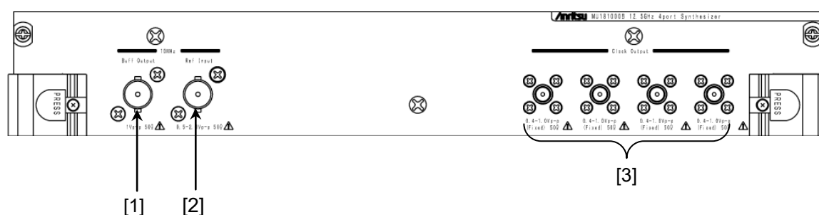
図3.1.1-2 MU181000B のパネル外観図
