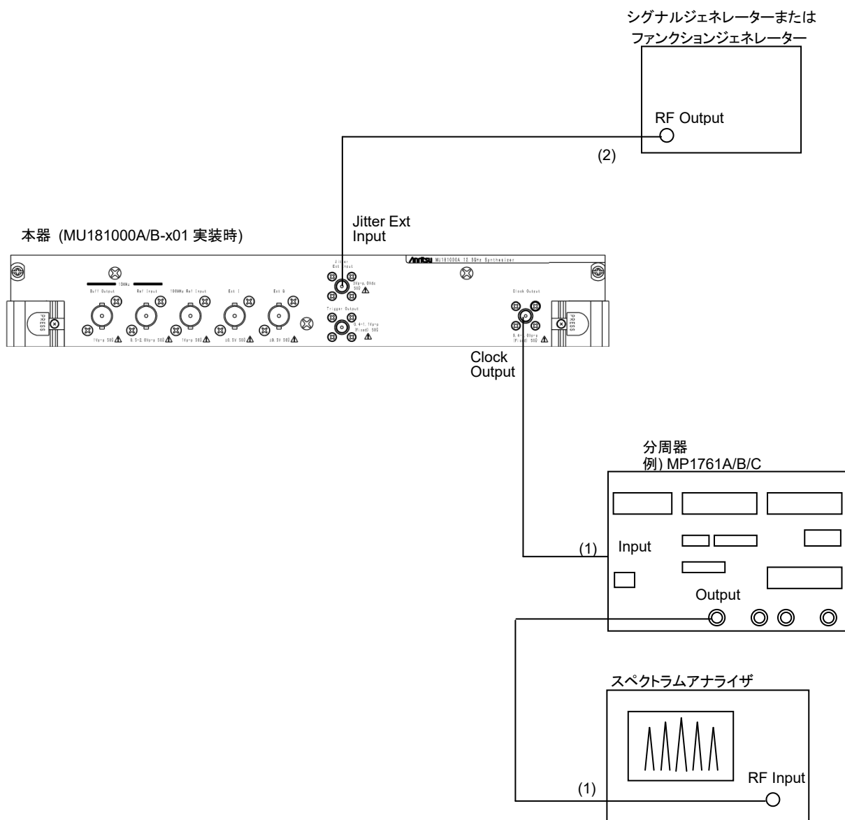
図6.3.4-2 0.4 Ulp-p 以上の正弦波ジッタ測定 of 接続図
