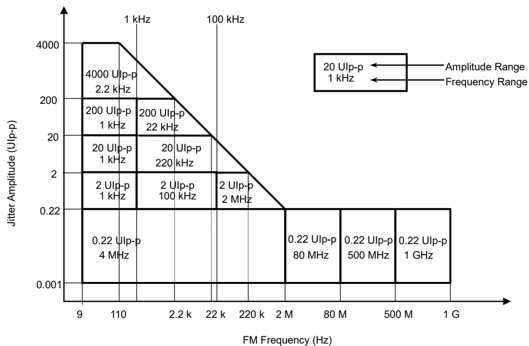
図4.2.2-6 3.2 \text{ GHz} < F_c \leq 6.4 \text{ GHz} 時の Range 選択
