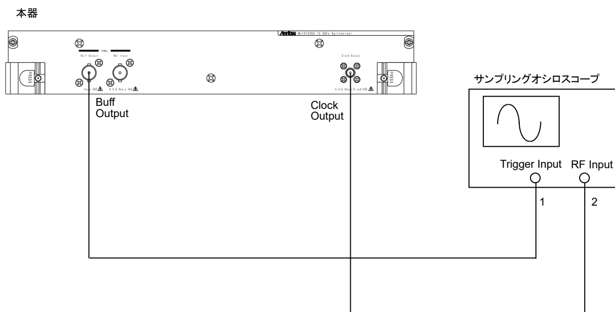
図6.3.1-1 波形測定の接続図
