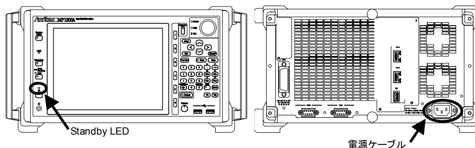
図2.1-1 MP1800A Standby LED と電源ケーブル
