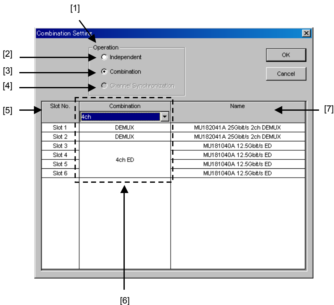
図5.3.3-1 Combination 設定画面
