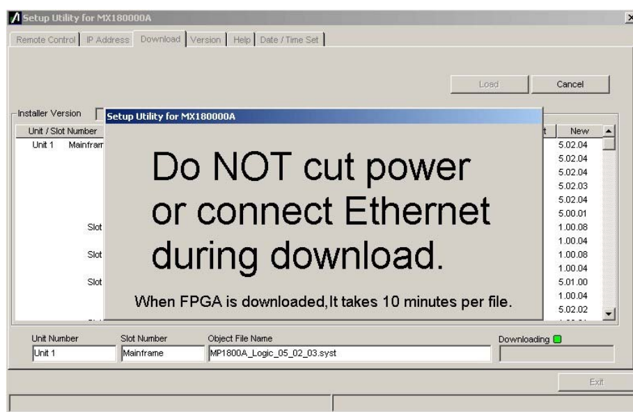
図6.5-2 ダウンロード画面 (ダウンロード中)
