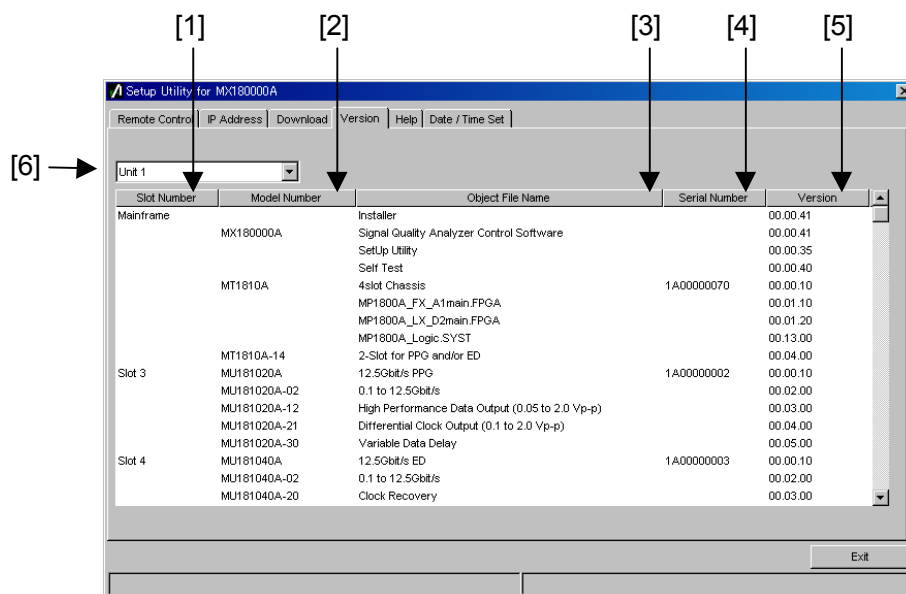
図6.6-1 ソフトウェアバージョン表示画面
