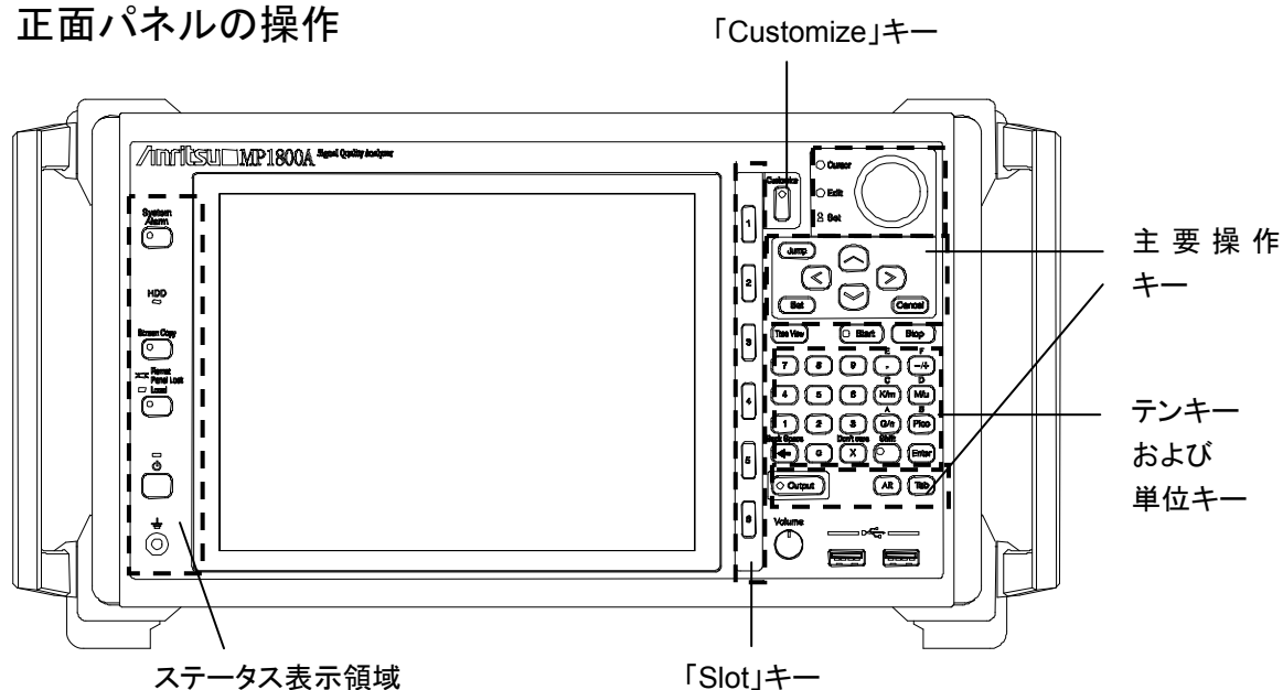
図4.2.1-1 正面パネル
