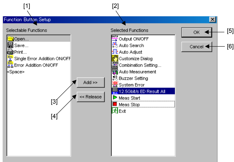
図5.4.1-1 Function Button Setup 画面
