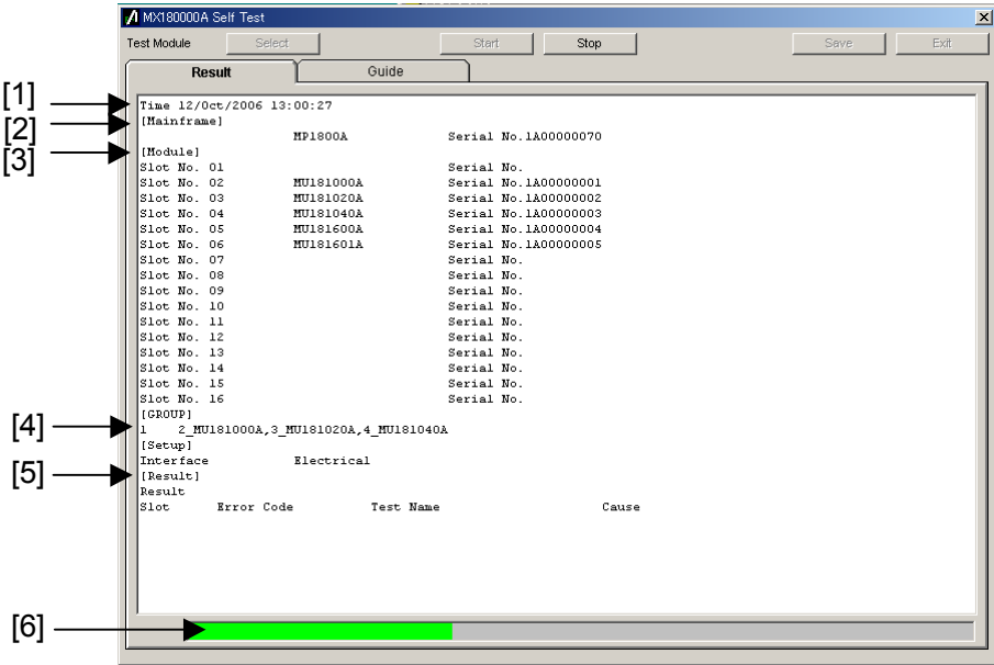
図7.3.4-1 テストモジュール結果表示画面
