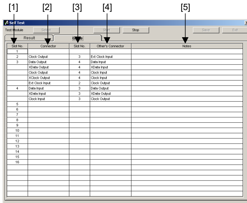
図7.3.3-1 接続ガイドタブ
