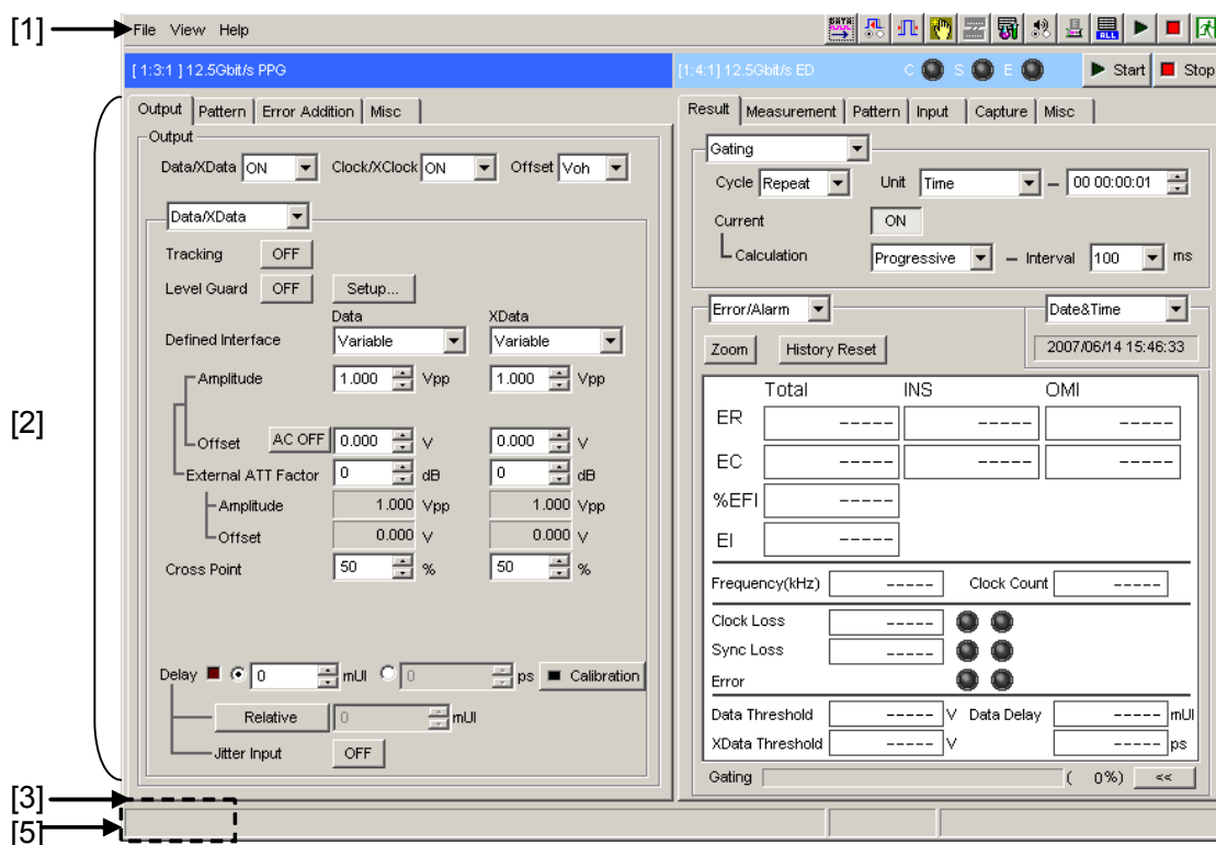
図3.1-1 Main Application 画面の構成 1
