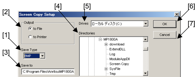
図5.2.5-1 Screen Copy Setup 画面
