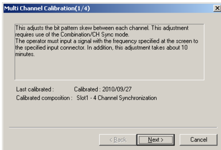
図5.2.10-1 Multi Channel Calibration 画面
