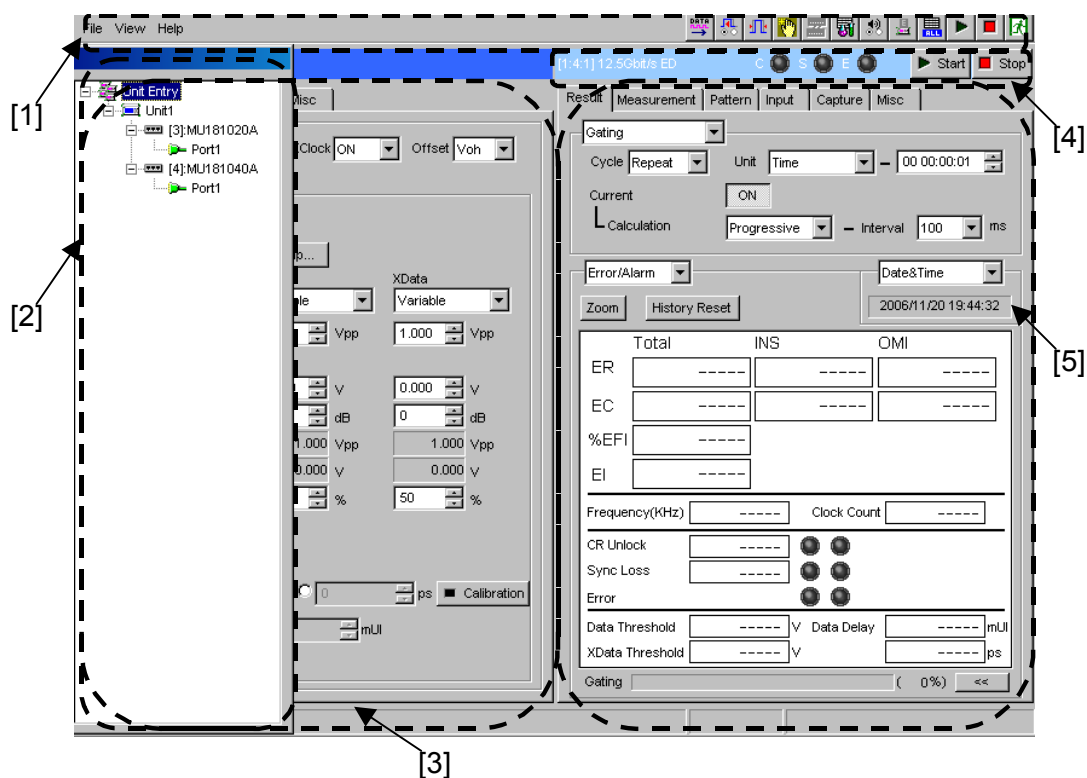
図4.2.2.1-1 フォーム間フォーカス移動
