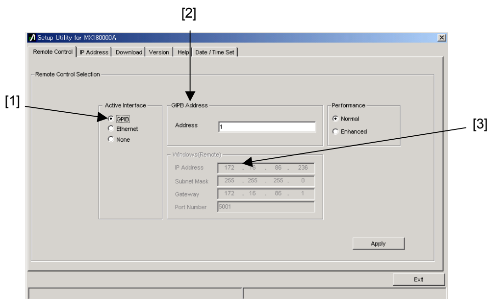
図6.3-1 リモートコントロール設定画面
