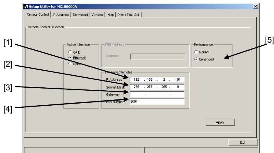
図6.3.2-1 Ethernet の設定画面
