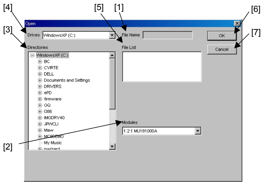
図5.2.3-1 Open 画面
