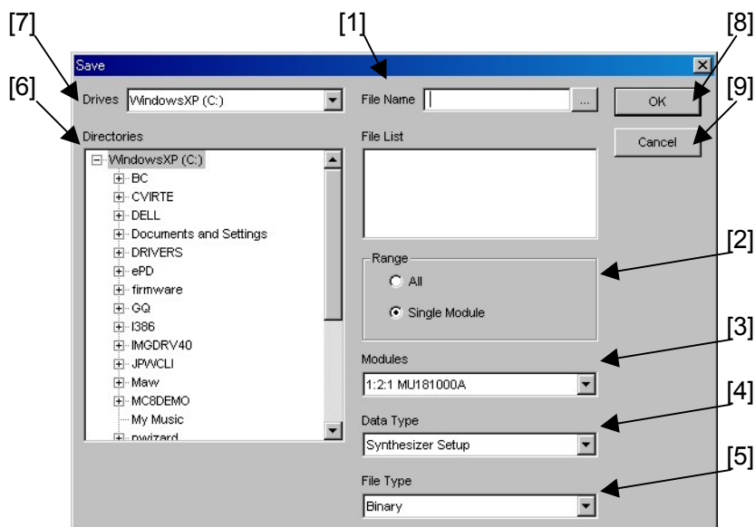
図5.2.4-1 Save 画面
