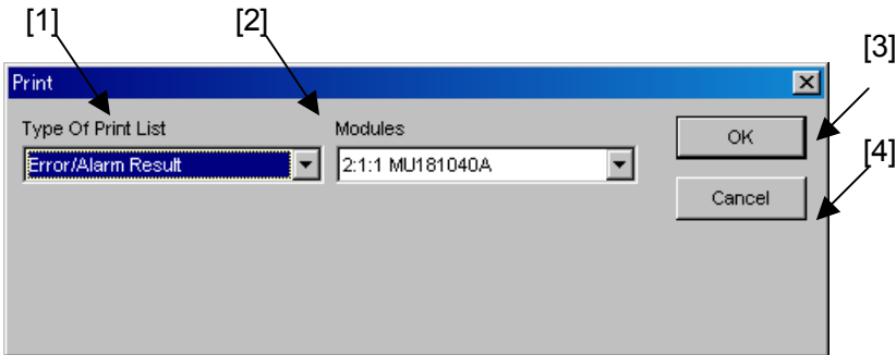
図5.2.6-1 Print 画面
