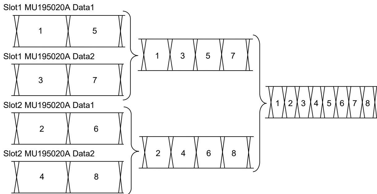
図 5.8.1-2 64G x 2ch Combination パターン生成 (MU195020A 2 モジュール)
