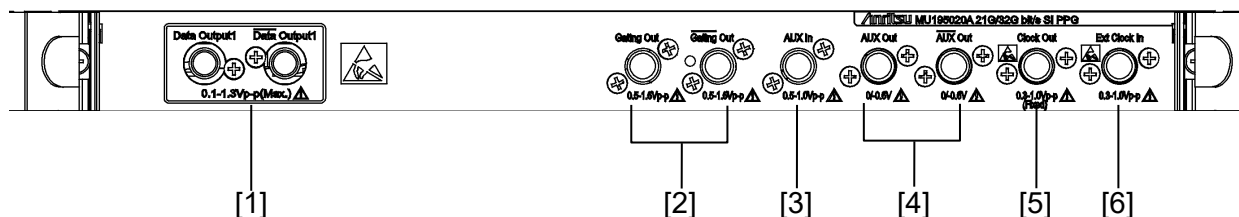
図3.1.1-1 パネル外観図 (MU195020A-x10)
