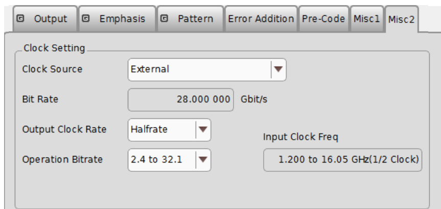
図 5.7.1.4-1 Clock Source 設定 (外部クロック供給源使用時)
