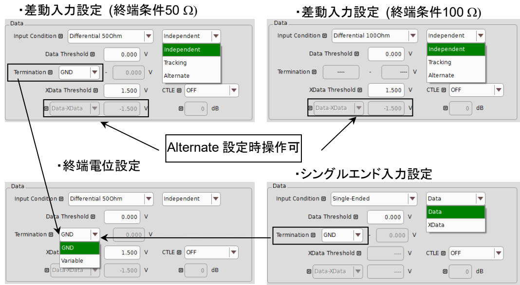
図 5.14.1-2 Data 入力条件設定
