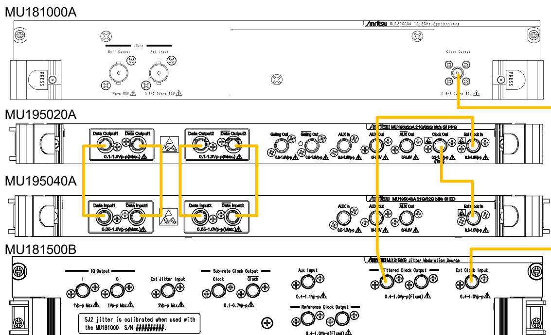
図3.2.3-1 ジッタを付加する場合の接続例
