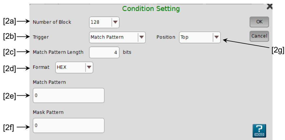
図 5.15.1-4 Condition Setting ダイアログボックス
