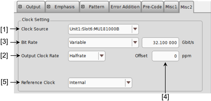
図 5.7.1-1 クロック設定項目画面 (MU181000B の場合)
