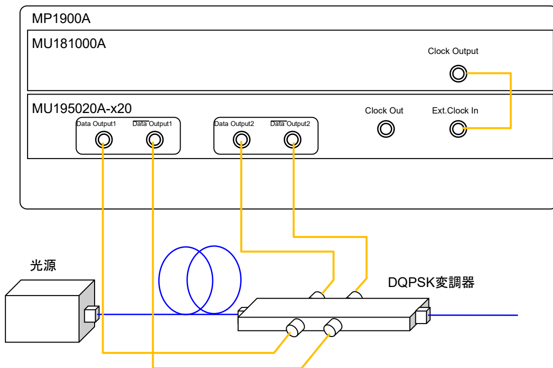
図6.2-1 56 Gbit/s DQPSK 信号発生の接続図
