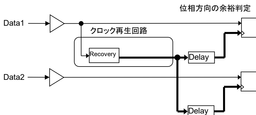
図 5.14.1-5 Recovered Clock 回路
