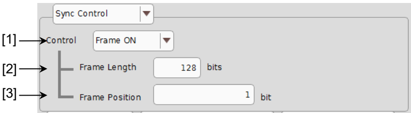
図 5.11.5-1 Sync Control 設定項目
