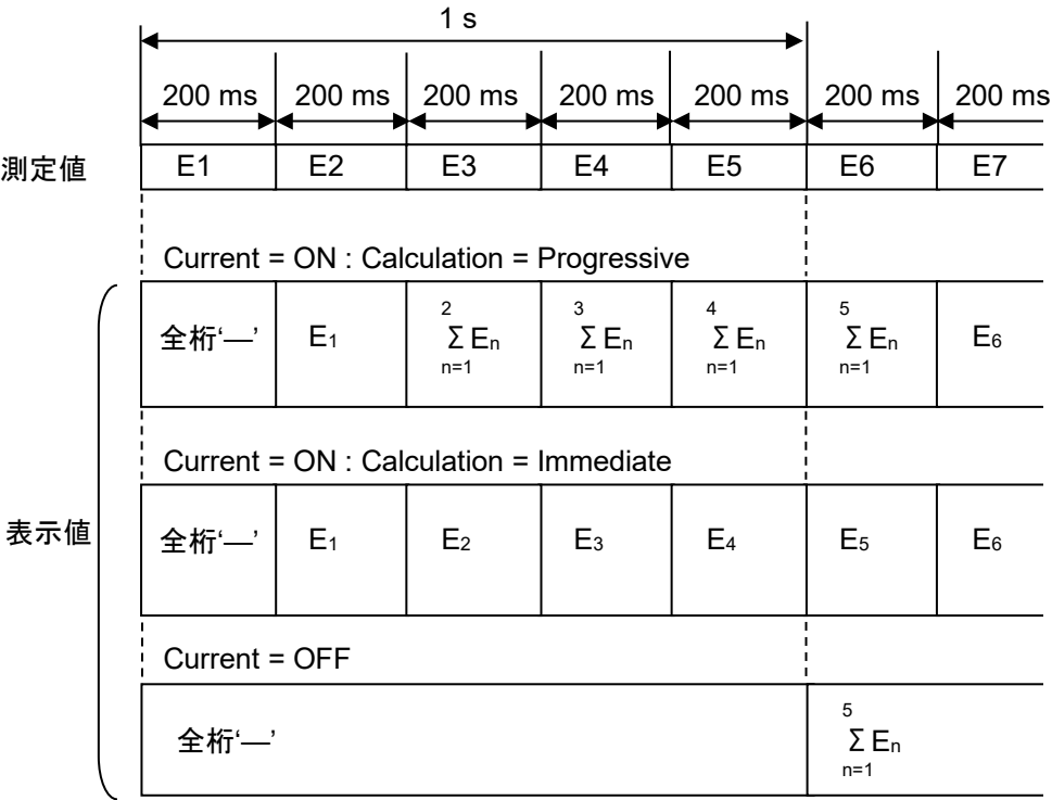
図 5.11.2-4 測定結果表示の関係
