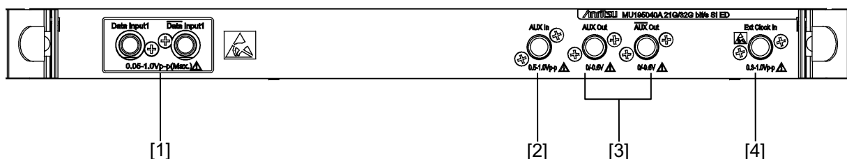
図3.1.2-1 パネル外観図 (MU195040A-x10)
