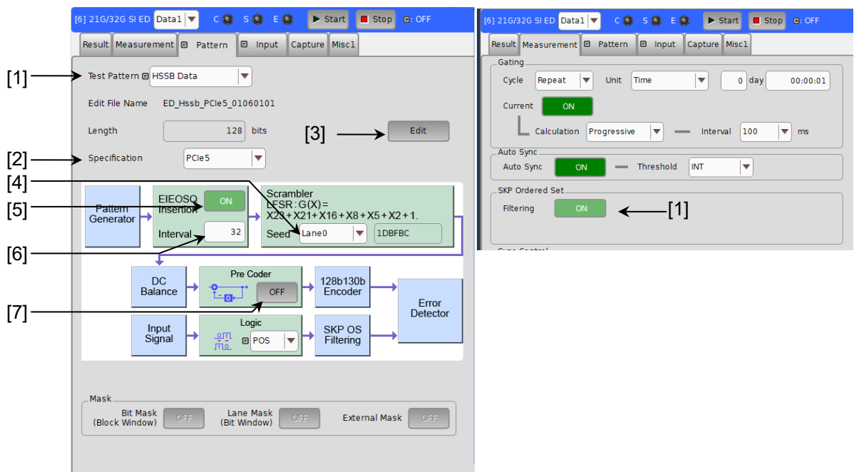
図 5.13.2-1 HSSB Data の設定
