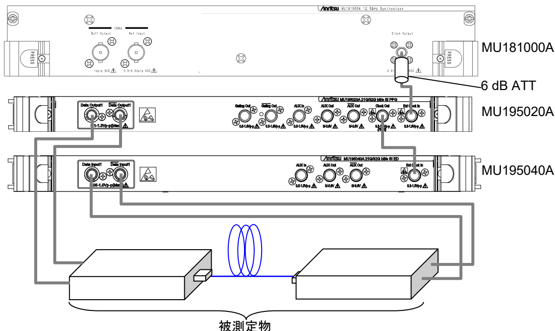
図3.2.1-1 モジュール間接続例
