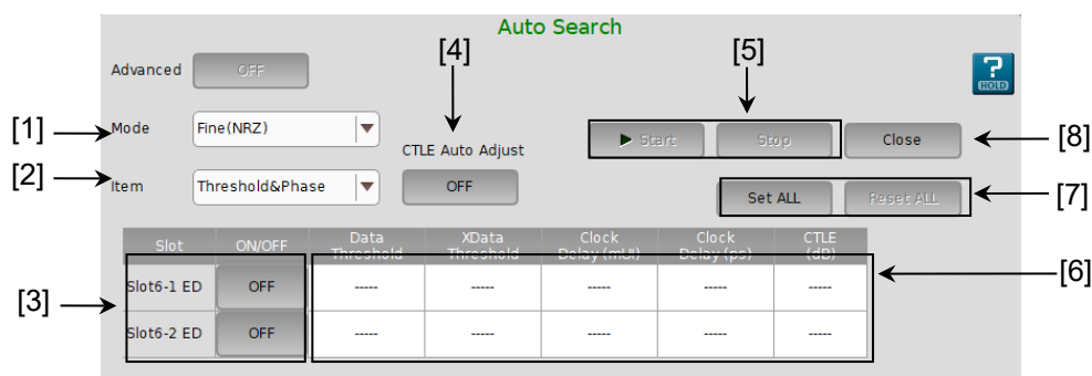
図 5.17.1-1 Auto Search ダイアログボックス
