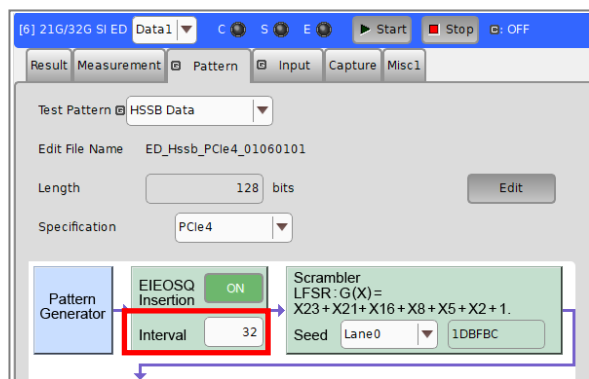
図 5.13.4-3 MU195040A の EIEOSQ Interval 設定
