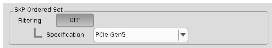
図 5.12.3-1 SKP Ordered Set 設定項目
