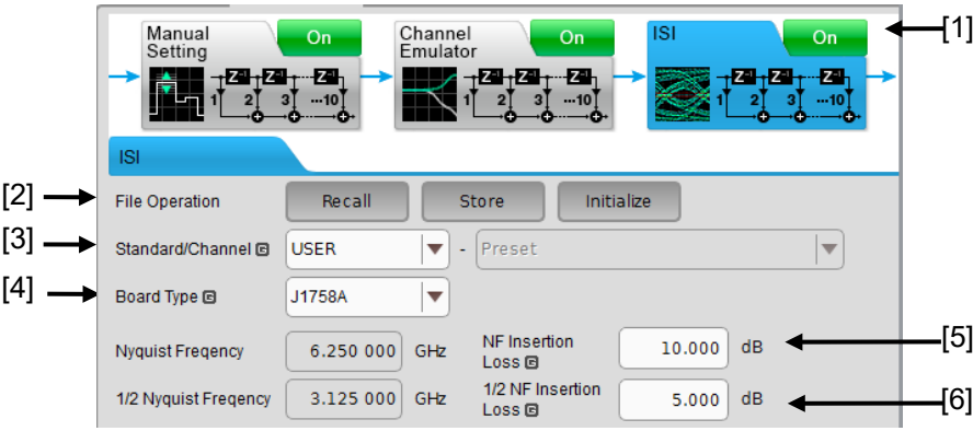
図 5.2.5-1 Emphasis タブ ISI 設定部
