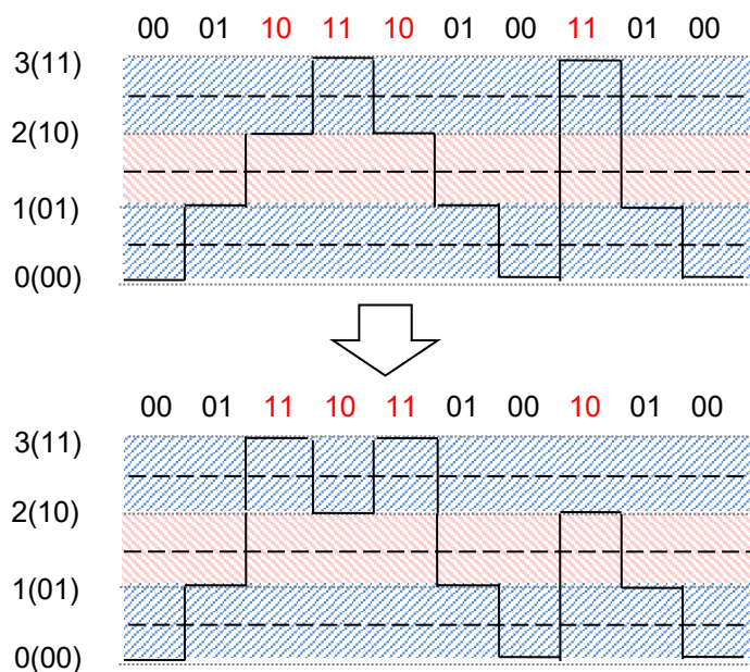
図 5.3.6-4 Gray Coding PAM4 パターン波形
