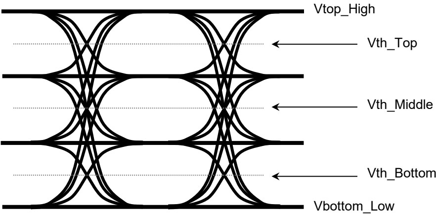
図 5.17.1-3 PAM4 波形の Vth イメージ
