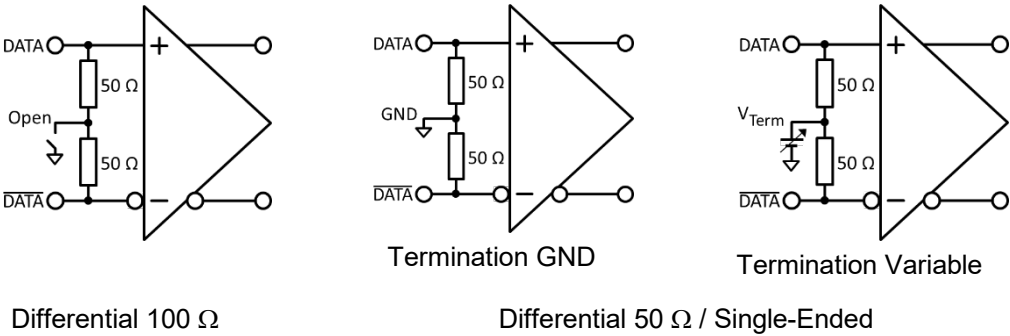
図 5.14.1-3 Data Termination 設定による終端方法の違い
