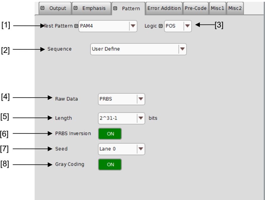
図 5.3.6-2 Test Pattern (PAM4-PRBS) 設定項目画面
