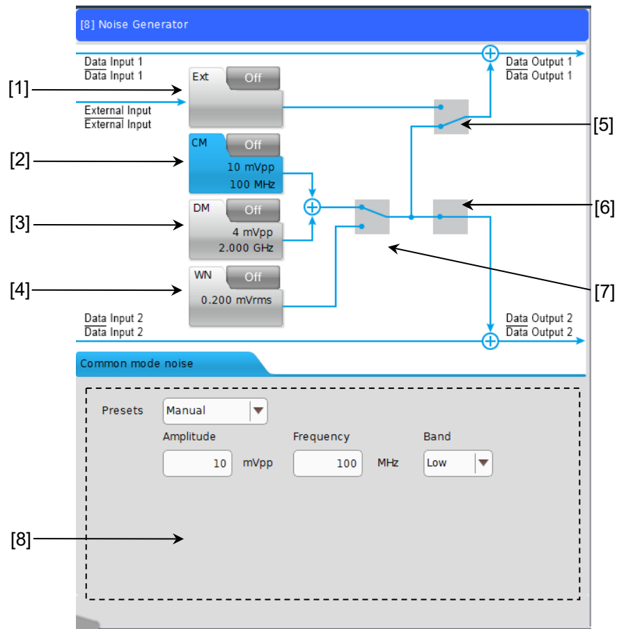
図 5.20.1-1 MU195050A 操作画面
