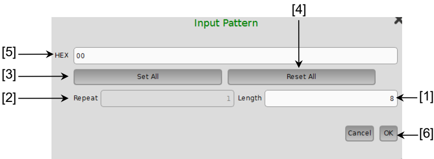
図 5.3.7.6-1 Input Pattern ダイアログボックス
