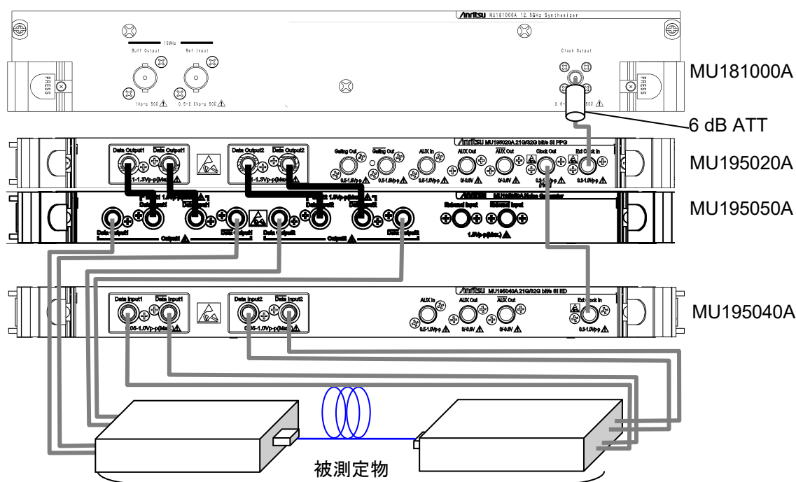
図3.2.2-1 モジュール間接続例
