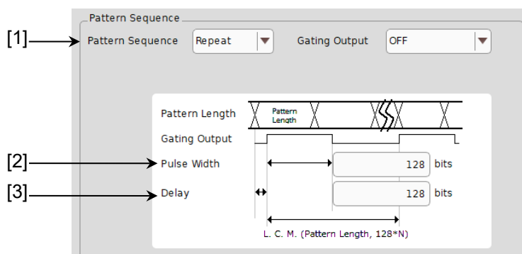
図 5.6.1.1-1 Pattern Sequence (Repeat) 設定項目画面
