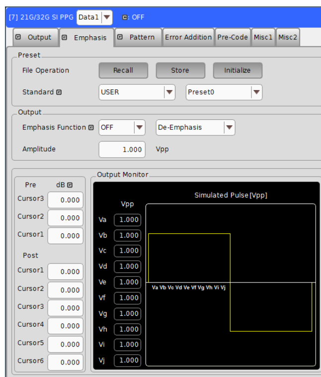
図 5.2-1 Emphasis タブ (MX190000A Version 2.0.0 以前)
