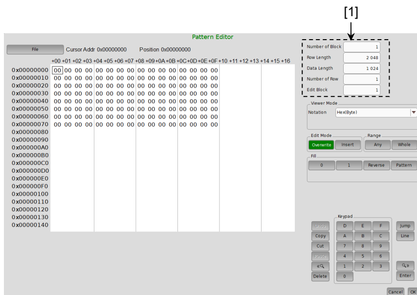
図 5.3.7.3-1 Pattern Editor ダイアログボックス-Mixed
