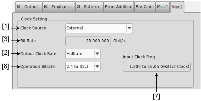
図 5.7.1-2 クロック設定項目画面 (External の場合)
