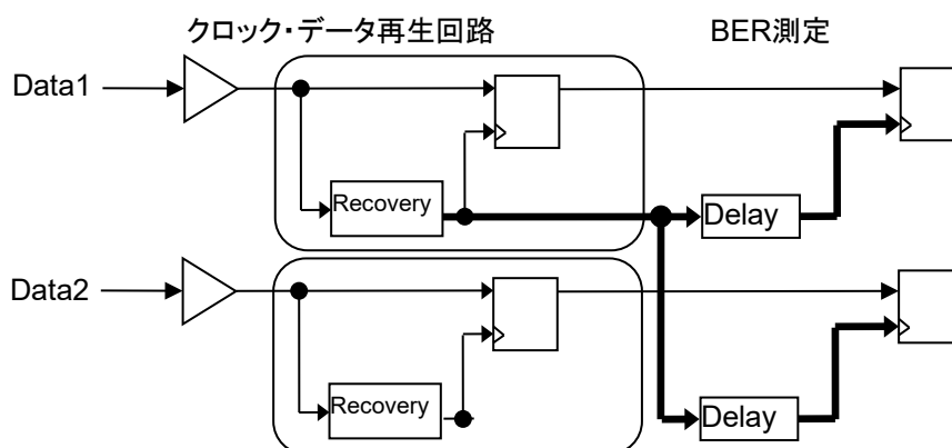
図 5.14.1-6 Clock and Data Recovery 回路
