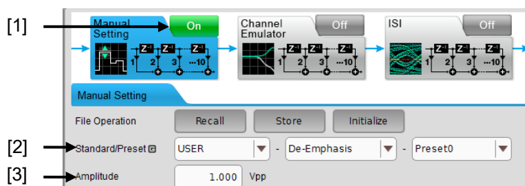
図 5.2.2-2 Emphasis タブ 機能選択部 (MX190000A Version 2.0.0 以降)
