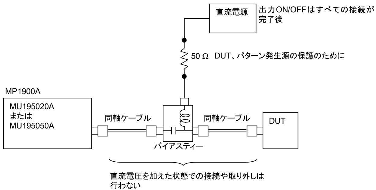
図2.3-1 バイアスティーの接続例
