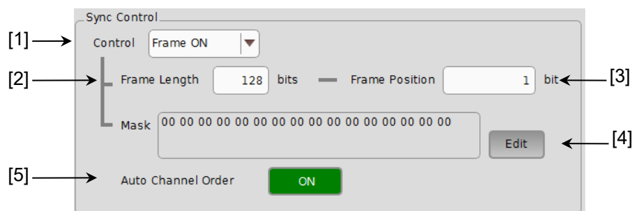
図 5.12.4-1 同期方式の設定
