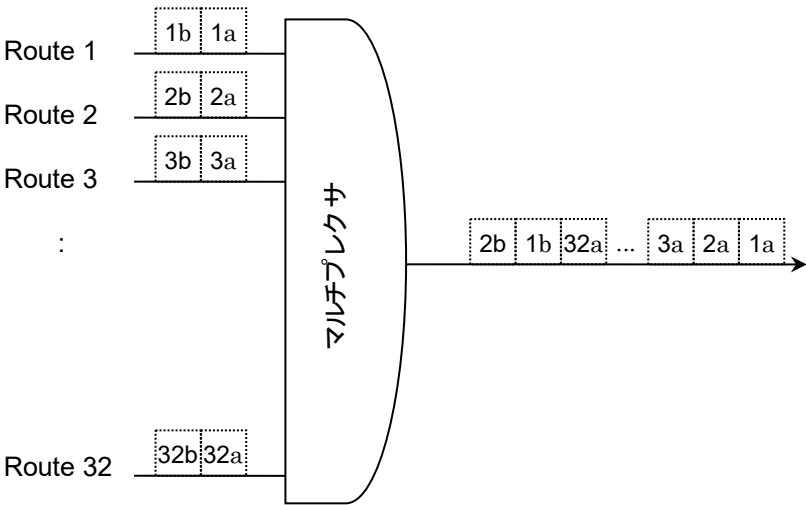
図 5.4-2 試験パターンのパラレル-シリアル変換
