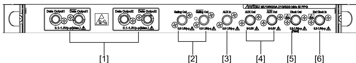
図3.1.1-2 パネル外観図 (MU195020A-x20)
