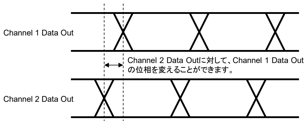
図 5.1.2-3 Combination 時の Delay 設定
