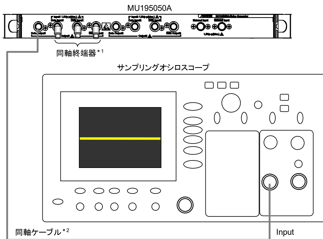
図8.3.6-2 ホワイトノイズ試験の接続図
