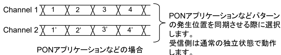
図 5.8.2-1 Channel Synchronization パターン生成
