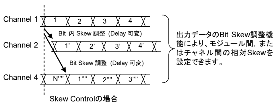
図 5.8.2-2 Channel Synchronization 時の Skew 調整
