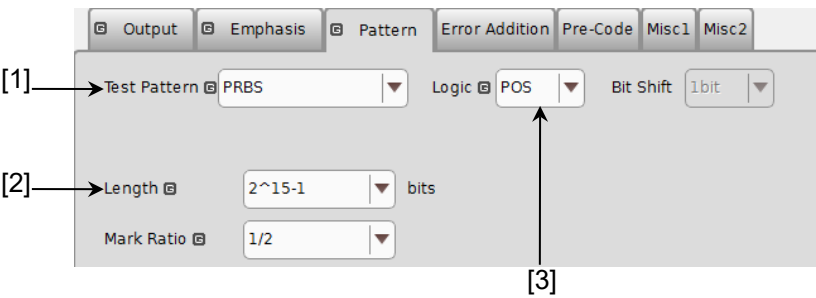
図 5.3.2-1 Test Pattern (PRBS) 設定項目画面
