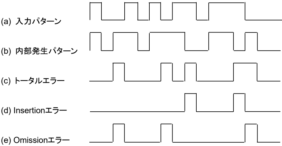
図 5.11.3-2 Error Detection (トータルエラー、Insertion エラー、Omission エラー)
