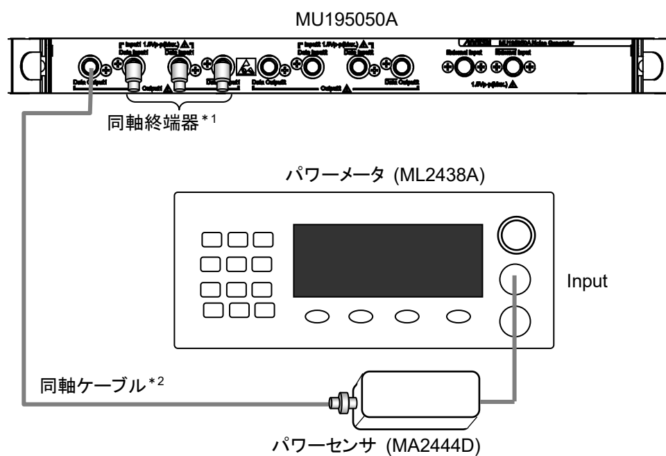
図8.3.6-1 CMI/DMI 試験の接続図
