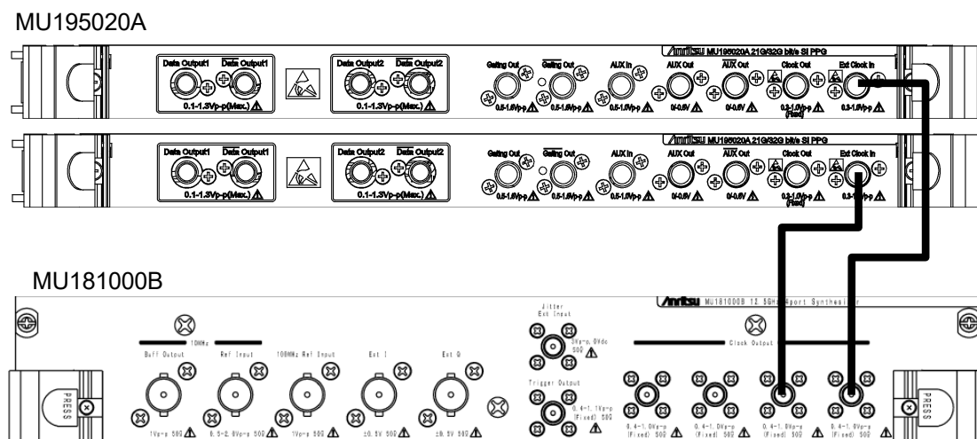
図3.2.4-1 PPG の Multi Channel 同期する場合の接続例
