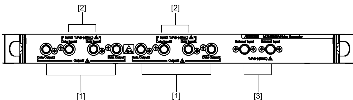
図3.1.3-1 パネル外観図 (MU195050A)
