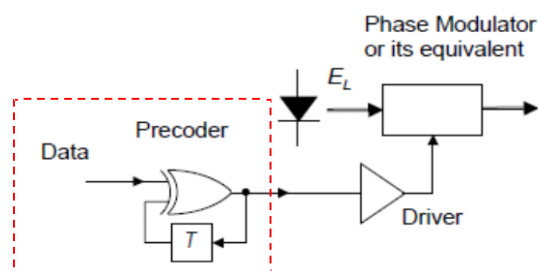
図 5.5-1 Pre-Code 論理図 (DQPSK)
