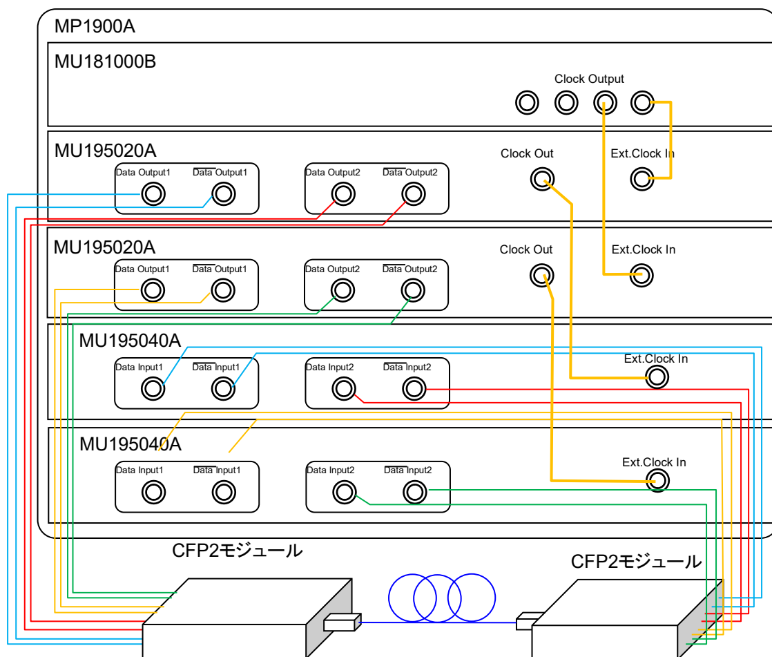
図6.1-1 CFP2 モジュール評価接続図
