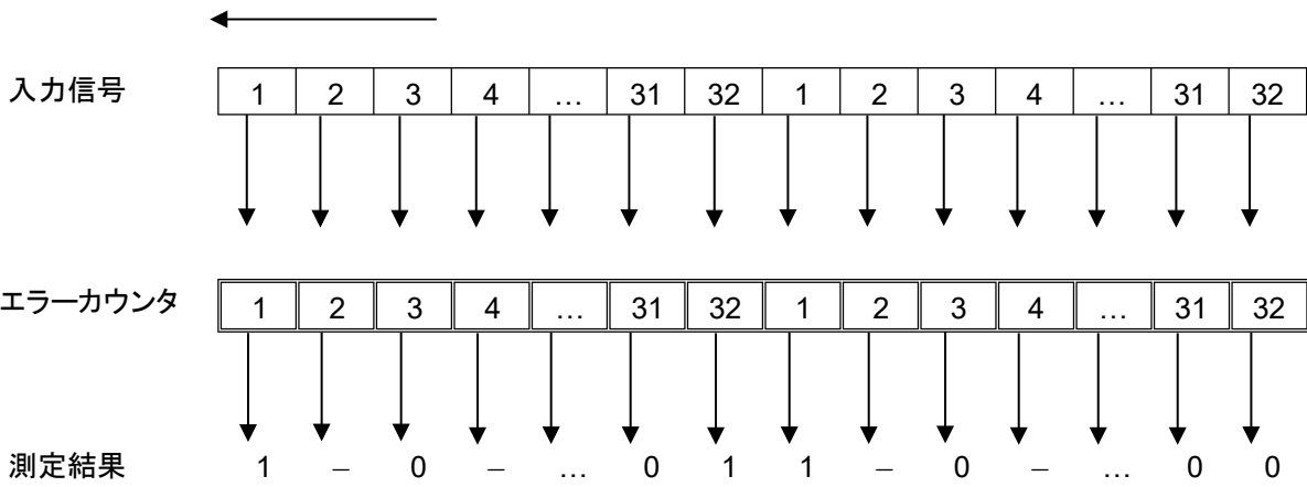
図 5.13.1-2 Bit Window 機能
