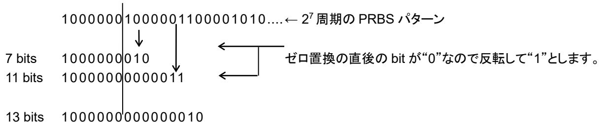
図A.2-1 ゼロ置換パターン
