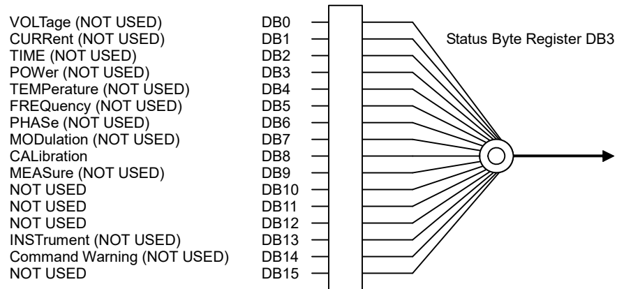
図 4.1.1-1 QUEStionable ステータスレジスタ
