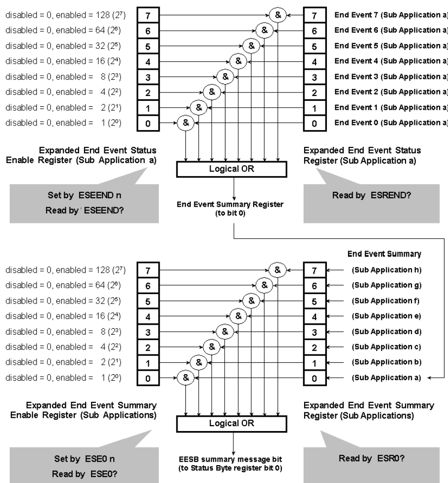
図1.9.15-1 拡張終了イベントステータスレジスタ (Sub Application a の例)
