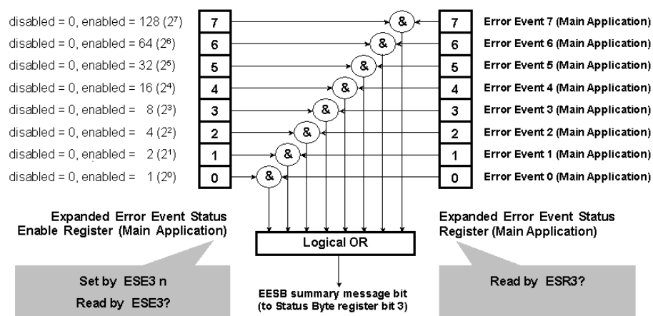
図1.9.12-1 拡張エラーイベントステータスレジスタ (Main Application)
