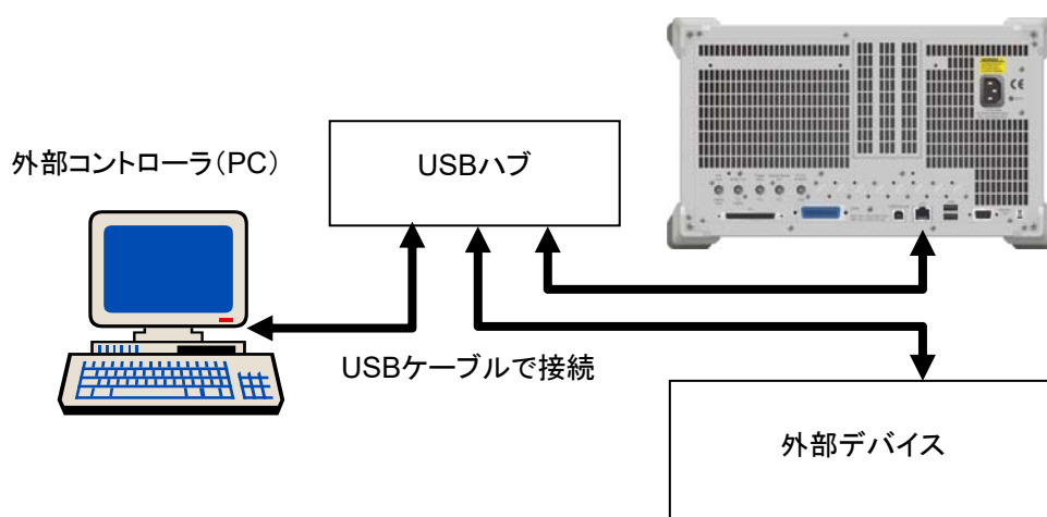
図1.2.3-2 本器と複数の外部機器の接続例
