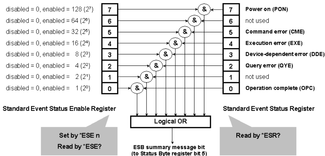
図1.9.7-1 標準イベントステータスレジスタ
