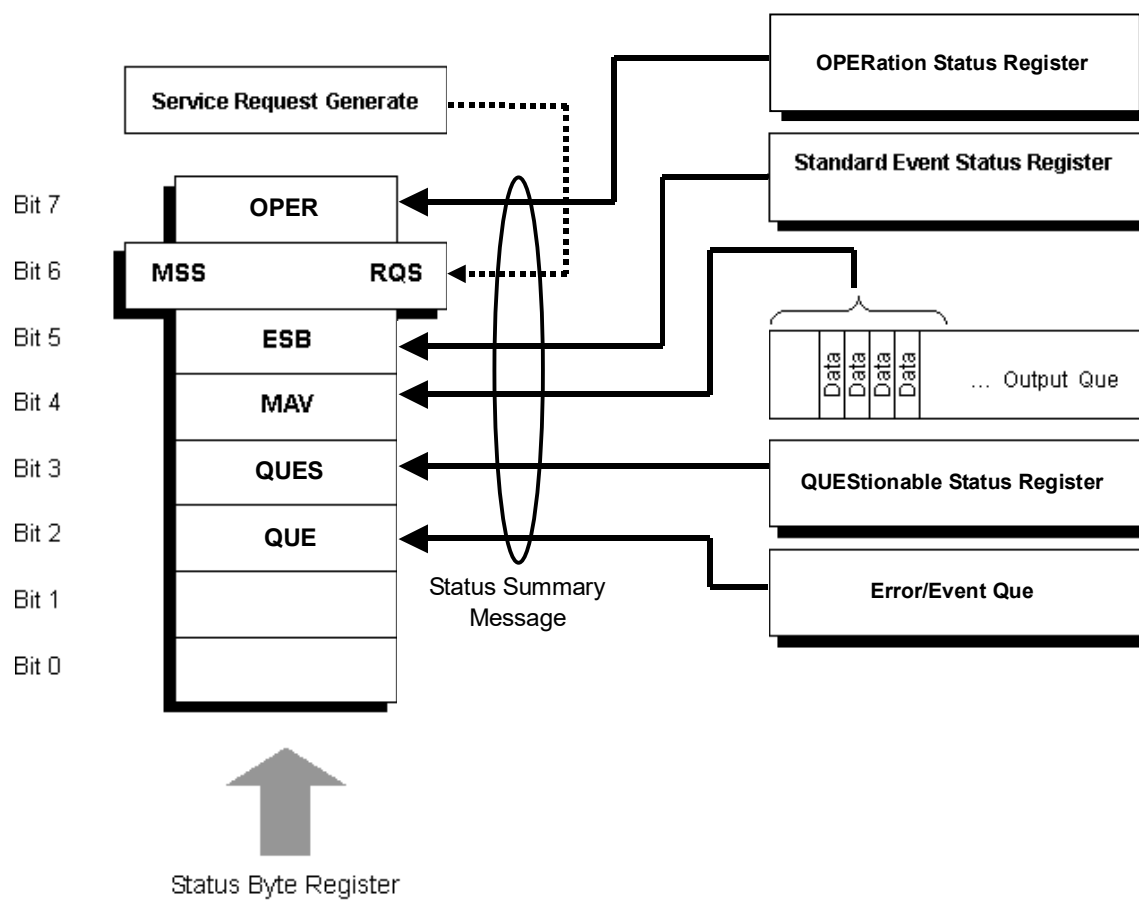
図1.9.3-1 SCPI モード時のステータスバイトレジスタ
