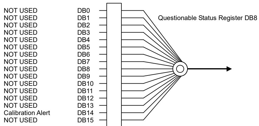
図 4.1.1-2 QUEStionable Calibration レジスタ
