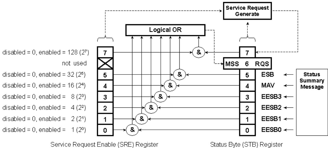
図1.9.6-1 サービスリクエスト (SRQ) のイネーブル操作
