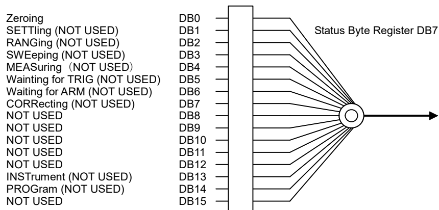
図 4.3.3-1 OPERation ステータスレジスタ
