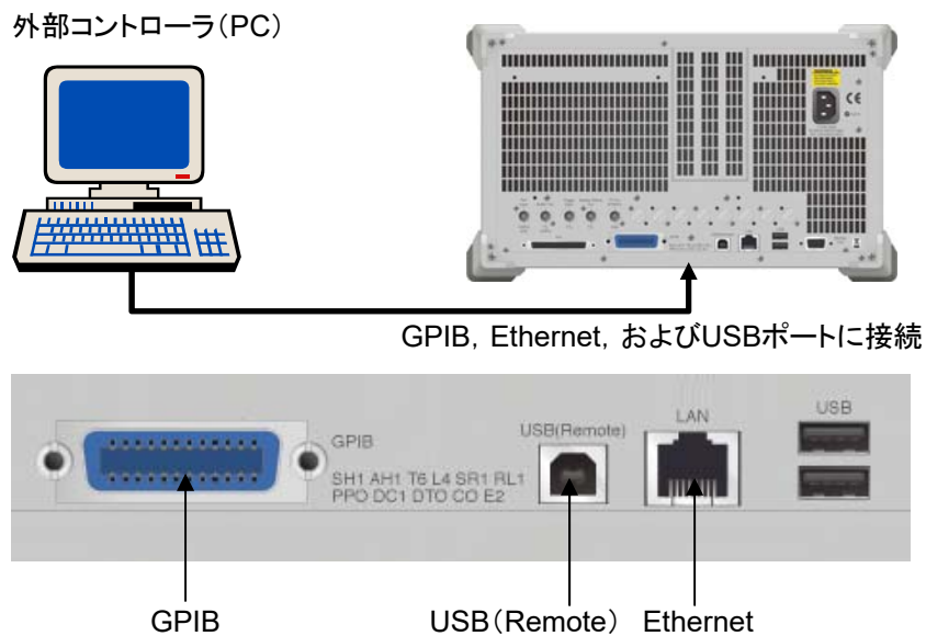
図1.2-1 外部コントローラ（PC）との接続ポート
