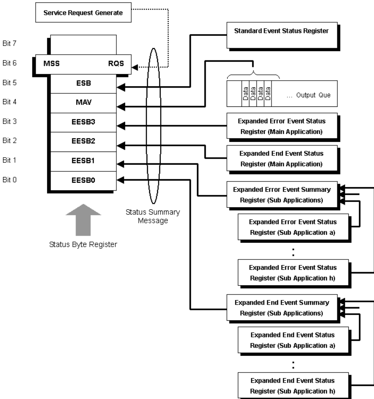
図1.9.4-1 Native モード時のステータスバイトレジスタ
