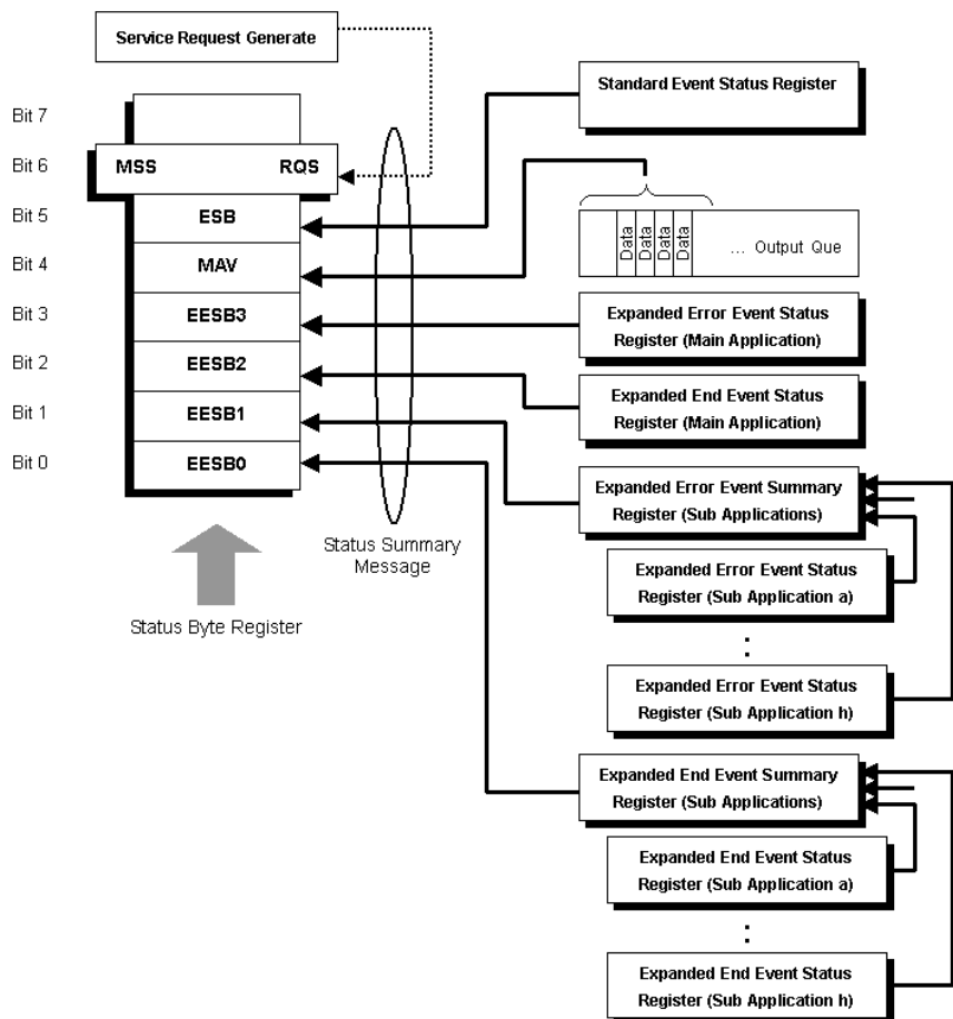
図1.9.11-1 拡張イベントステータスレジスタモデル
