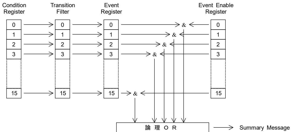
図1.9.9-1 SCPI 規定ステータスレジスタの構成図
