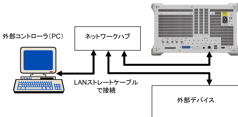
図1.2.2-2 本器と複数の外部機器の接続例
