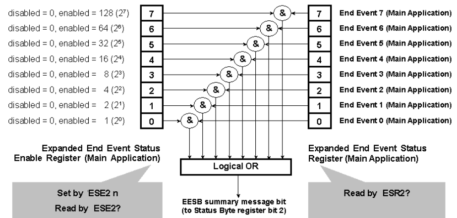
図1.9.13-1 拡張終了イベントステータスレジスタ (Main Application)
