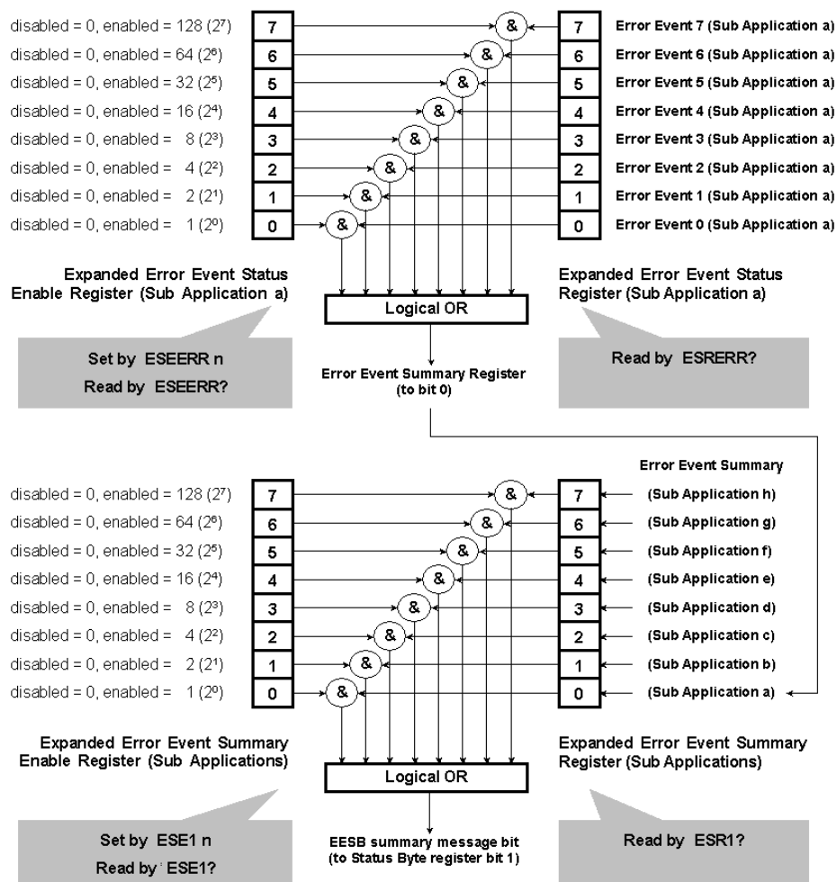
図1.9.14-1 拡張終了イベントステータスレジスタ (Sub Application a の例)
