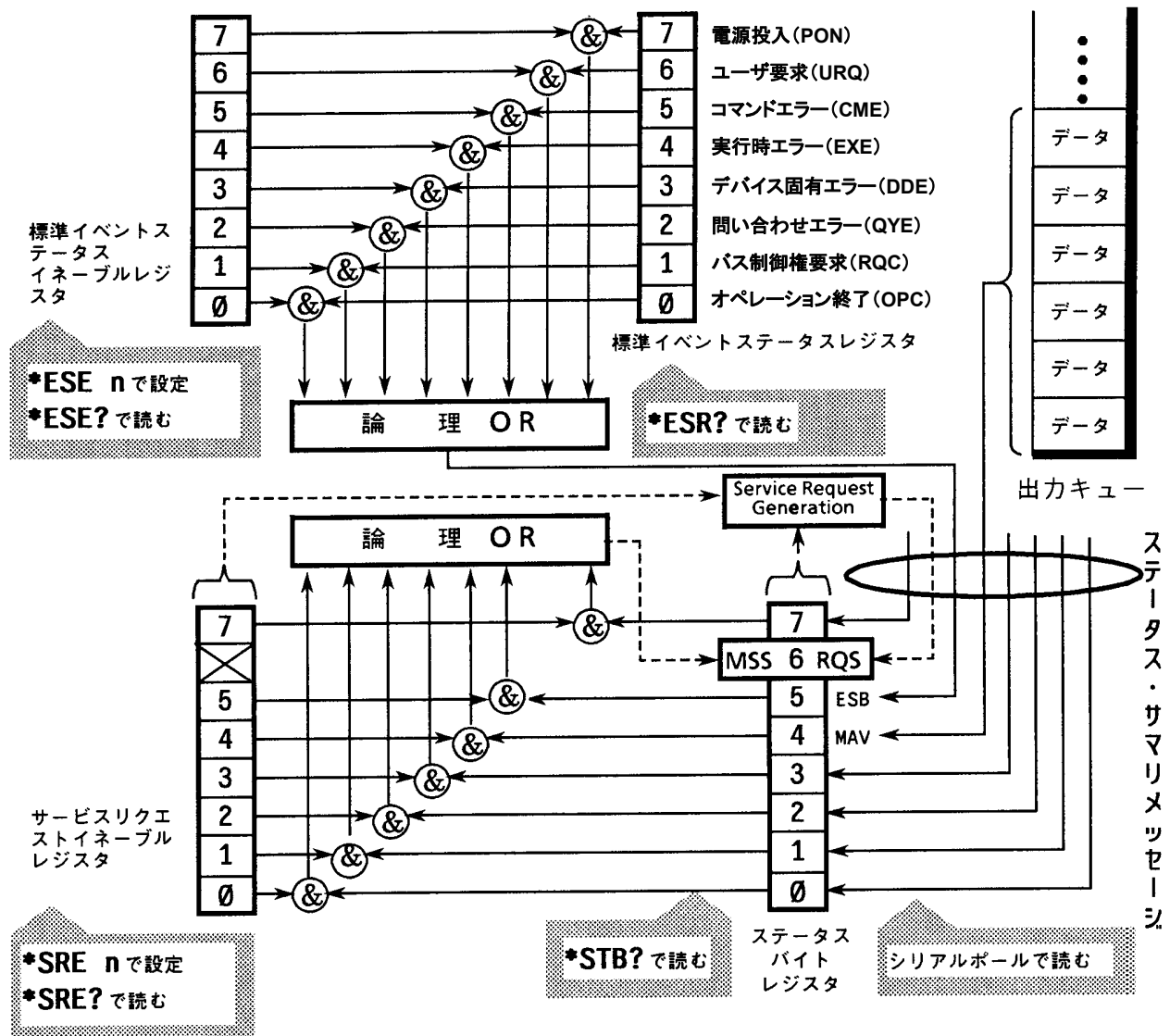
図1.9.1-1 IEEE488.2 標準ステータスのモデル
