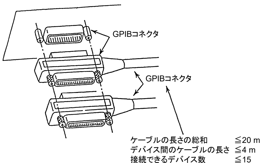
図1.2.1-1 GPIB ケーブルの接続
