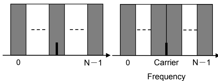
図3.7.8-1 セグメント配置と 1Segment Target の関係 (左: 奇数セグメント時, 右: 偶数セグメント時)
