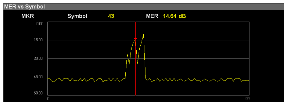
図3.6.7-1 MER vs Symbol グラフ
