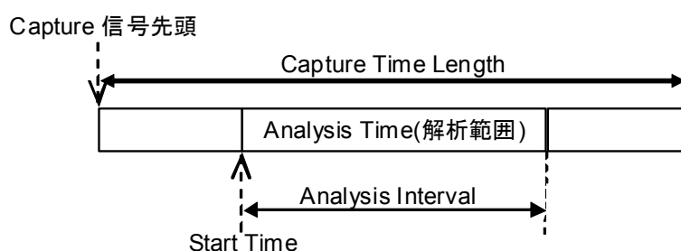
図3.5.1.1-1 Analysis Time と Capture Time のイメージ
