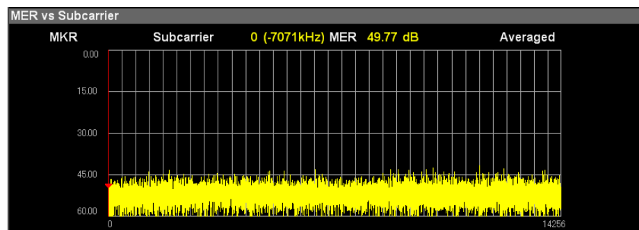
図3.6.6-1 MER vs Subcarrier グラフ
