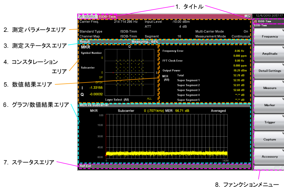
図3.1.1-1 画面の見方 (Modulation Analysis の例)
