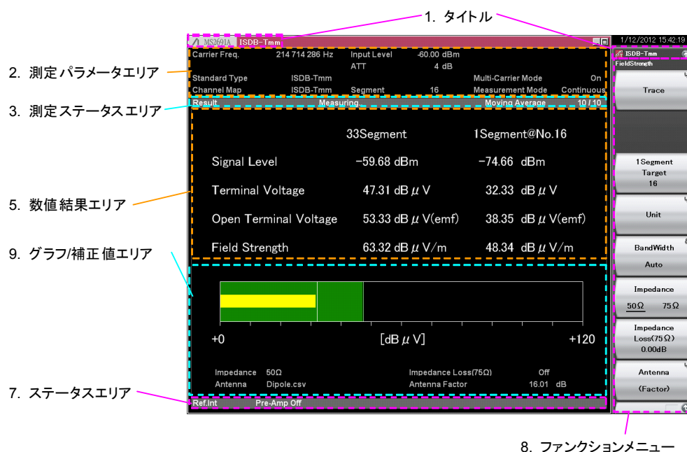
図3.1.1-2 画面の見方 (Field Strength の例)
