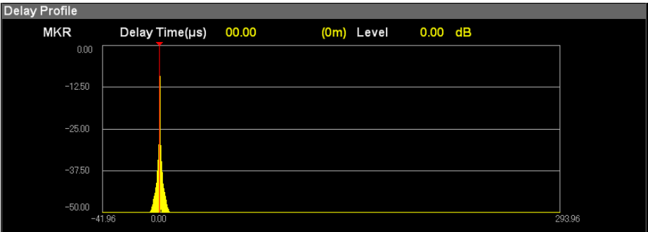
図3.6.9-1 Delay Profile グラフ
