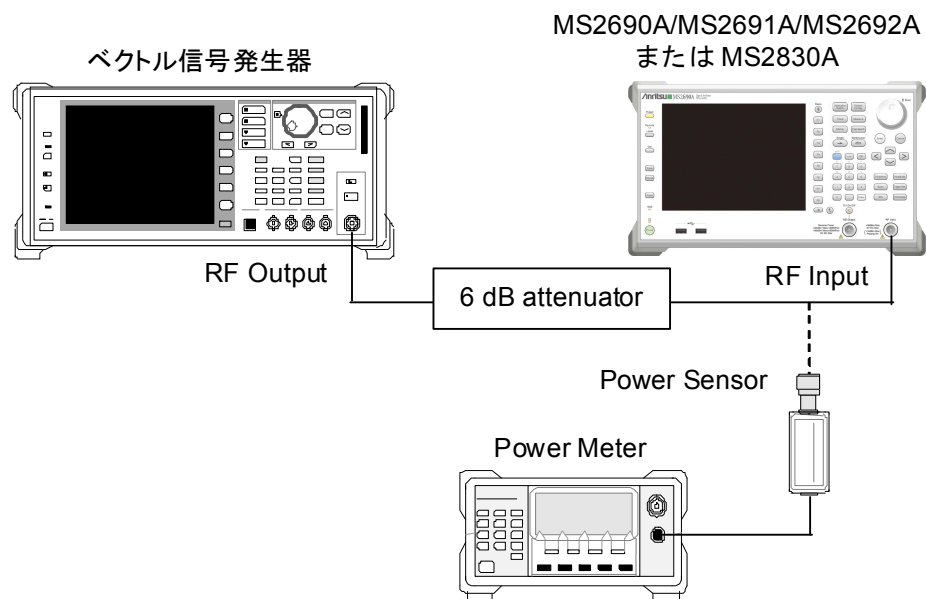
図 5.2.2-1 残留 MER 試験
