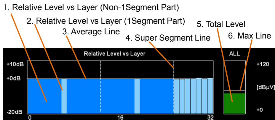
図3.7.7-1 レベルバーグラフ
