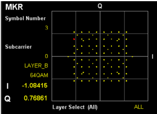
図3.6.5-1 コンスタレーショングラフ
