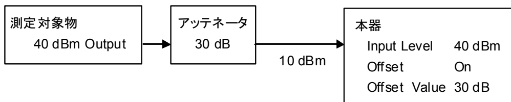
図3.2.2-1 Offset 設定例
