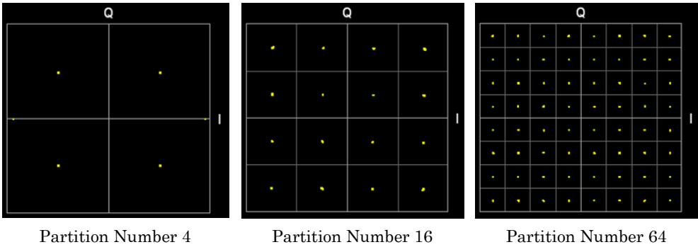
図3.6.5-2 コンスタレーショングラフ
