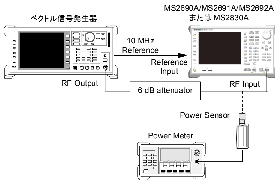
図 5.2.1-1 キャリア周波数確度試験
