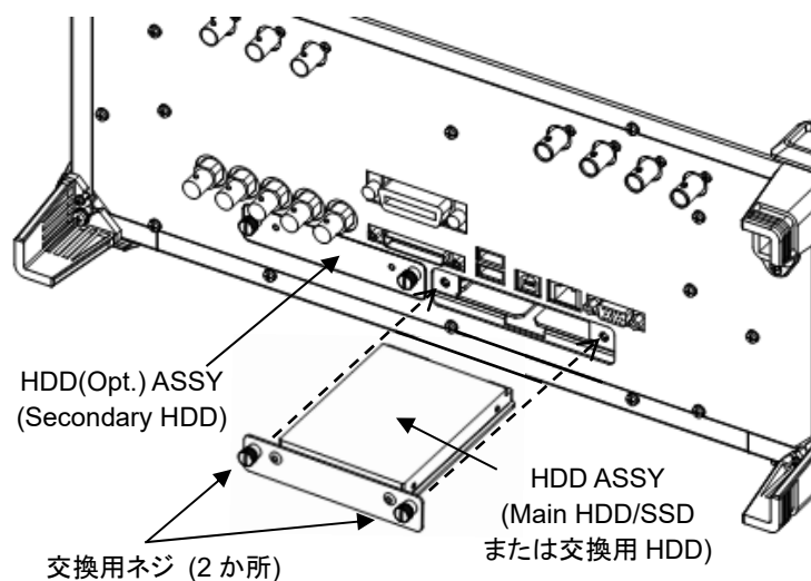
図9.4-1 HDD ASSY の交換
