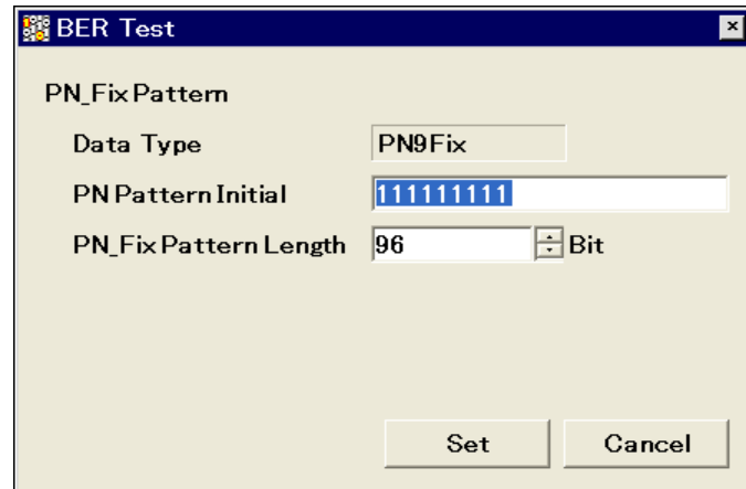
図8.8-2 PN Pattern Initial 設定
