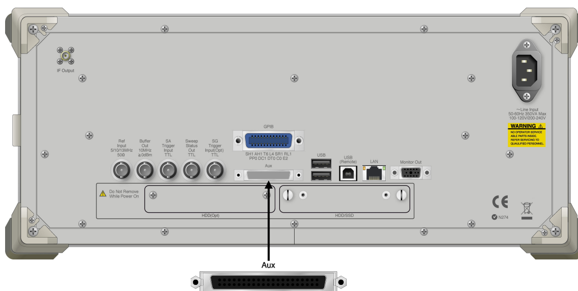
図8.4-1 入力コネクタ
