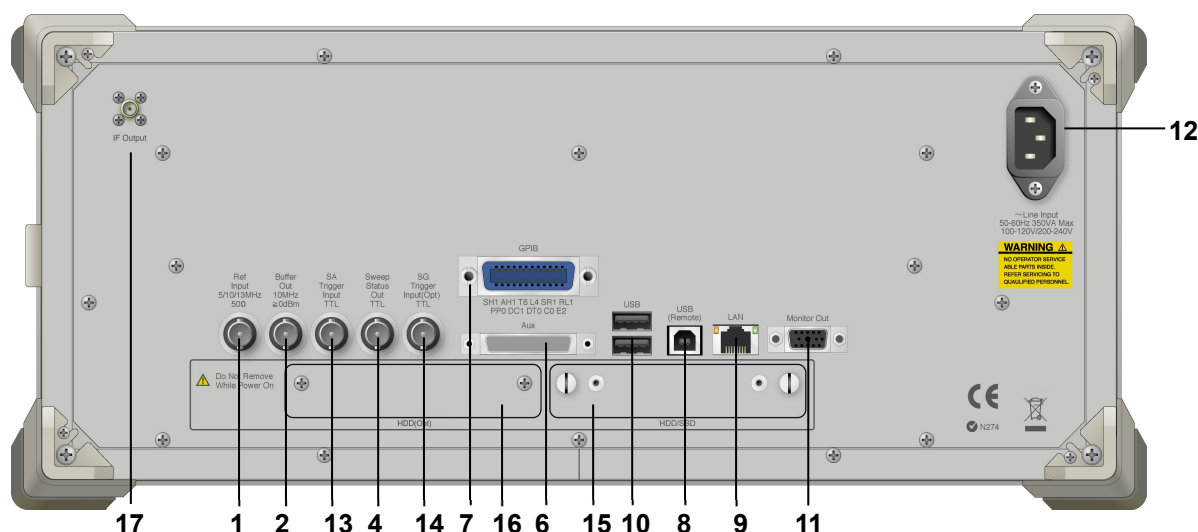
図 3.1.1-2 背面パネル
