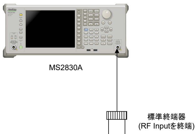
図6.2.5-1 表示平均雑音レベル
