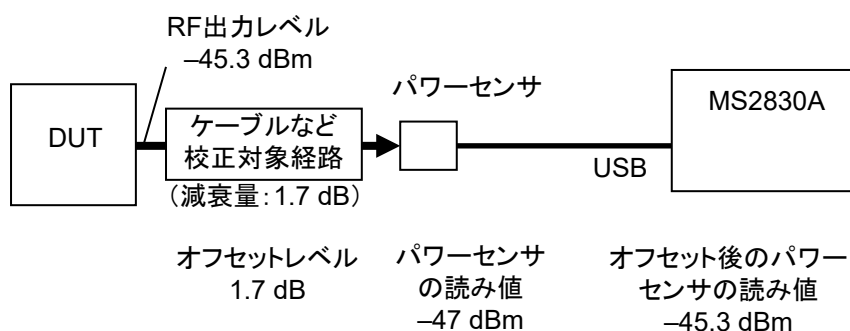
図7.3.2-1 オフセットレベルの概要
