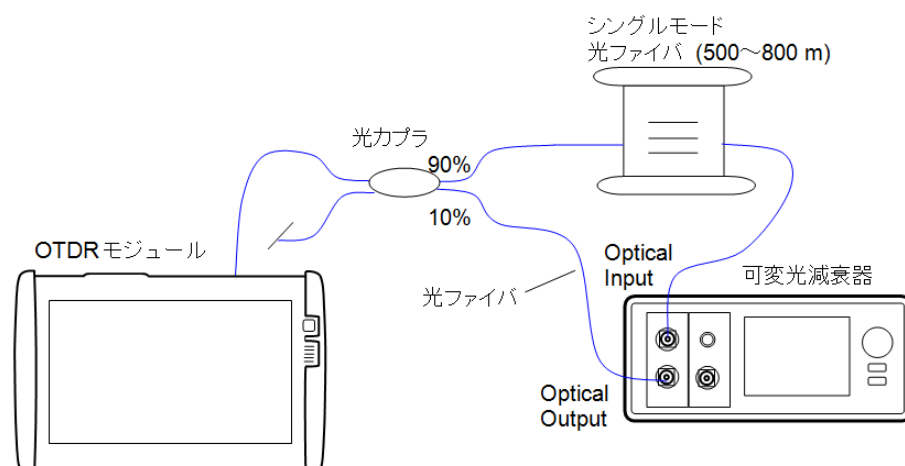
接続図
