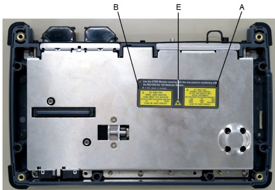
図7 ラベルの貼付位置 (MU100020A、MU100021A、MU100022A、MU100023Aの前面)
