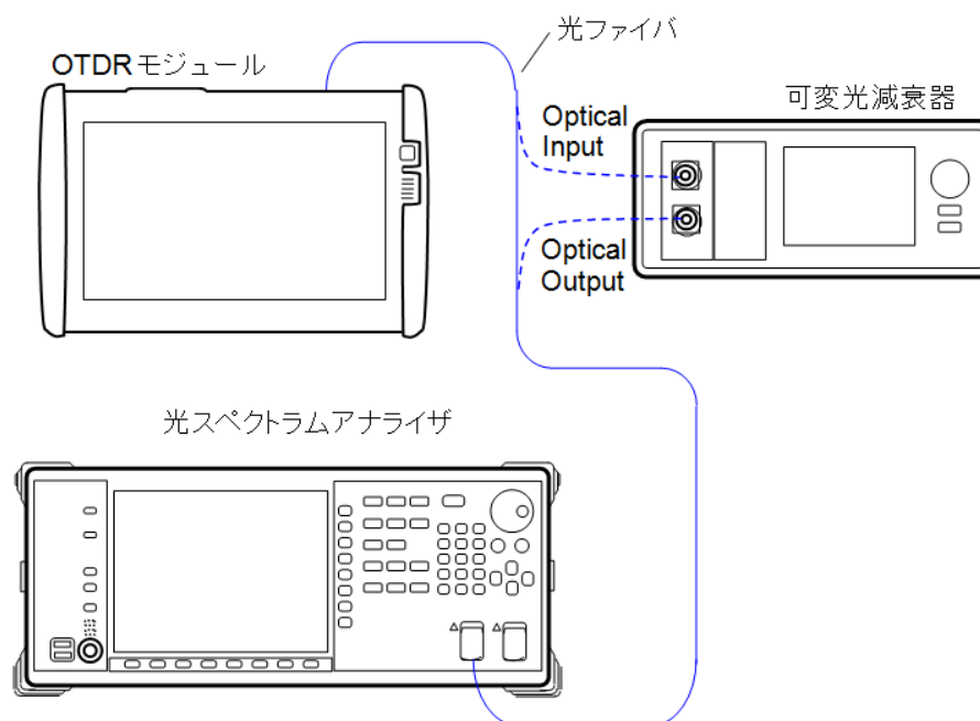
接続図
