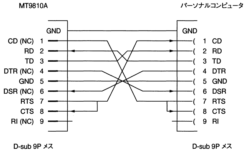
DOS/V パーソナルコンピュータとの接続図
