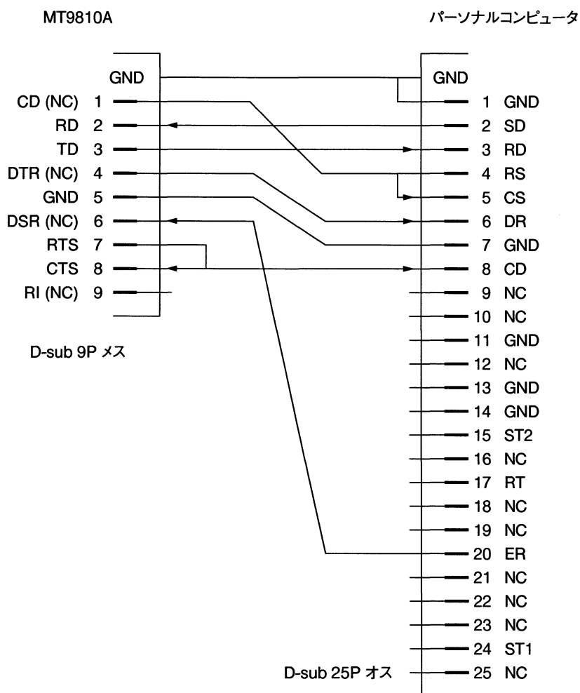
D-Sub25ピンのインタフェースを持つパーソナルコンピュータとの接続図
