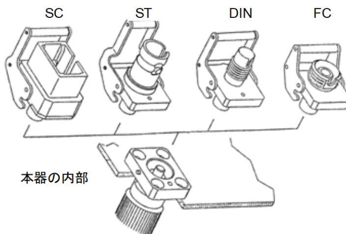
図2.9-2 光コネクタの種類
