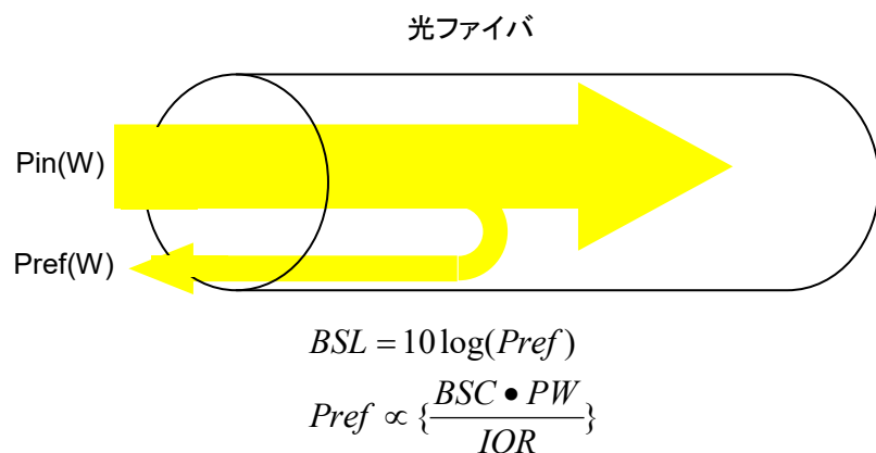
図1.3.1-1 後方散乱レベルの定義
