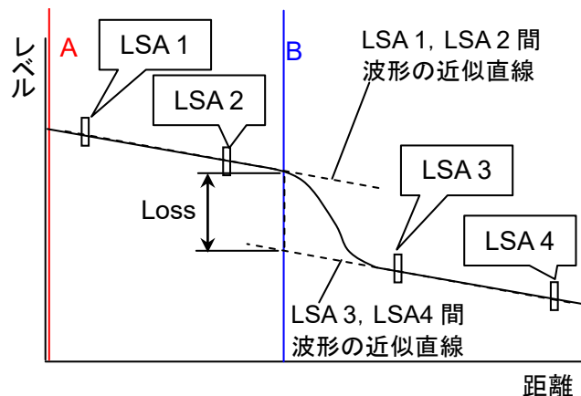
図4.10.1-3 接続損失 (LSA) の測定方法
