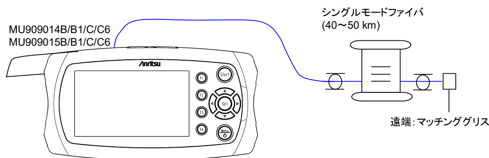
図11.1.4-3 ダイナミックレンジ測定のための接続図 (MU909014B/B1/C/C6、MU909015B/B1/C/C6)
