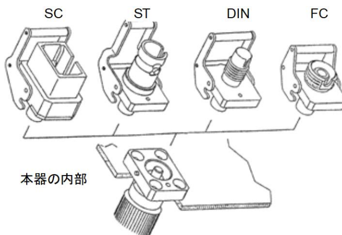
図2.9-2 光コネクタの種類
