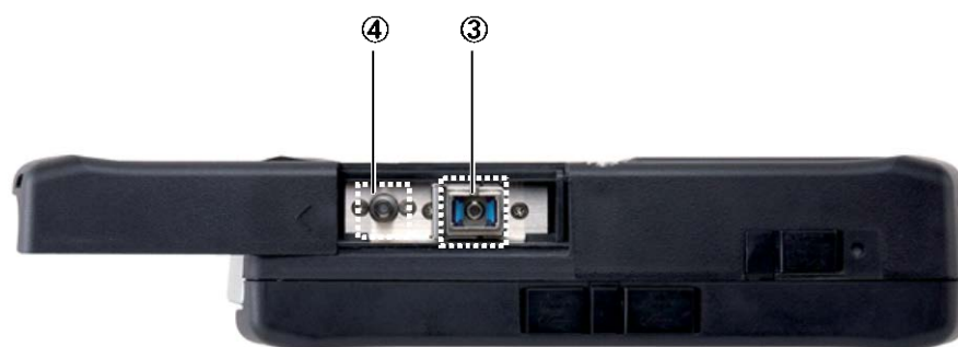
図2.2.2-2 上面 (MU909014A1/B1、MU909015B1)
