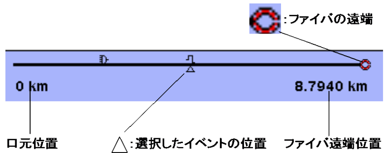
図4.5.1-2 ファイバ模式図
