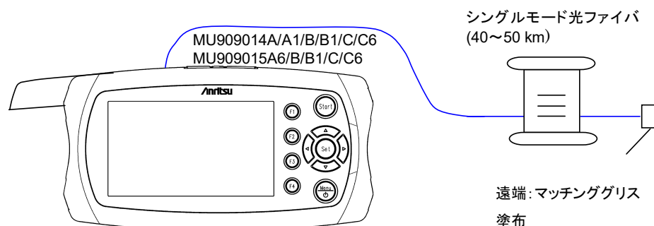
図11.1.6-1 リニアリティ測定の接続図
