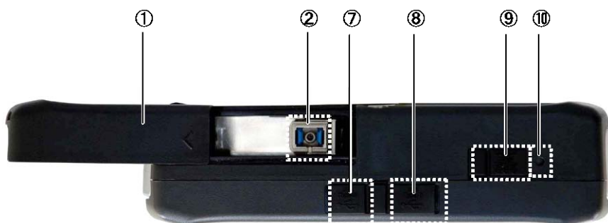
図2.2.2-1 上面 (MU909014A/B、MU909015A6/B、MU909015C-059/069)
