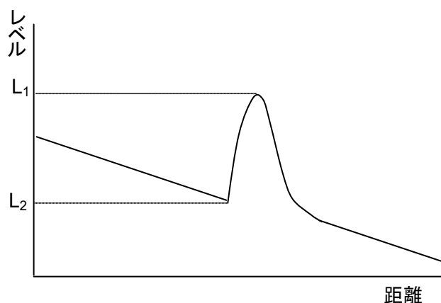
図4.10.2-1 反射減衰量の測定方法
