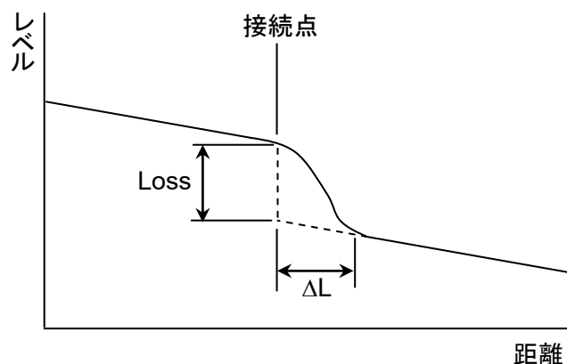
図4.10.1-2 ファイバ接続の測定例
