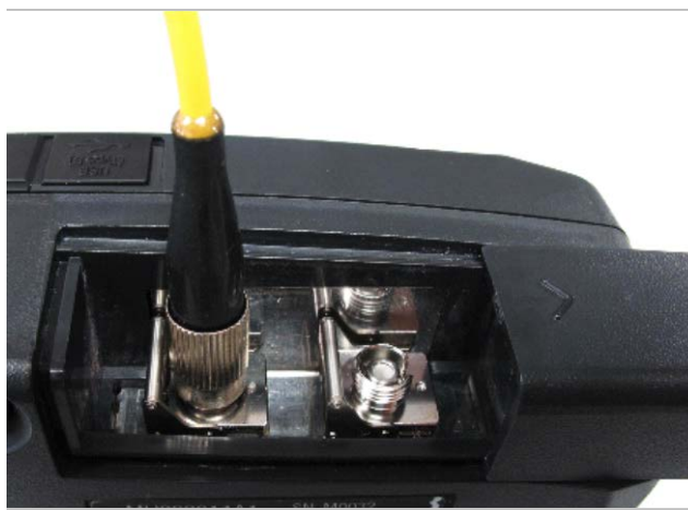
図2.6-1 光ファイバケーブルの接続
