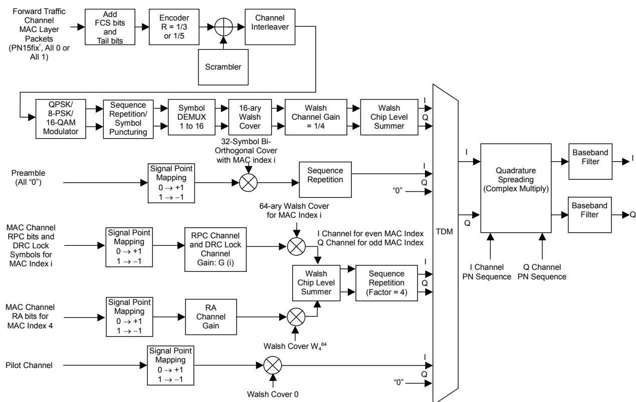
図3.1.5.1-2 1xEV-DO フォワードアクティブスロットのブロックダイアグラム
