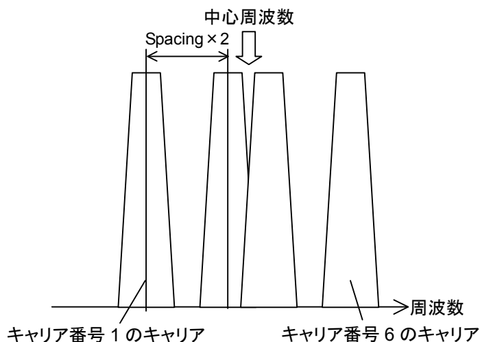
図3.1.5.2-1 マルチキャリアの例
