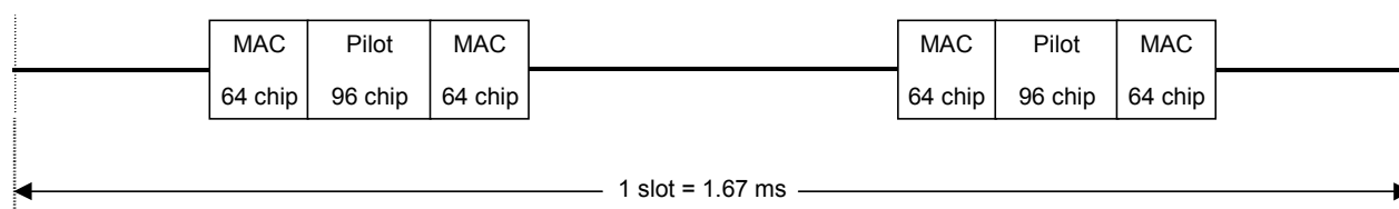
図3.1.5.1-6 時分割多重後の 1xEV-DO フォワードアイドルスロットのスロットフォーマット
