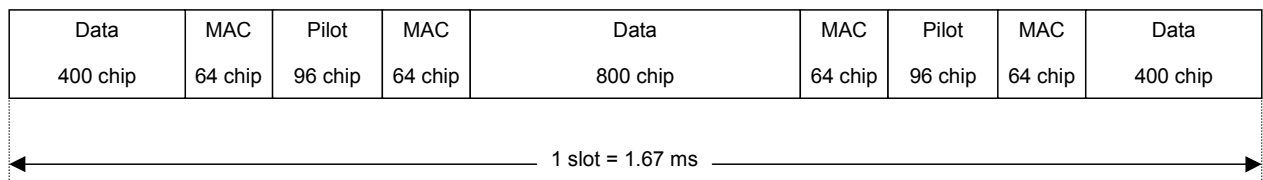
図3.1.5.1-4 時分割多重後の 1xEV-DO フォワードアクティブslotのslotフォーマット
