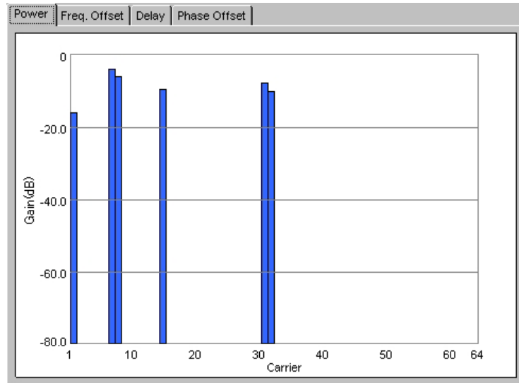
図3.2.1.1-6 Power グラフ
