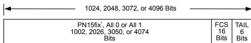
図3.1.5.1-1 フォワードのパケットのフォーマット
