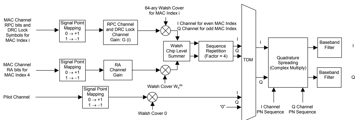
図3.1.5.1-5 1xEV-DO フォワードアイドルスロットのブロックダイアグラム
