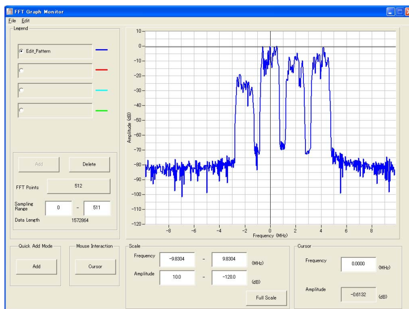
図3.2.4-3 FFT グラフ画面
