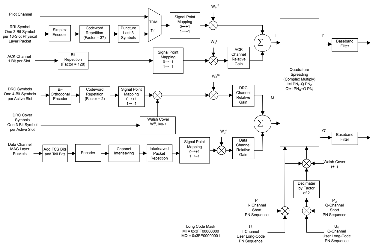
図3.2.5.1-2 1xEV-DO リバースのブロックダイヤグラム
