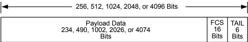
図3.2.5.1-1 リバースのパケットのフォーマット
