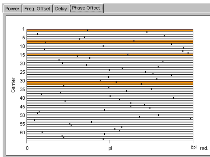
図3.2.1.1-9 Phase Offset グラフ
