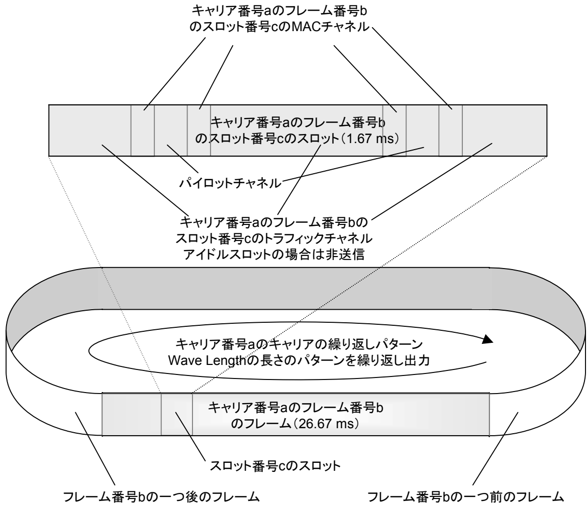
図3.1.5.1-3 1xEV-DO フォワードシングルキャリア波形パターンの繰り返し概念図
