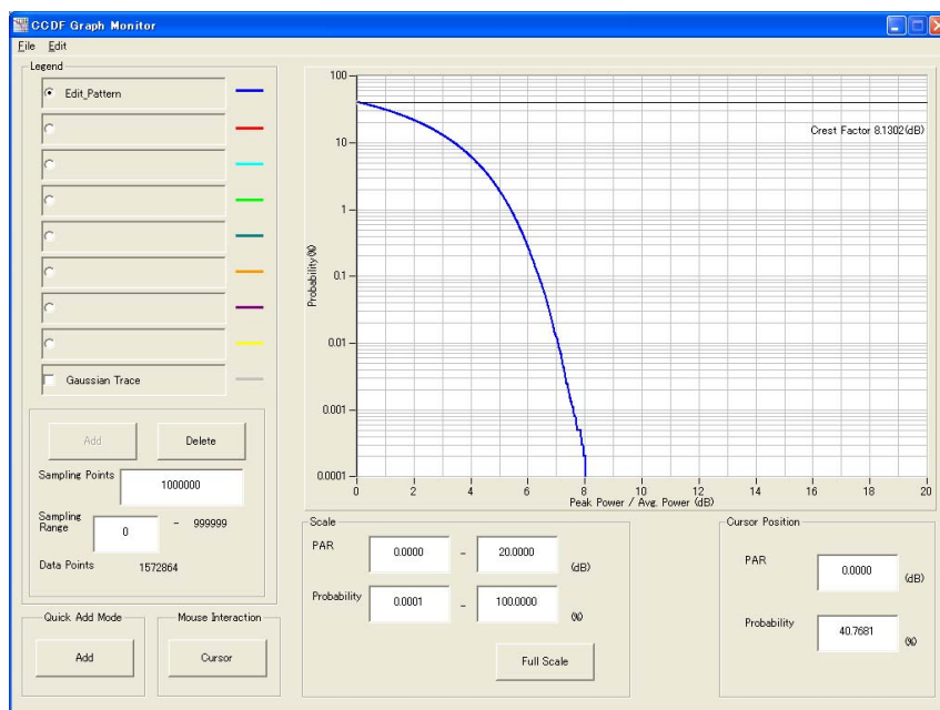
図3.2.4-1 CCDF グラフ画面
