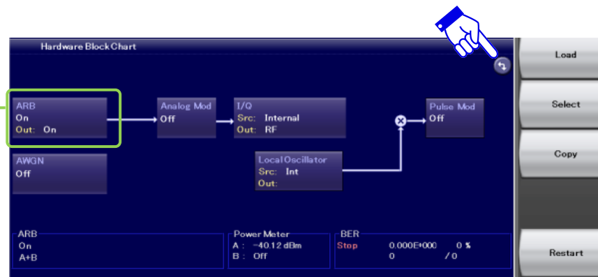
Hardware Block Chart 画面
