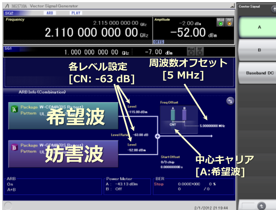
希望波 + 変調妨害波 MG3710Aの設定例
