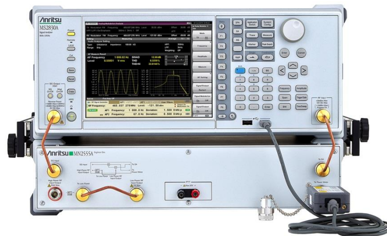
MN2555Aとシグナルアナライザ MS2830A、 USBパワーセンサを接続 (MS2830Aに固定オプションを搭載)
