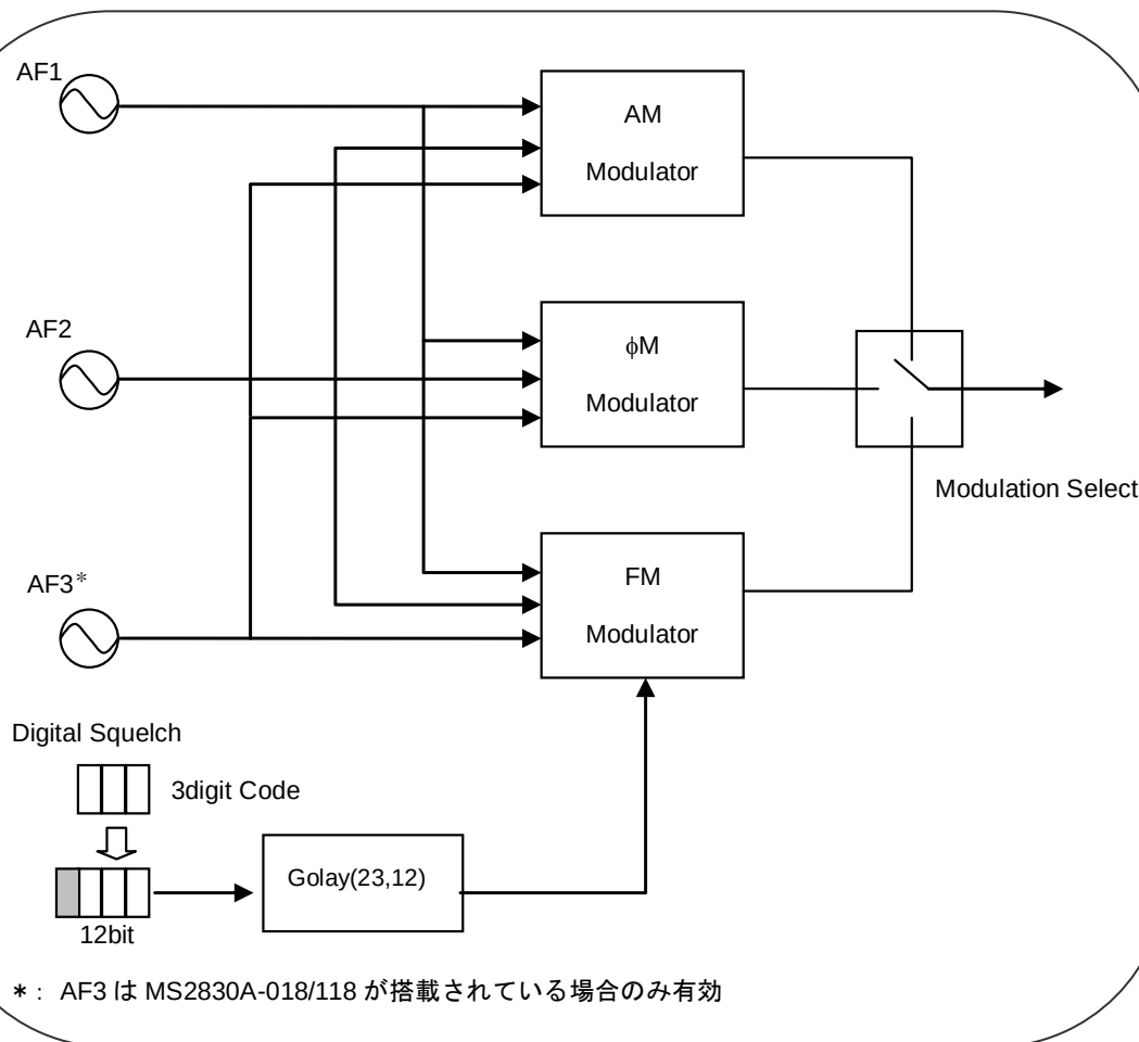
AF信号生成方法の概念図
